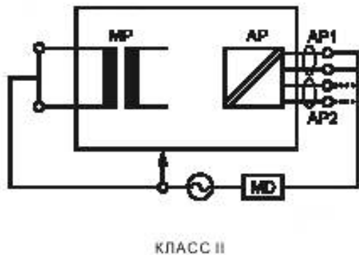
Рисунок 6 — Схема для измерения ТОКА УТЕЧКИ РАБОЧЕЙ ЧАСТИ: РАБОЧАЯ ЧАСТЬ ТИПА F: альтернативный метод
