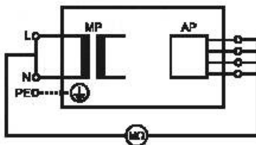
Рисунок 9 — Схема для измерения сопротивления изоляции между СЕТЕВОЙ ЧАСТЬЮ и защитным заземлением для ОБОРУДОВАНИЯ КЛАССА I и (незаземленными) ДОСТУПНЫМИ ПРОВОДЯЩИМИ ЧАСТЯМИ для ОБОРУДОВАНИЯ КЛАССА I и КЛАССА II
