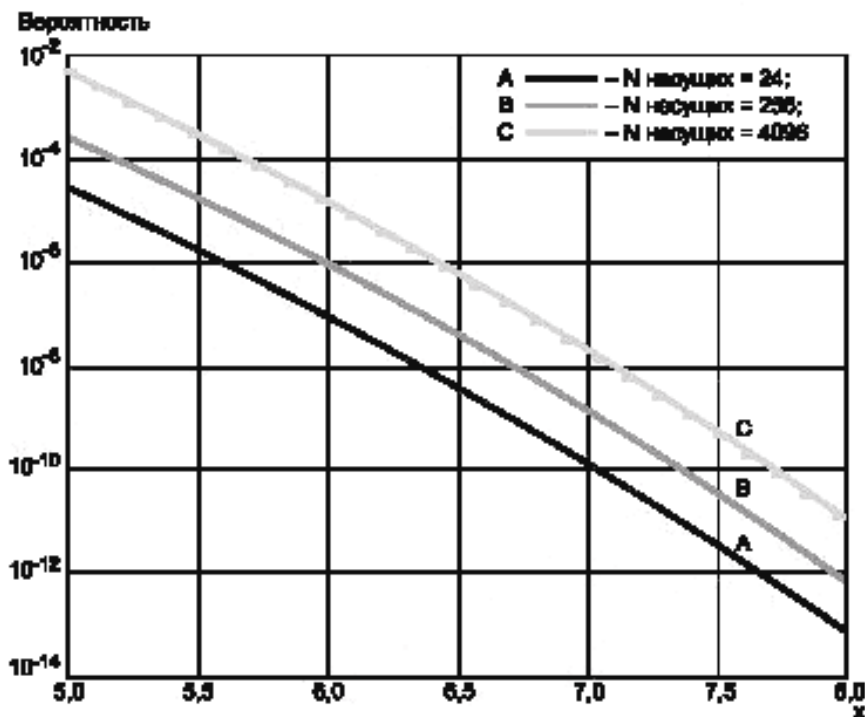
Рисунок A.3 — Вероятность символа с CF > x
