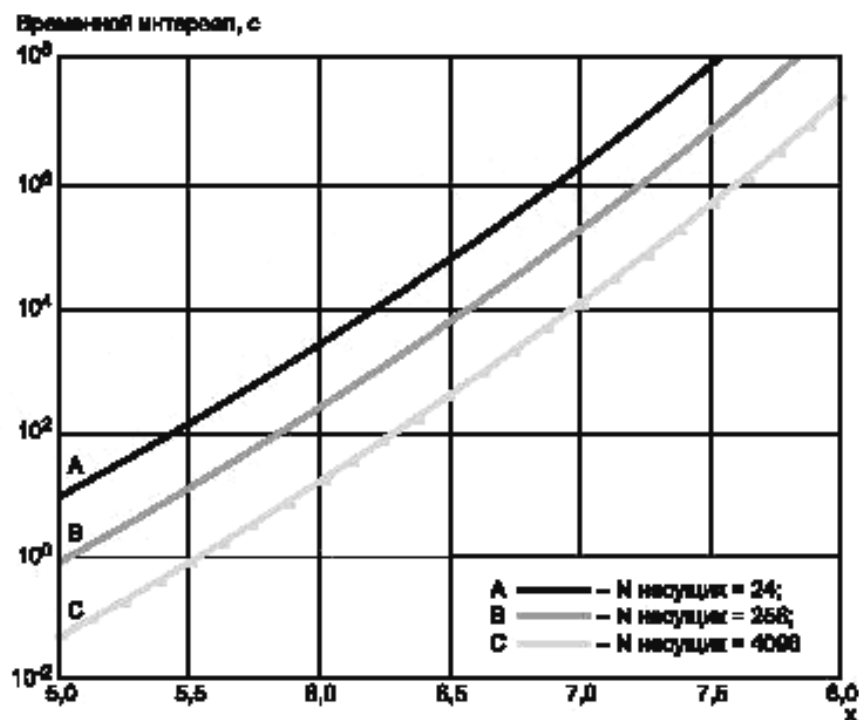
Рисунок А.4 — Интервал между поступлением символа при CF > x (DMT — символ с частотой, равной 4 кГц)
