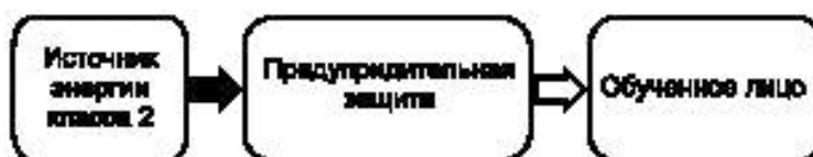
Рисунок 14 — Модель защиты обученного лица от воздействия источника энергии класса 2
