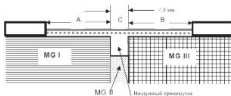
Рисунок O.18 — Компоненты из материалов с разными значениями СИТ, воздушный промежуток между которыми имеет ширину менее X мм
