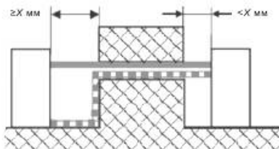
Рисунок O.7 — Нескрепленный стык с широкой канавкой
