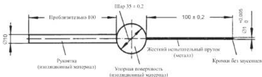
Рисунок V.5 — Щуп для испытания клемм
