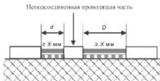
Рисунок O.3 — V-образная канавка
