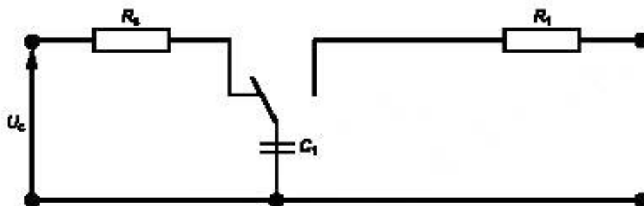
Рисунок D.2 — Испытательный генератор для интерфейса антенны
