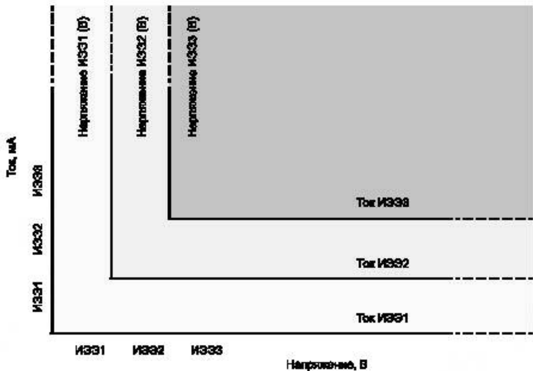
Рисунок 23 — График, демонстрирующий, что предельные значения параметров ИЭЗ зависят и от тока, и от напряжения
