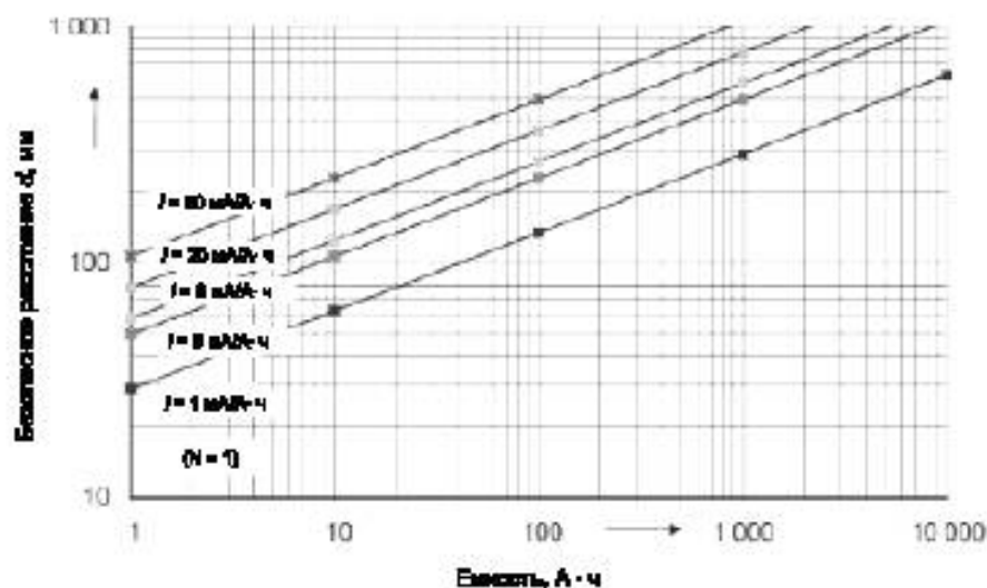
Рисунок М.1 — Зависимость расстояния d от номинальной емкости для различных токов заряда I (мА/А · ч)
