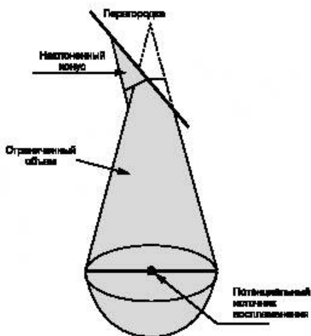
Рисунок 44а — Наклонная перегородка
