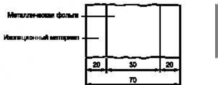
Рисунок 35 — Расположение металлической фольги на изоляционном материале
