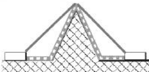
Рисунок O.4 — Промежуточная неподсоединенная проводящая часть
