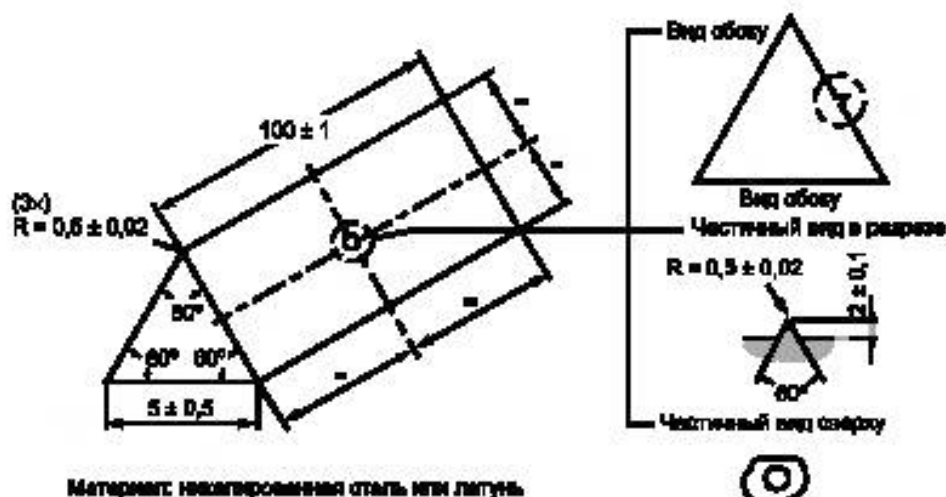
Рисунок 32 — Оправка
