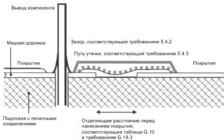
Рисунок O.12 — Покрытие поверх печатного монтажа
