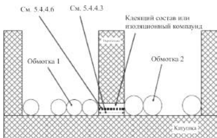
Рисунок O.16 — Секционированная катушка
