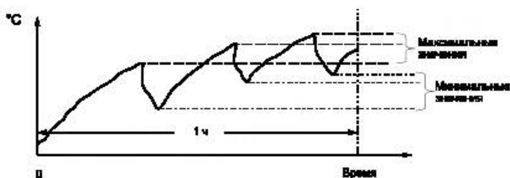
Рисунок G.1 — Определение среднеарифметического значения температуры
