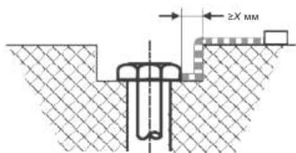
Рисунок O.10 — Большое углубление
