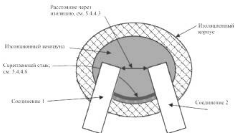
Рисунок O.15 — Устройство, заполненное изоляционным компаундом
