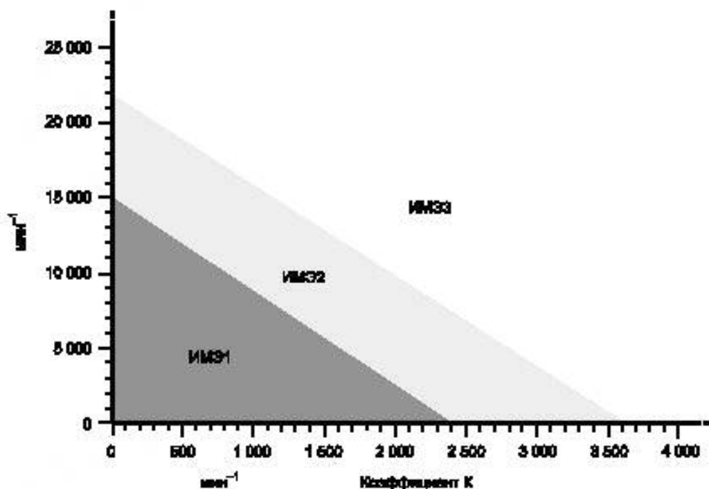
Рисунок 47 — График, на котором показаны предельные значения параметров ИМЭ для вращающихся лопастей вентиляторов
