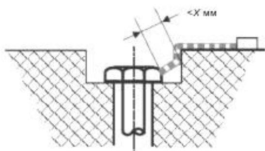
Рисунок O.9 — Малое углубление
