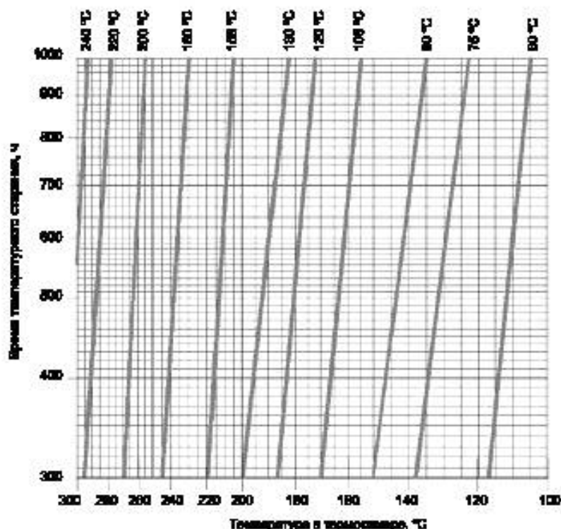
Рисунок G.2 — Время теплового старения
