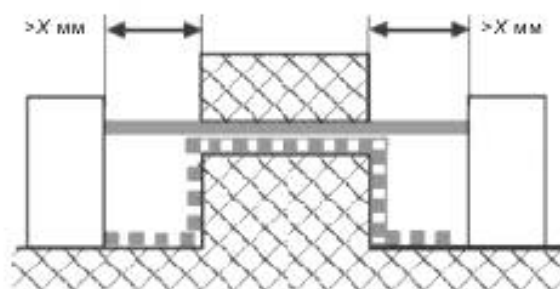
Рисунок O.6 — Нескрепленный стык с узкой канавкой
