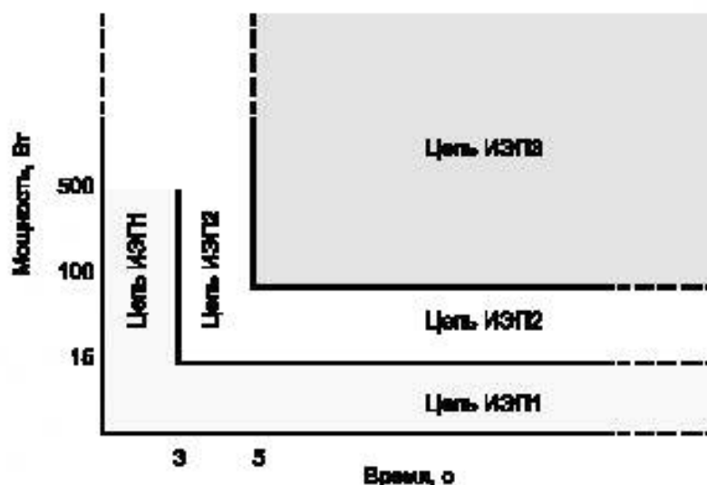
Рисунок 40 — Классификация источников электропитания
