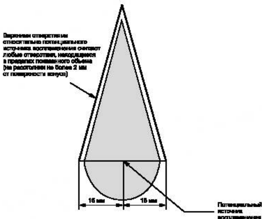
Рисунок 45 — Верхние отверстия
