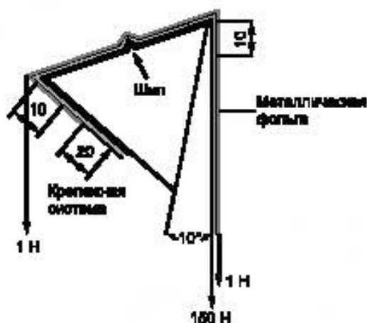
Рисунок 34 — Конечное положение оправки
