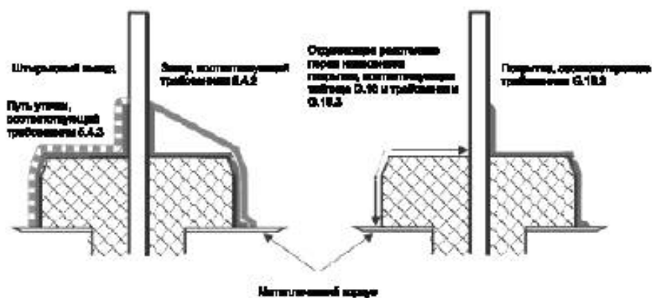
Рисунок O.11 — Покрытие выводов
