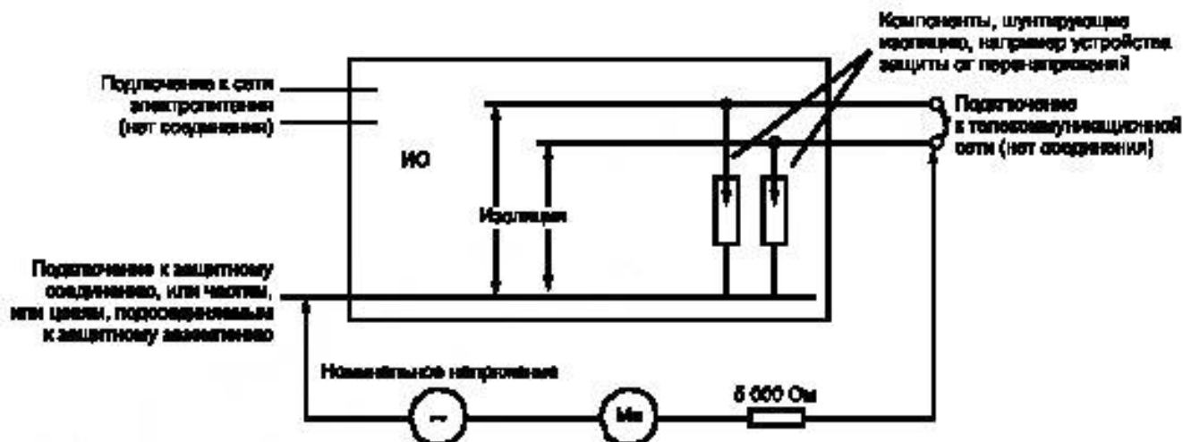
Рисунок 37 — Испытание разделения между телекоммуникационной сетью и землей
