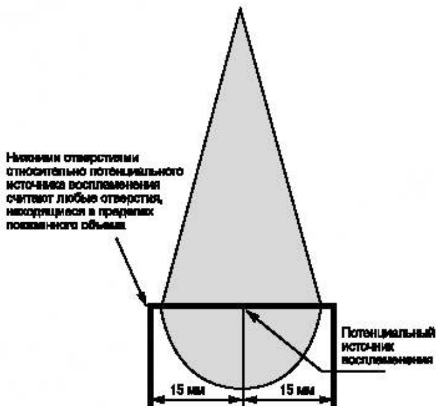
Рисунок 46 — Нижние отверстия
