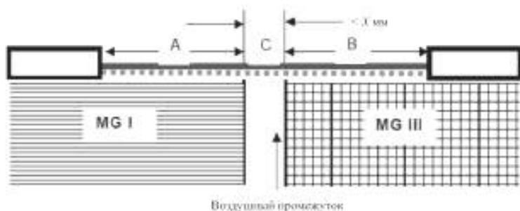
Рисунок O.17 — Материалы с разными значениями СИТ
