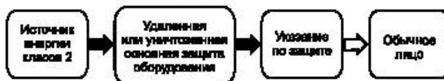
Рисунок 11 — Модель защиты обычного лица от воздействия источника энергии класса 2 в процессе эксплуатации оборудования
