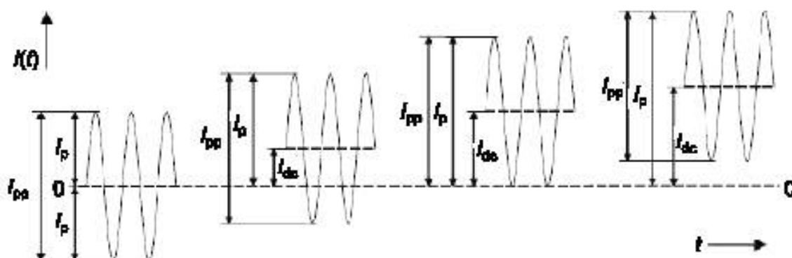
Рисунок Н.3 — Пиковое значение тока и удвоенная амплитуда тока
