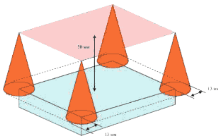
Рисунок 17 — Использование конуса пламени в случае крупного компонента
