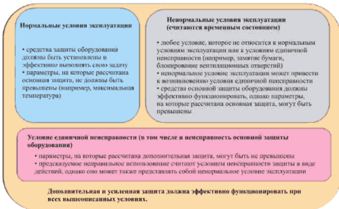
Рисунок 25 — Обзор режимов работы
