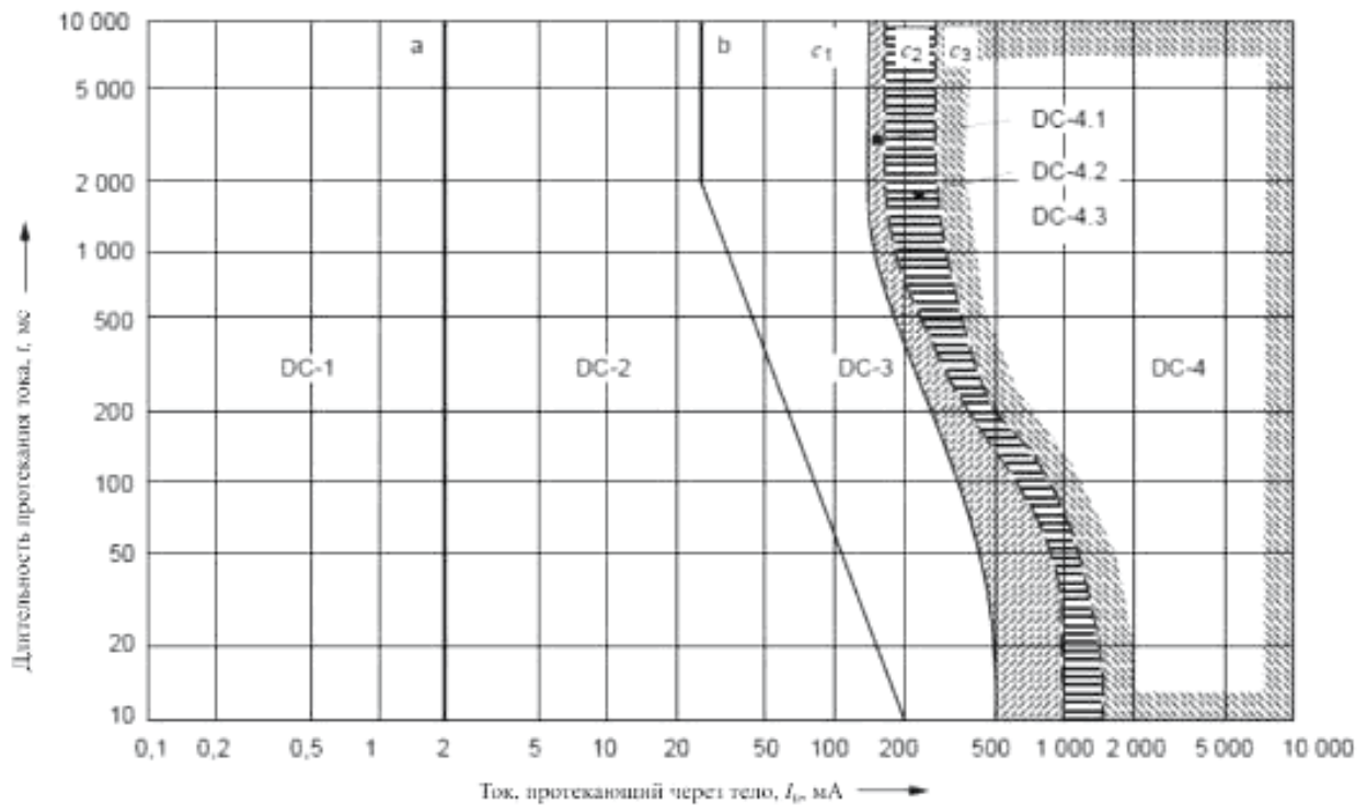
Рисунок 2— Условные зоны на графике «время/ток», описывающие воздействие постоянного тока на человека для пути протекания тока снизу вверх (IEC/TS 60479-1:2005, рисунок 22)
