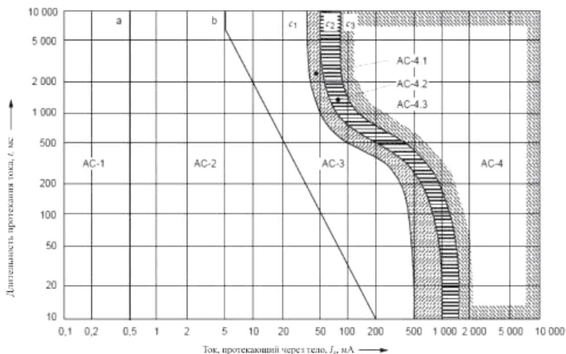
Рисунок 1— Условные зоны на графике «время/ток», описывающие воздействие переменного тока (15–100 Гц) на человека для пути протекания тока «левая рука – ноги» (IEC/TS 60479-1:2005, рисунок 20)
