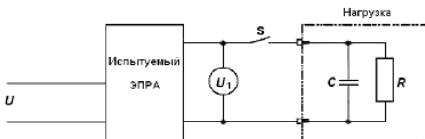
Рисунок А.1б — Испытательная схема измерения тока при соединении ЭПРА с нагрузкой после достижения установившегося режима работы
