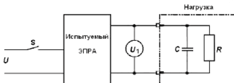
Рисунок А.1а — Испытательная схема измерения тока при включении ЭПРА в сеть
