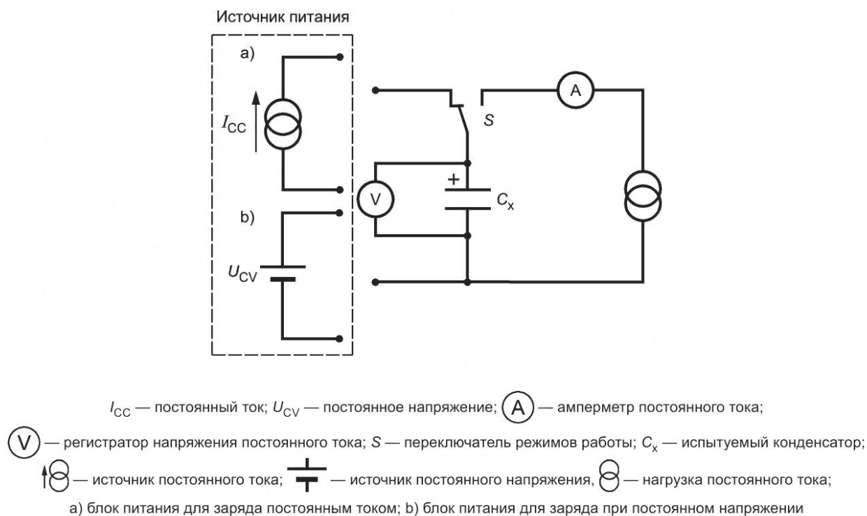
Рисунок 1 — Принципиальная электрическая схема измерения емкости и внутреннего сопротивления
