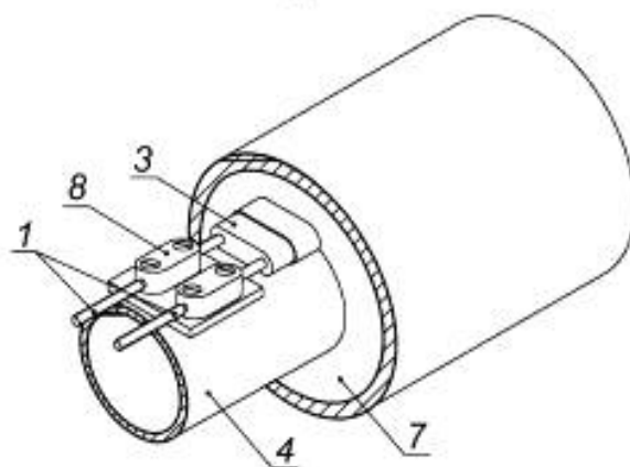
Деталь А
