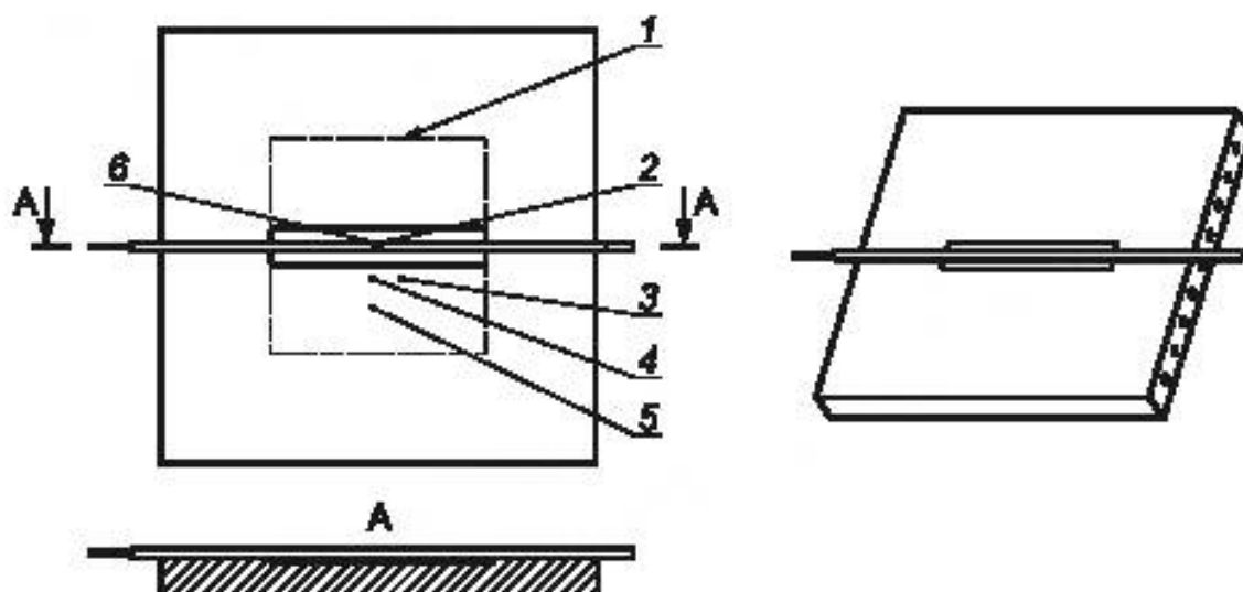
Рисунок 8 — Испытательный трубопровод
