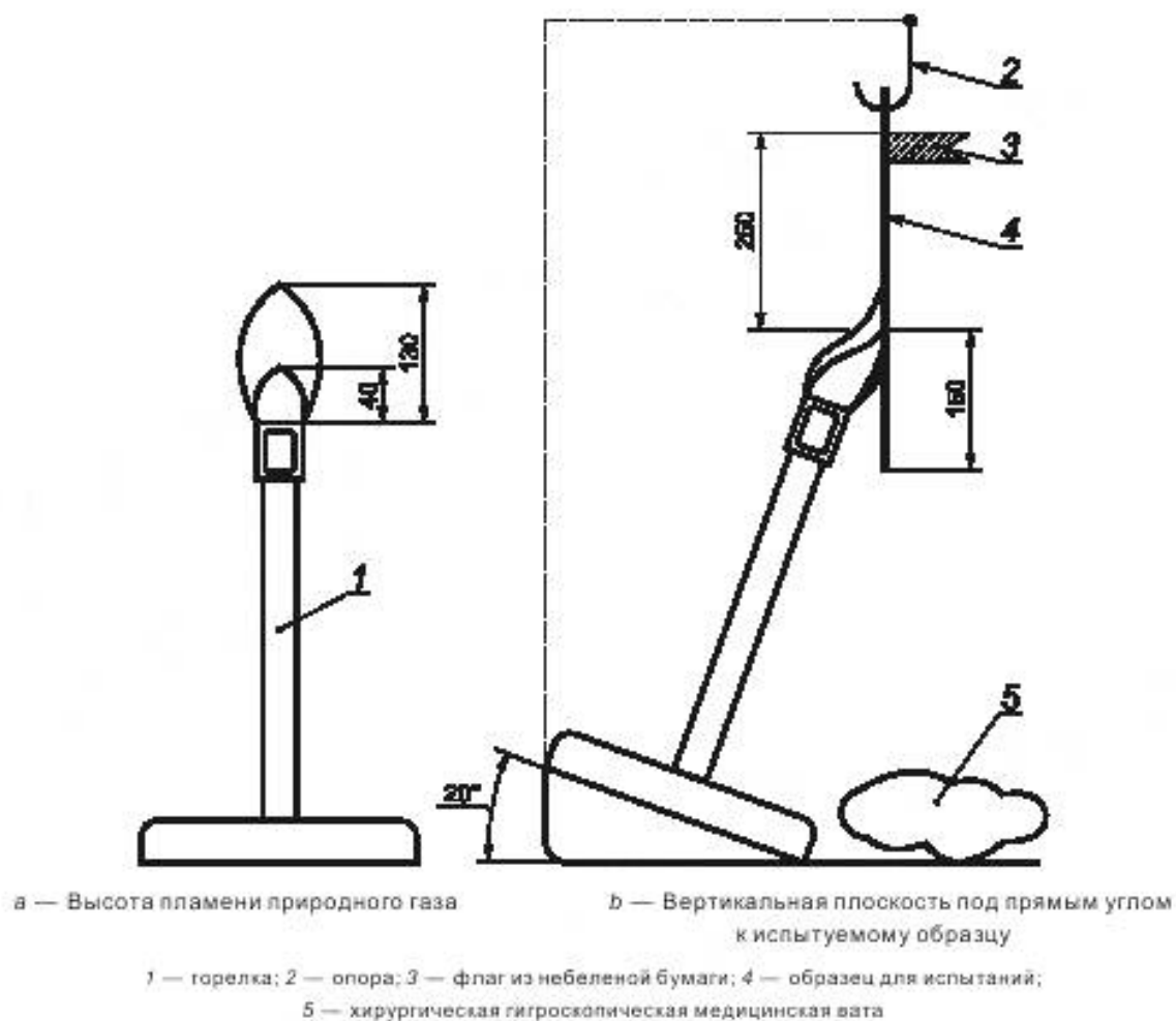
Рисунок 1 — Испытание на воспламеняемость
