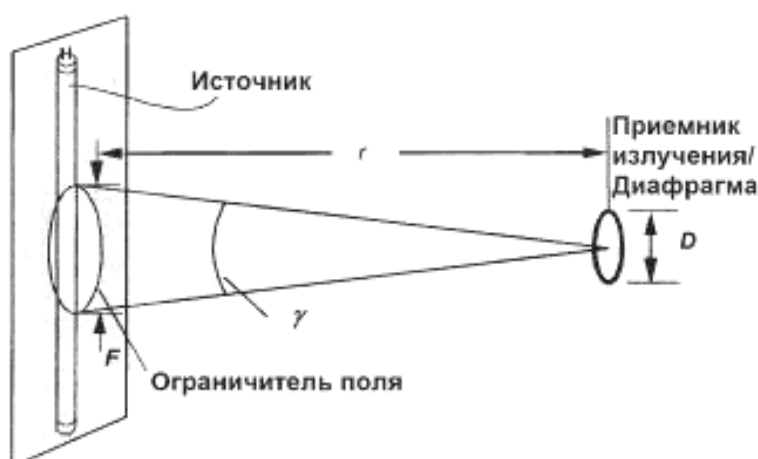
Рисунок 5.3 – Альтернативная схема измерений энергетической яркости
