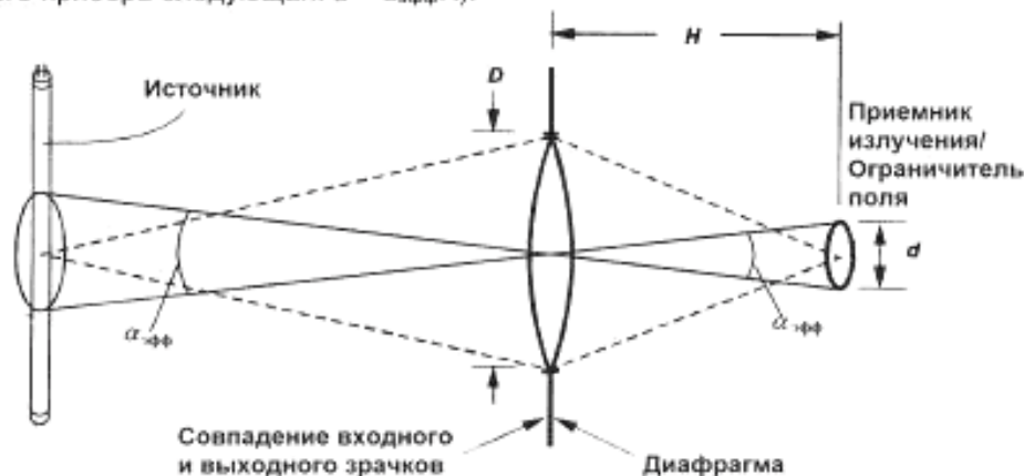
Рисунок 5.2 – Пример изображения прибора для измерений энергетической яркости
