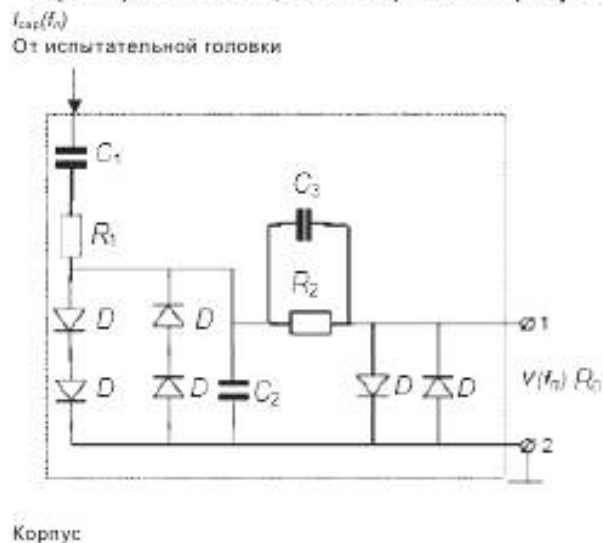
Рисунок 2 – Пример схемы защиты
