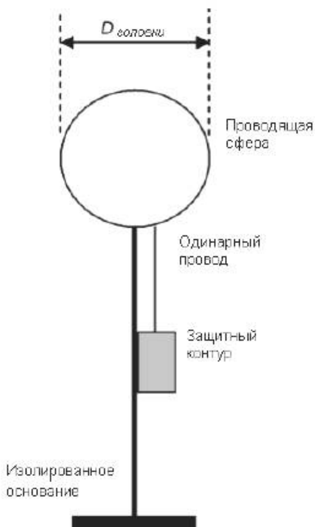
Рисунок 1– Испытательная головка «Ван-дер-Хуфдена»
