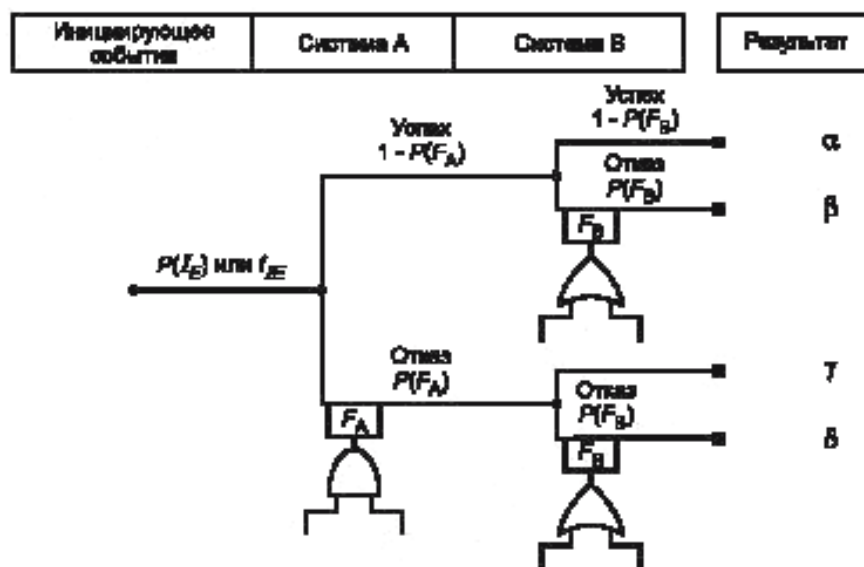
Рисунок 6 — Соединение с деревом неисправностей
