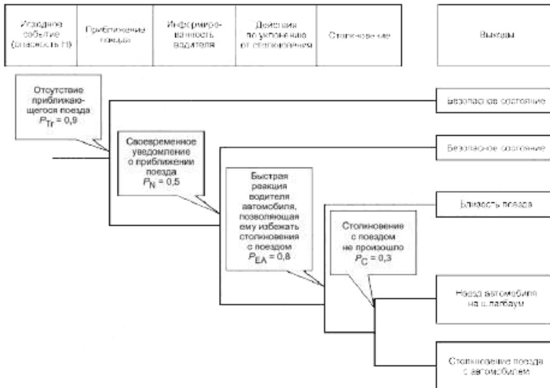
Рисунок В.4 — ETA для железнодорожного переезда
