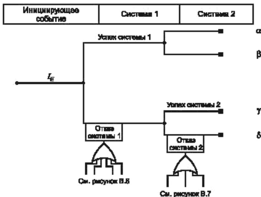
Рисунок В.5 — Простой пример
