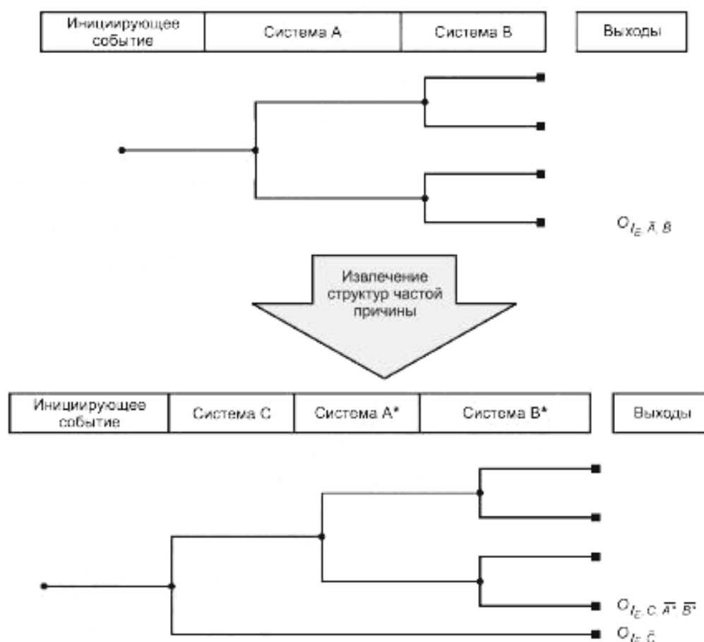
Рисунок 4 — Моделирование структурных или физических зависимостей
