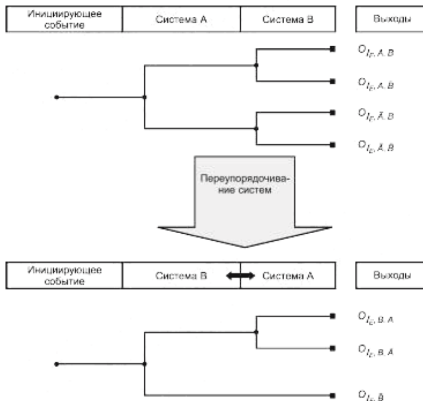
Рисунок 3 — Функциональные зависимости дерева событий
