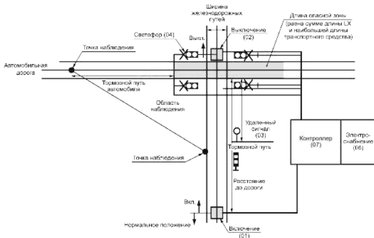
Рисунок В.3 — Система железнодорожного переезда (LX)
