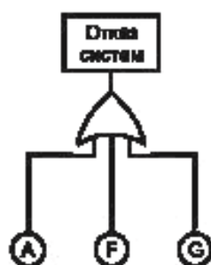
Рисунок В.7 — Дерево неисправностей для системы 2
