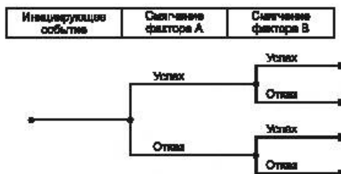
Рисунок 2 — Основное графическое представление дерева событий
