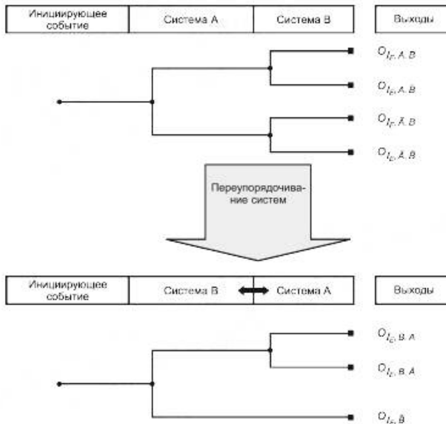
Рисунок 3 — Функциональные зависимости дерева событий
