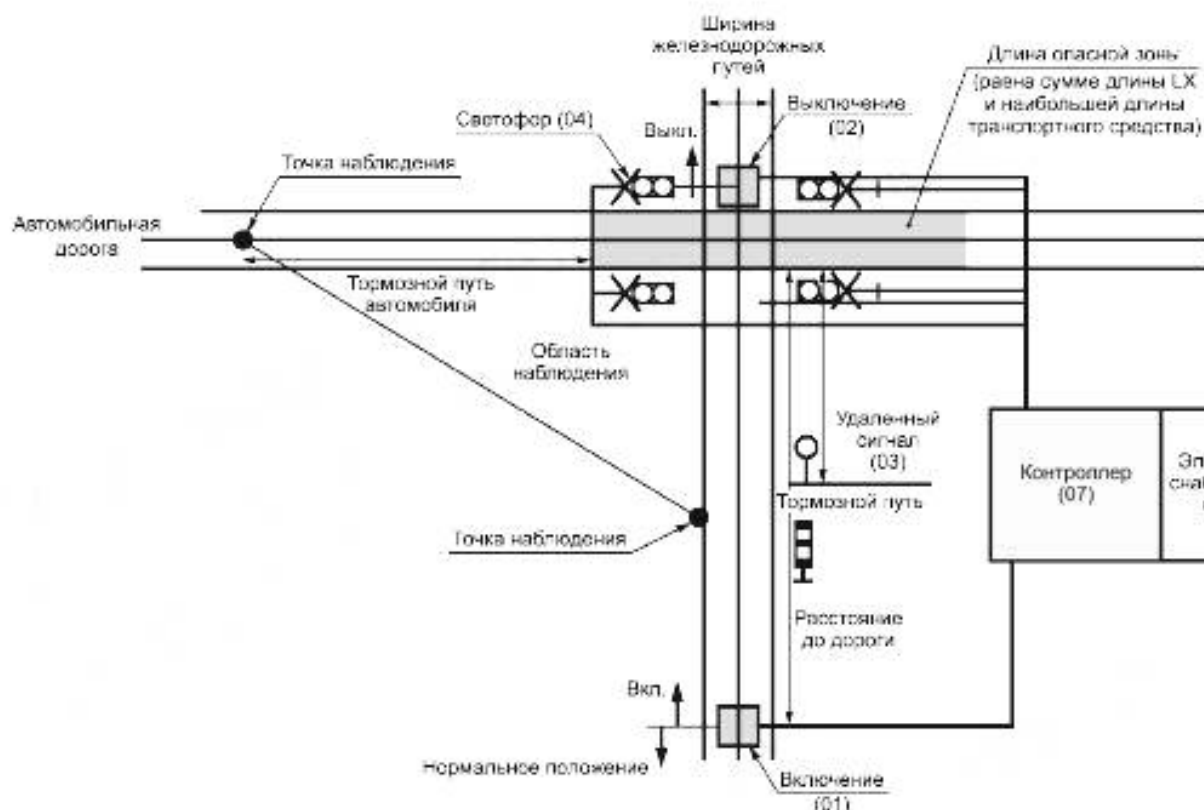
Рисунок В.3 — Система железнодорожного переезда (LX)
