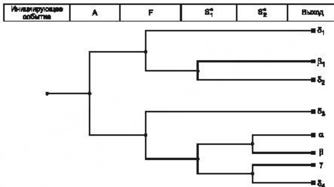
Рисунок В.8 — Модифицированное дерево событий
