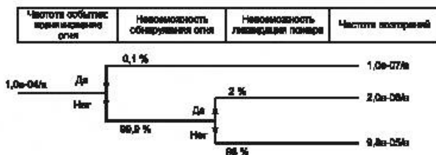
Рисунок В.2 — Дерево событий для пожара
