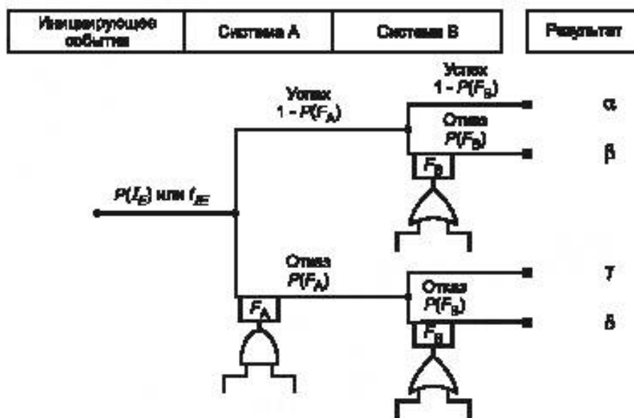
Рисунок 6 — Соединение с деревом неисправностей
