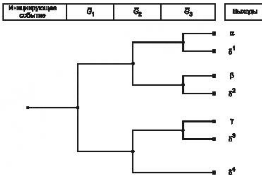
Рисунок В.9 — Дерево событий после «группировки отказов»
