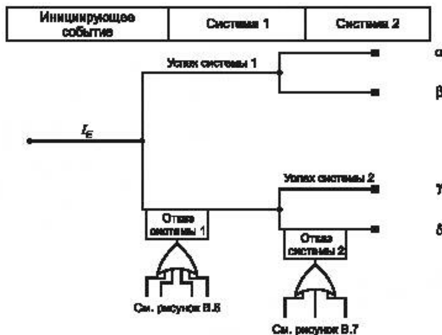
Рисунок В.5 — Простой пример
