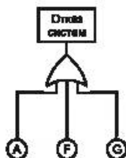
Рисунок В.7 — Дерево неисправностей для системы 2
