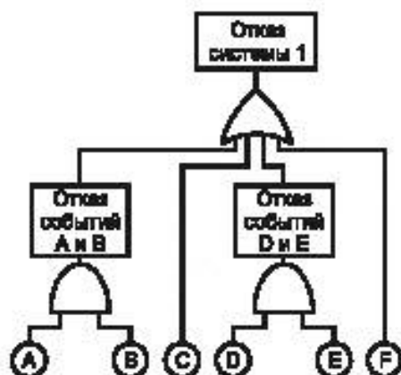
Рисунок В.6 — Дерево неисправностей для системы 1
