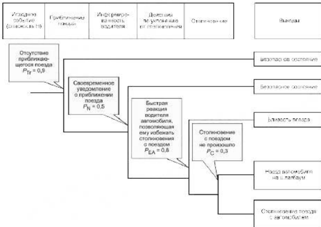
Рисунок В.4 — ETA для железнодорожного переезда
