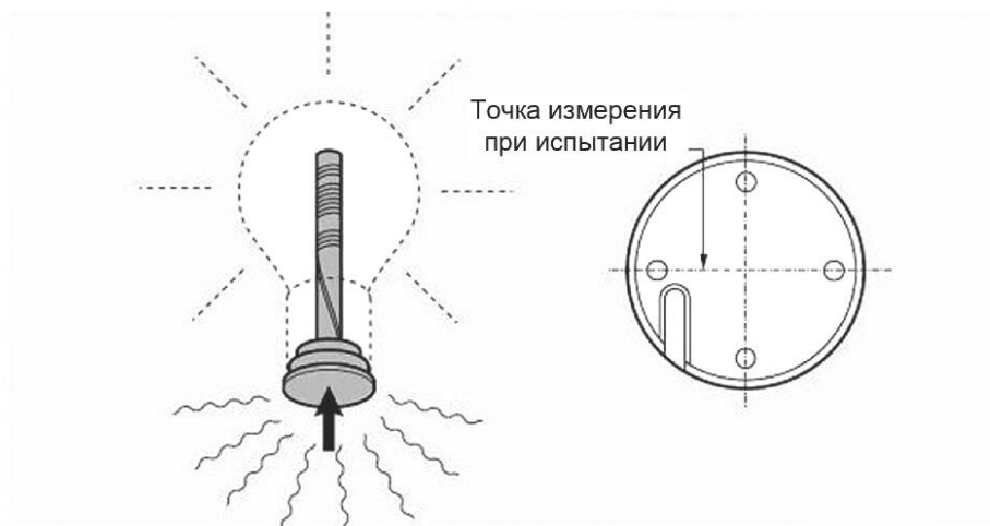
Рисунок F.1 — Точка измерения температуры при испытании высокочастотной газоразрядной лампы с внутренним соединением (рабочая частота 2500—3000 кГц)
