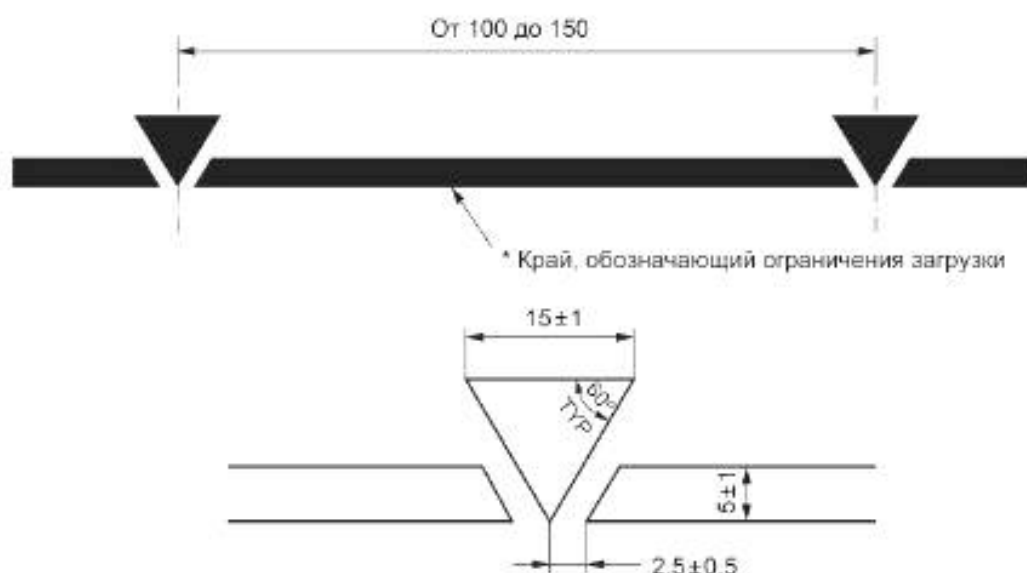
Рисунок 4 — Маркировка ограничения загрузки
