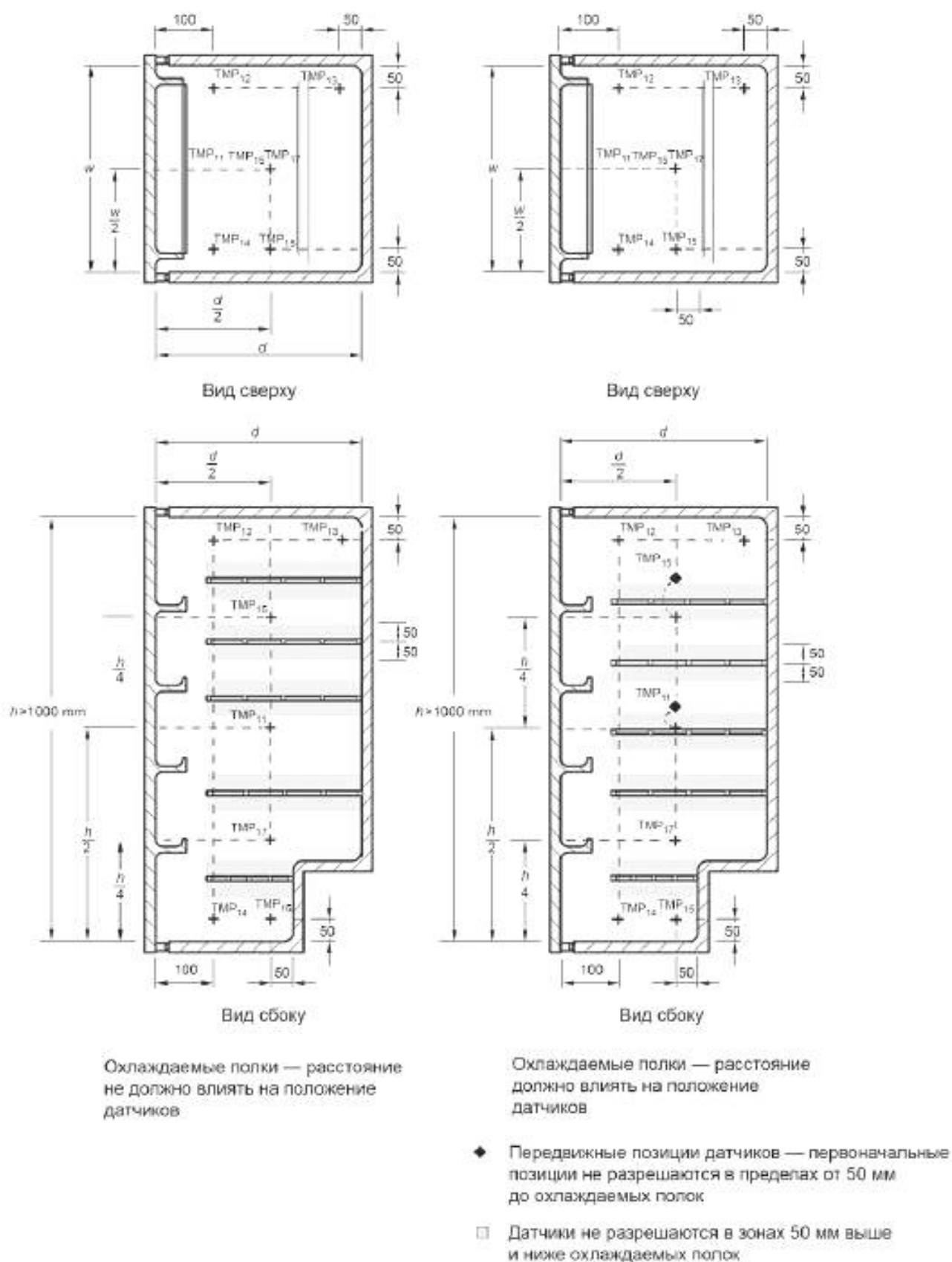
Рисунок D.6 — Расположение датчиков температуры внутри вертикального низкотемпературного отделения с охлаждаемыми полками и с высотой больше 1000 мм
