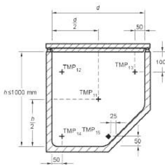
Вид сбоку d) Тип 4
