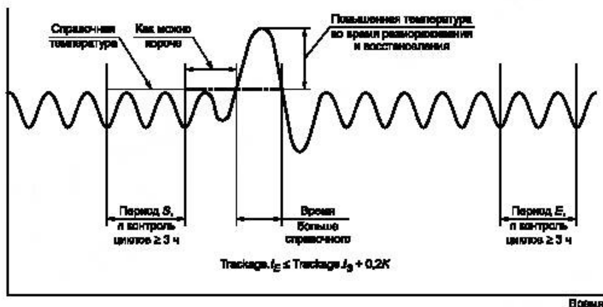
Рисунок 3 — Последовательность испытаний хранения
