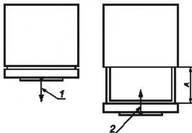
A — ход выдвижения; 1 — выдвижение; 2 — задвигание
