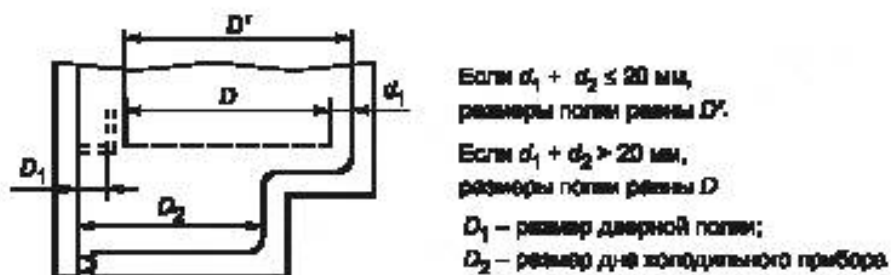
с) Определение глубины дверной полки прибора типа «шкаф»
