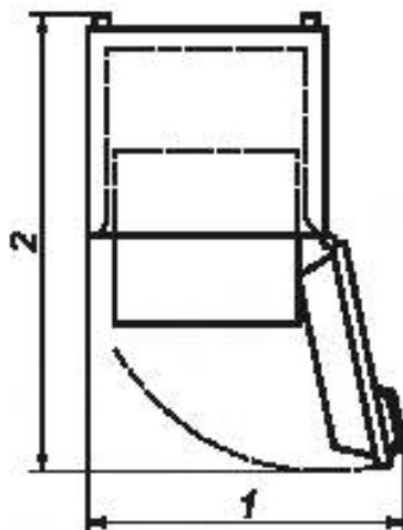
1 — ширина; 2 — глубина при открытой двери
