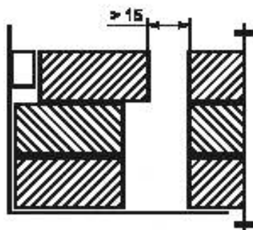
Рисунок 8 — Размещение стопок пакетов, уложенных со смещением
