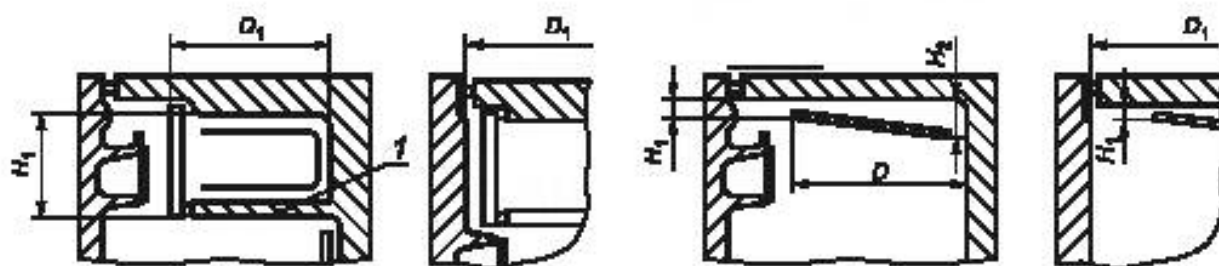
Перегородка, рассматриваемая как нераздельная часть
