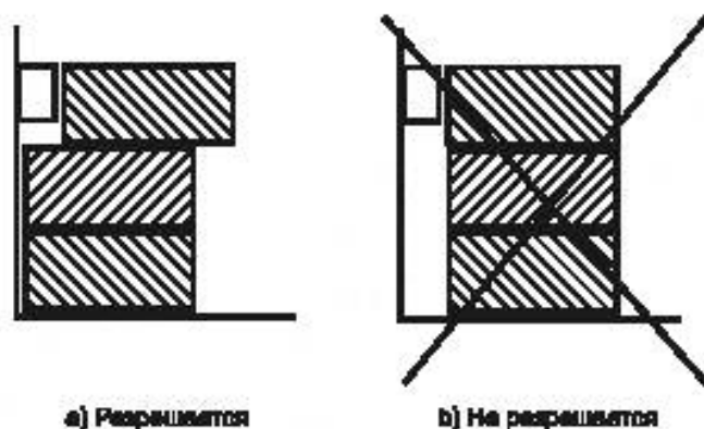
Рисунок 7 — Стопка пакетов, уложенных со смещением
