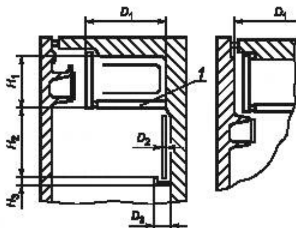
Перегородка, рассматриваемая как отдельная часть
