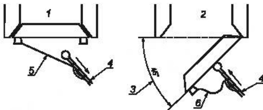
1 — открывание двери; 2 — закрывание двери; 3 — угол открывания; 4 — толкатель; 5 — трос в натянутом состоянии; 6 — трос без натяжения
