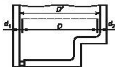
b) Определение глубины полки
