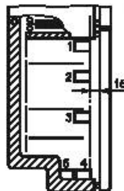
Вид сбоку (в разрезе)
