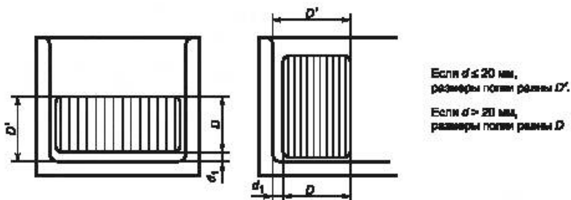
е) Определение ширины и глубины полуполок
