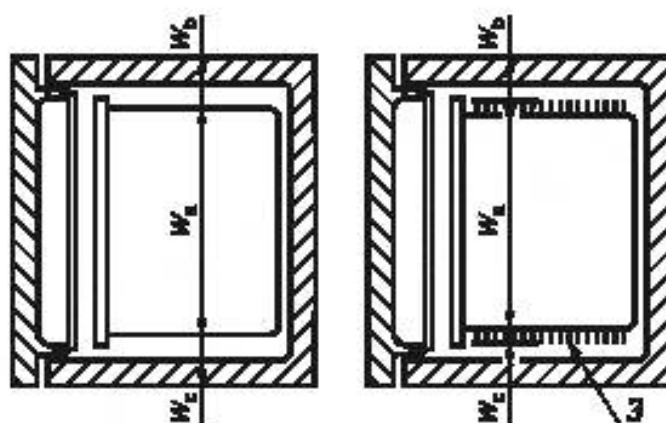
Определение ширины (вид сверху)
