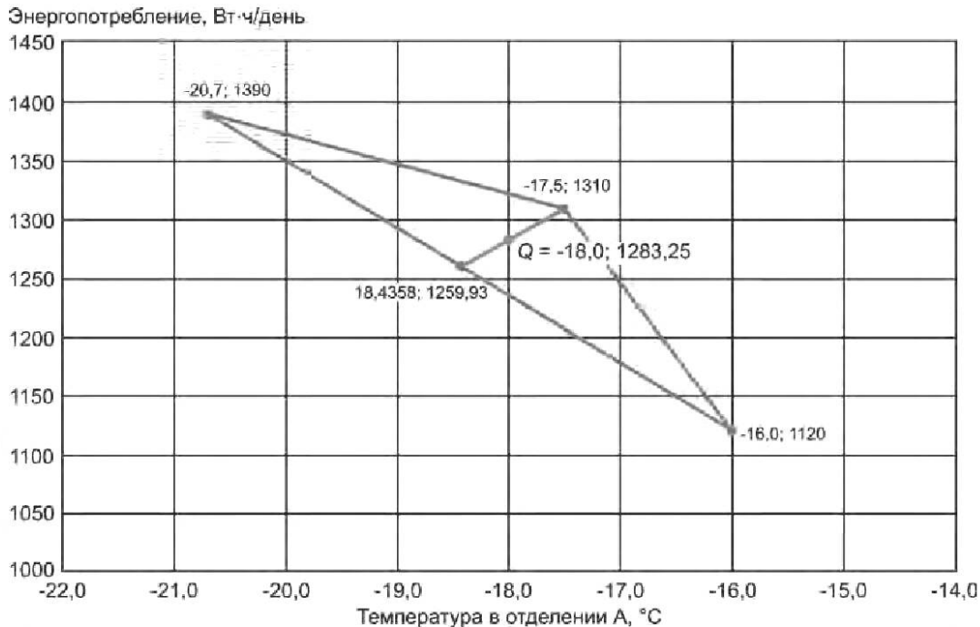
Рисунок I.9 — Пример триангуляции (температура и энергопотребление)
