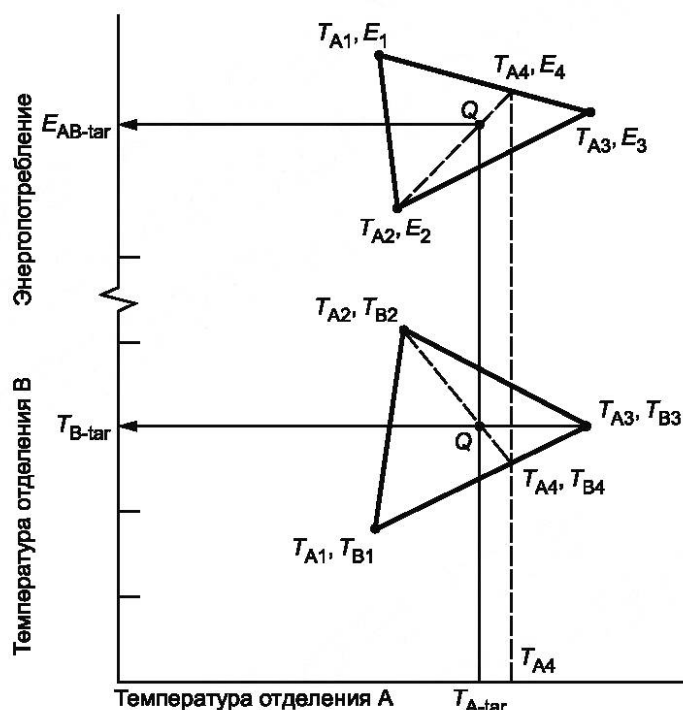
Рисунок Е.4 — Схематическое представление интерполяции посредством триангуляции
