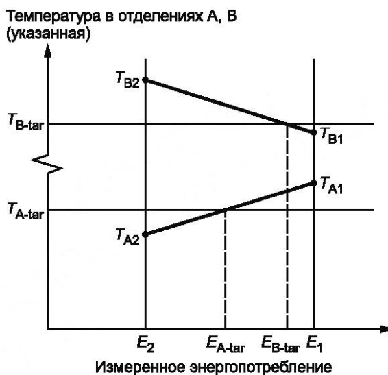
Рисунок Е.3 — Интерполяция без корректных результатов
