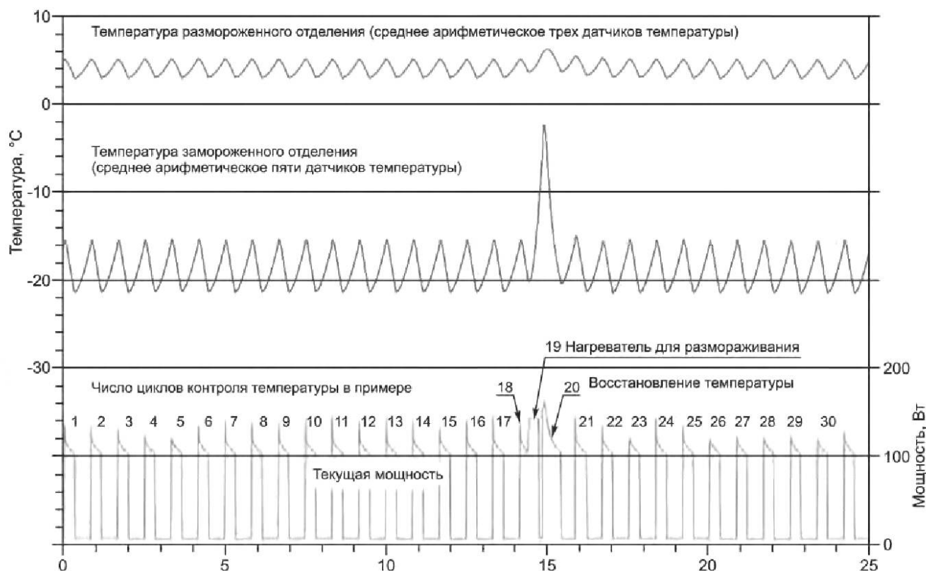
Рисунок I.10 — Пример данных по мощности и температуре
