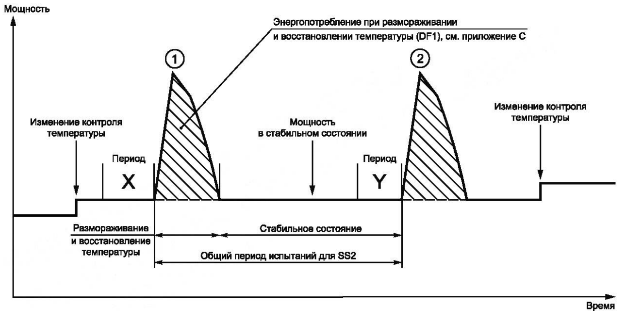
Рисунок В.3 — Подход SS2 — типичная модель работы холодильного прибора с циклом управления размораживанием
