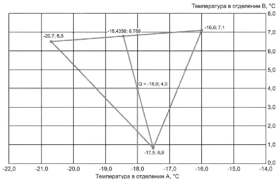
Рисунок 1.8 — Пример триангуляции (температуры)
