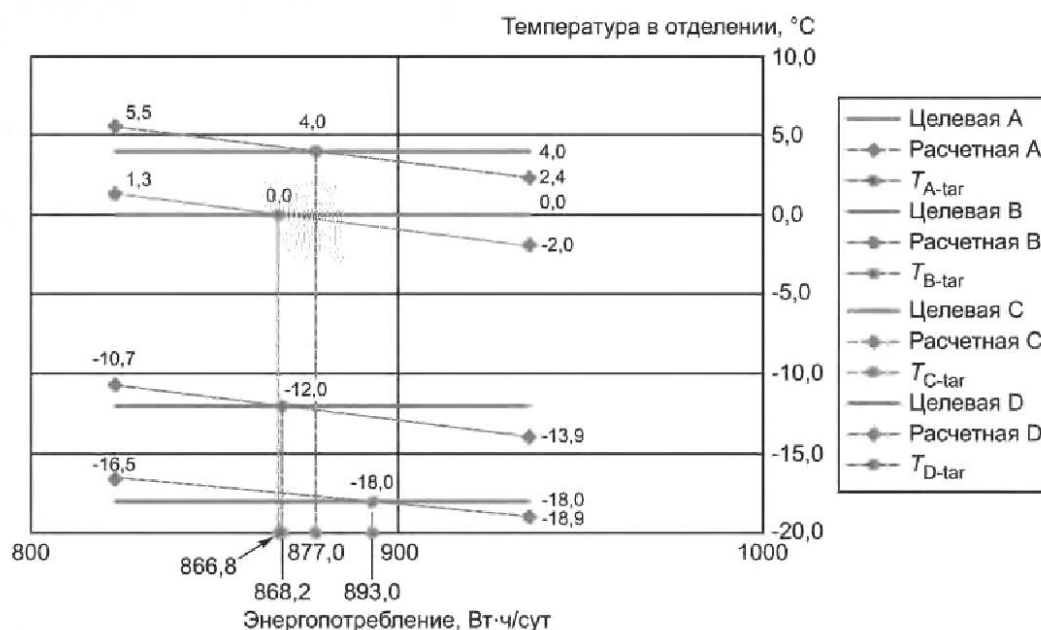
Рисунок I.7 — Пример интерполяции для 4 отделений
