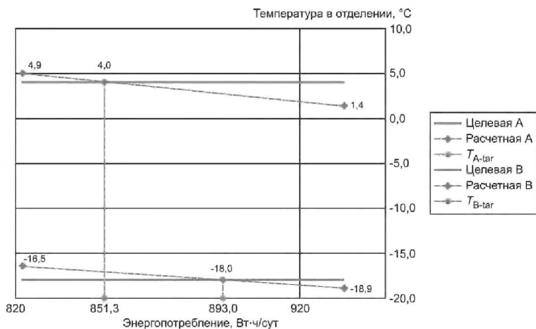
Рисунок I.2 — Пример линейной интерполяции для двух отделений (отделение В критическое)
