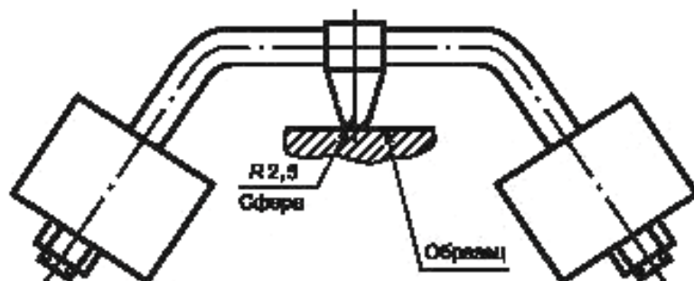
Рисунок 5 — Устройство для вдавливания шарика (по МЭК 60598-1, рисунок 10)
