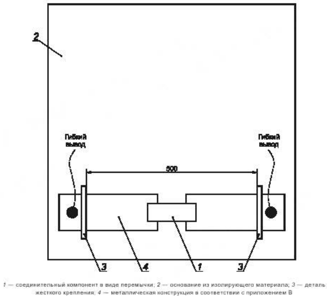
Рисунок 3 — Пример соединения перемычкой
