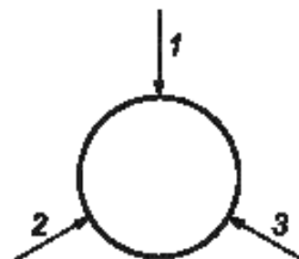
Рисунок 1 — Пример измерения толщины покрытия по окружности стержня
