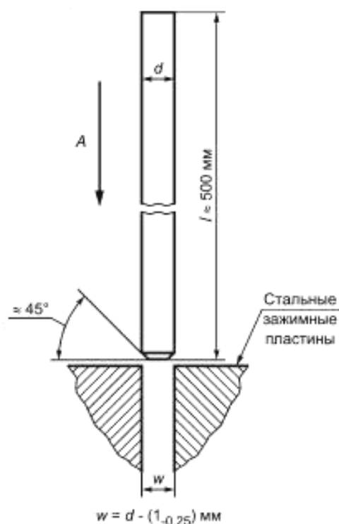
Рисунок 2 — Пример испытания адгезии
