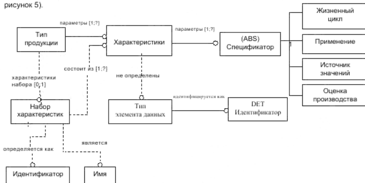
Рисунок 5 – Включение наборов характеристик
