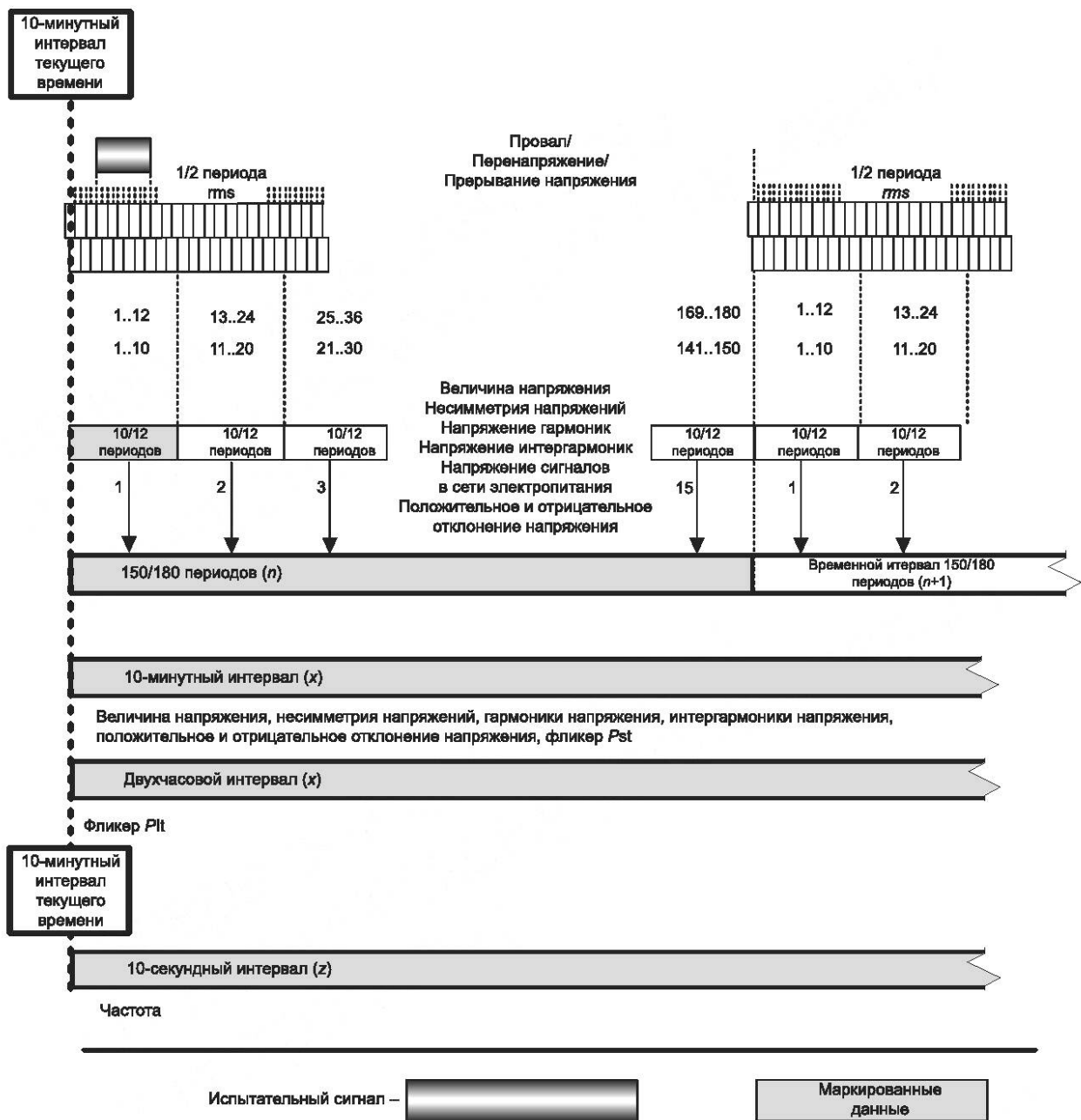
Рисунок 16 — Испытание маркирования для измерительных приборов класса А
