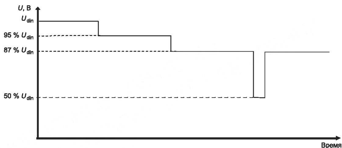
Рисунок 38 — Испытание скользящего опорного напряжения сравнения
