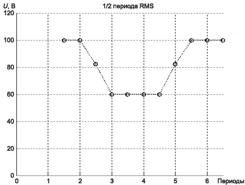
Рисунок 6 — Вторая детализация формы сигнала при испытании на провалы напряжения в соответствии с испытанием A4.1.2
