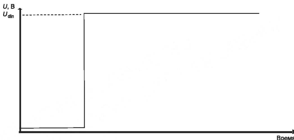
Рисунок 10 — Порог срабатывания при испытаниях скользящего опорного напряжения сравнения
