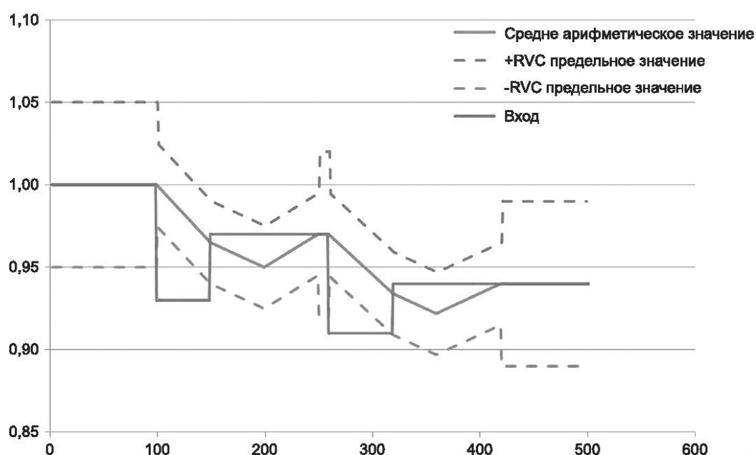
Рисунок 33 — Форма сигнала вместе с RVC-предельными значениями и средним арифметическим значением по A13.5.2
