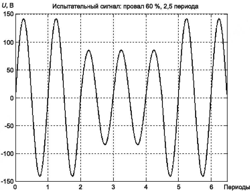
Рисунок 34 — Первая детализация формы сигнала при испытании на провалы напряжения в соответствии с испытанием S4.1.2
