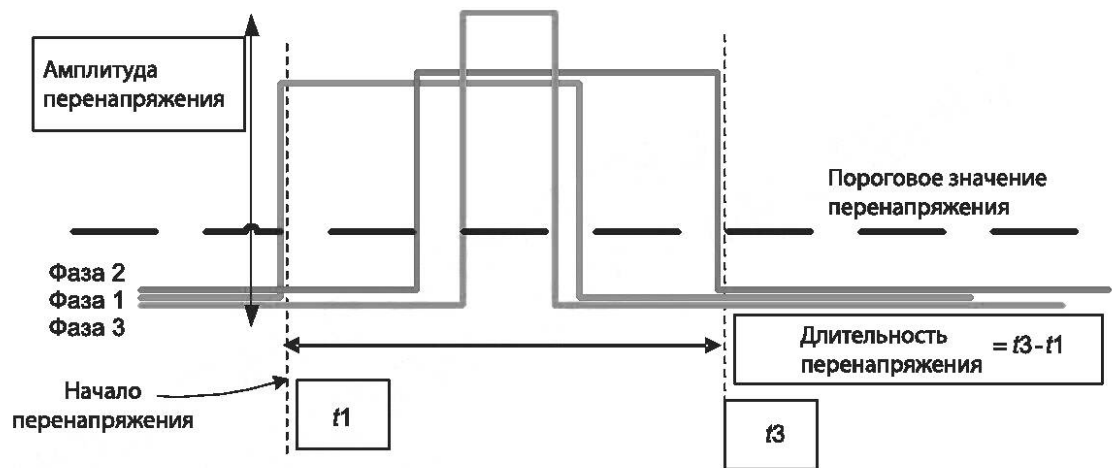
Рисунок 14 — Первая детализация формы волны при испытаниях на перенапряжения в многофазной системе
