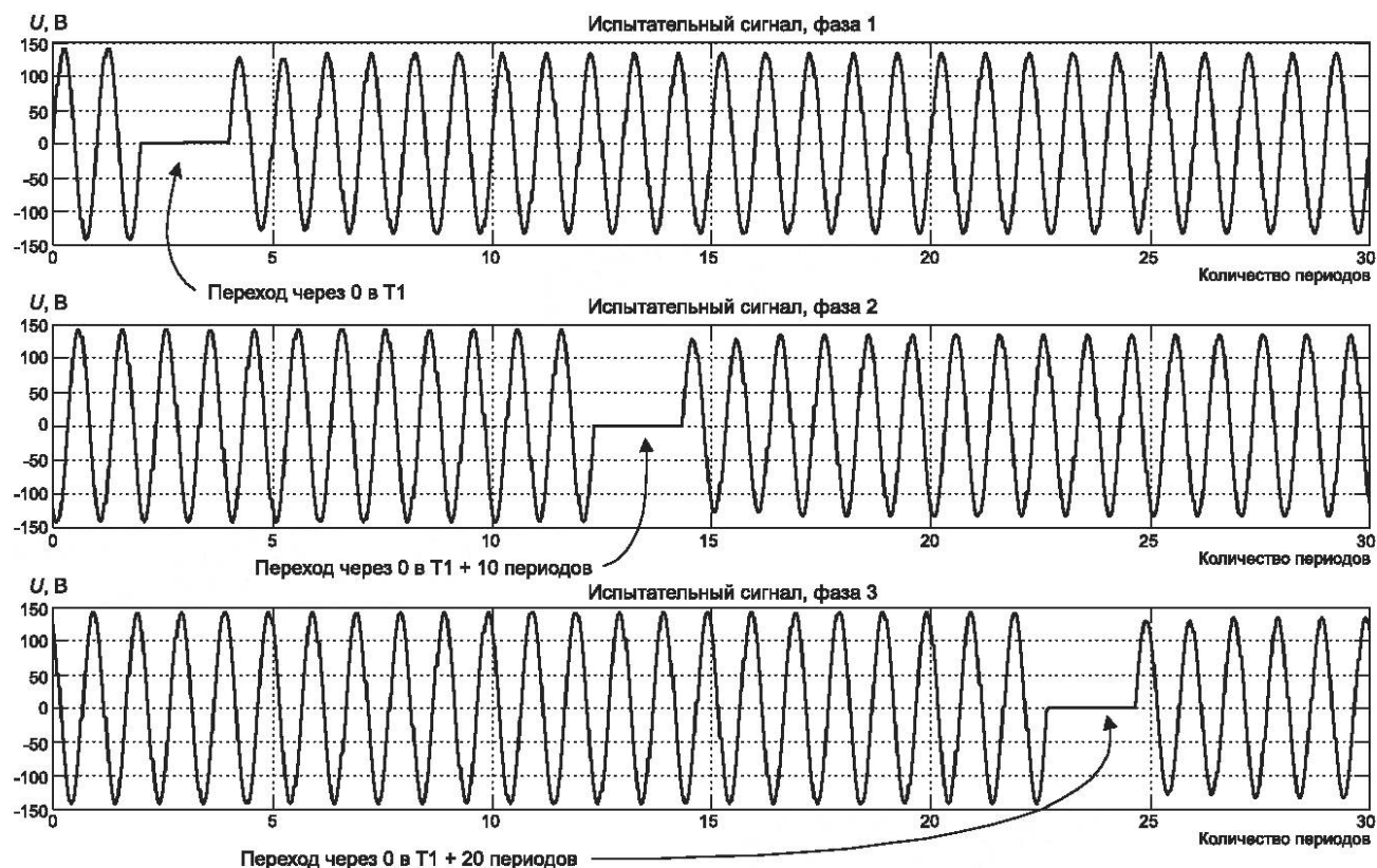
Рисунок 1 — Общее представление испытаний на провалы напряжения в соответствии с испытанием A4.1.1
