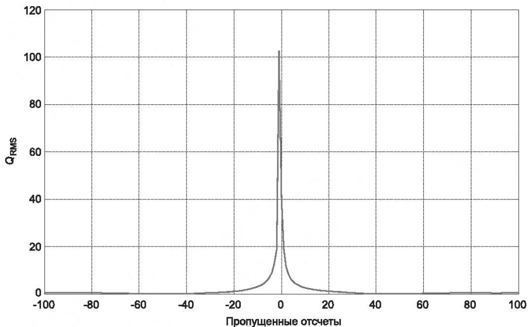
Рисунок G.7 — Q_{RMS} для идеального сигнала, ошибка выборки = -300 \cdot 10^{-6}
