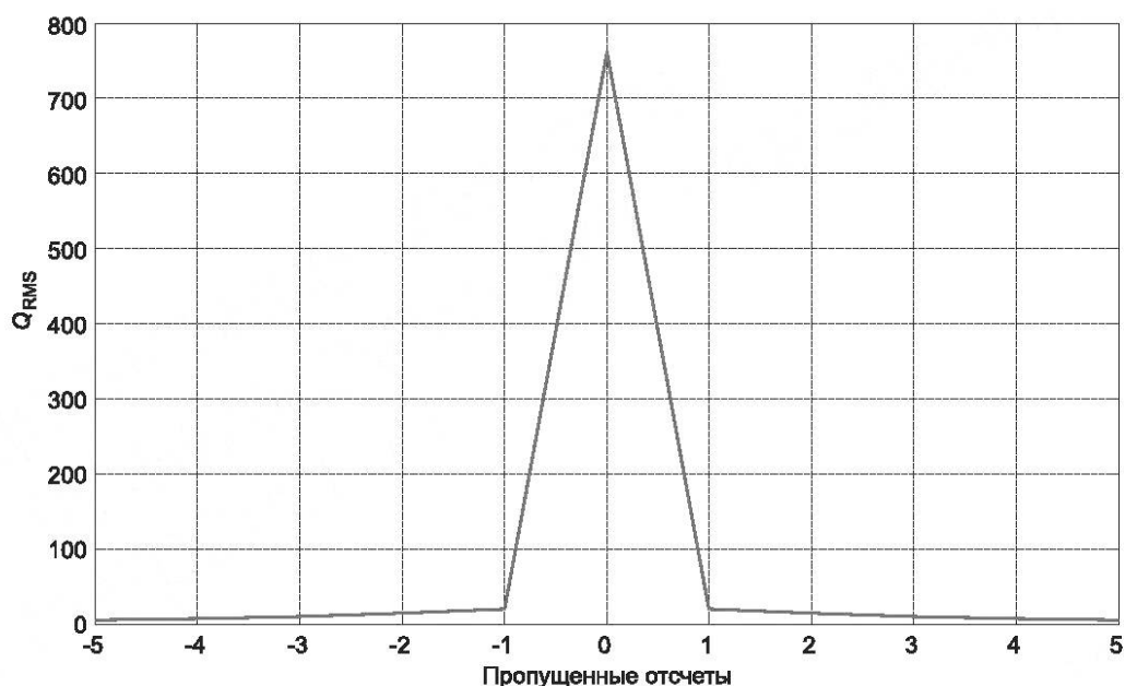
Рисунок G.6 — Обнаружение одного пропущенного отсчета
