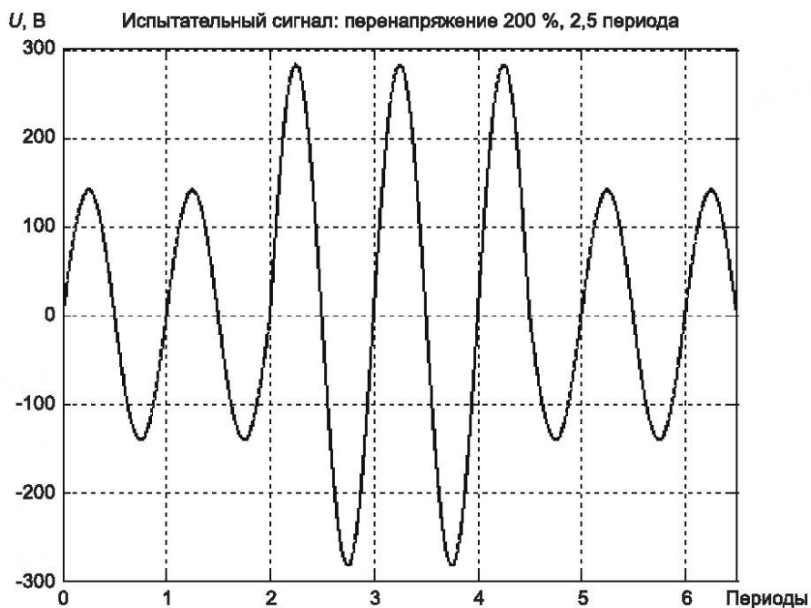
Рисунок 36 — Первая детализация формы сигнала при испытании на перенапряжения в соответствии с испытанием S4.1.2
