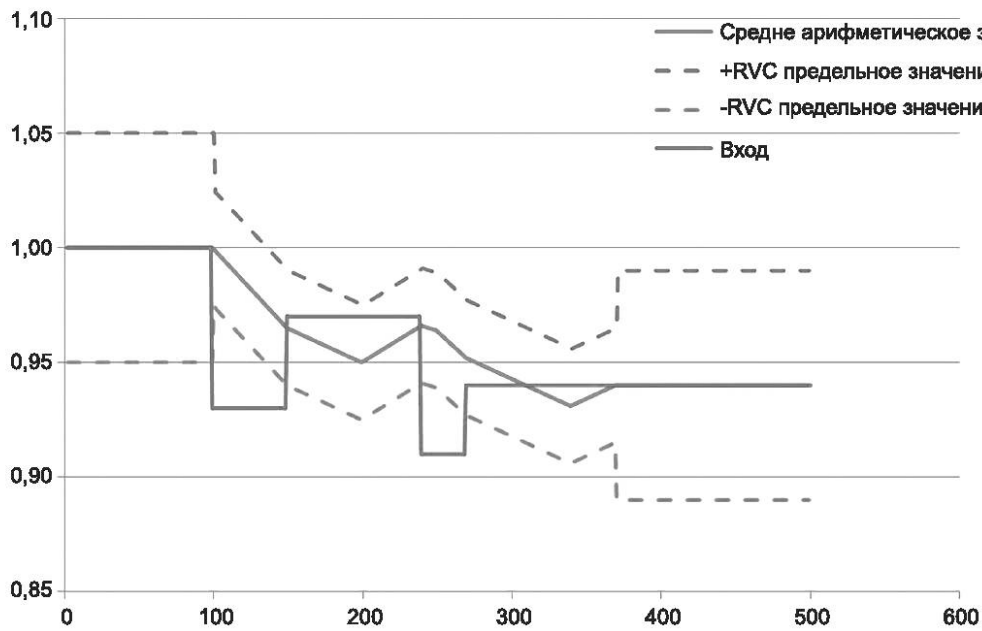
Рисунок 31 — Форма сигнала вместе с RVC-предельными значениями и средним арифметическим значением по A13.5.1
