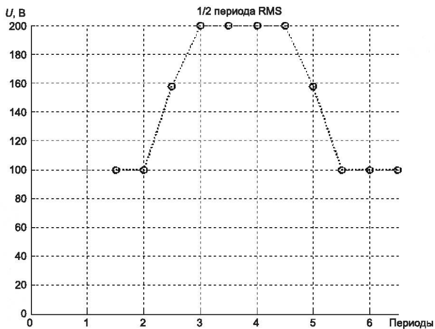
Рисунок 8 — Вторая детализация формы сигнала при испытании на перенапряжения в соответствии с испытанием A4.1.2
