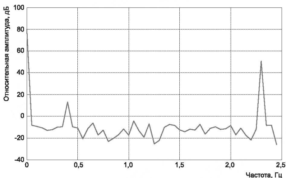
Рисунок G.3 — Нестабильность частоты 2,3 Гц
