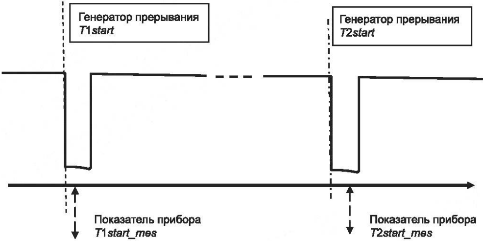
Рисунок 46 — Оценка неопределенности измерения времени
