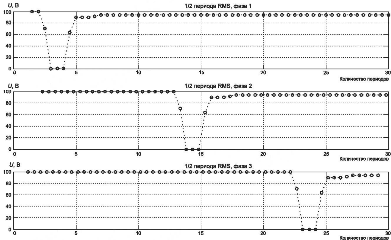
Рисунок 2 — Первая детализация формы сигнала при испытании на провалы напряжения в соответствии с испытанием A4.1.1
