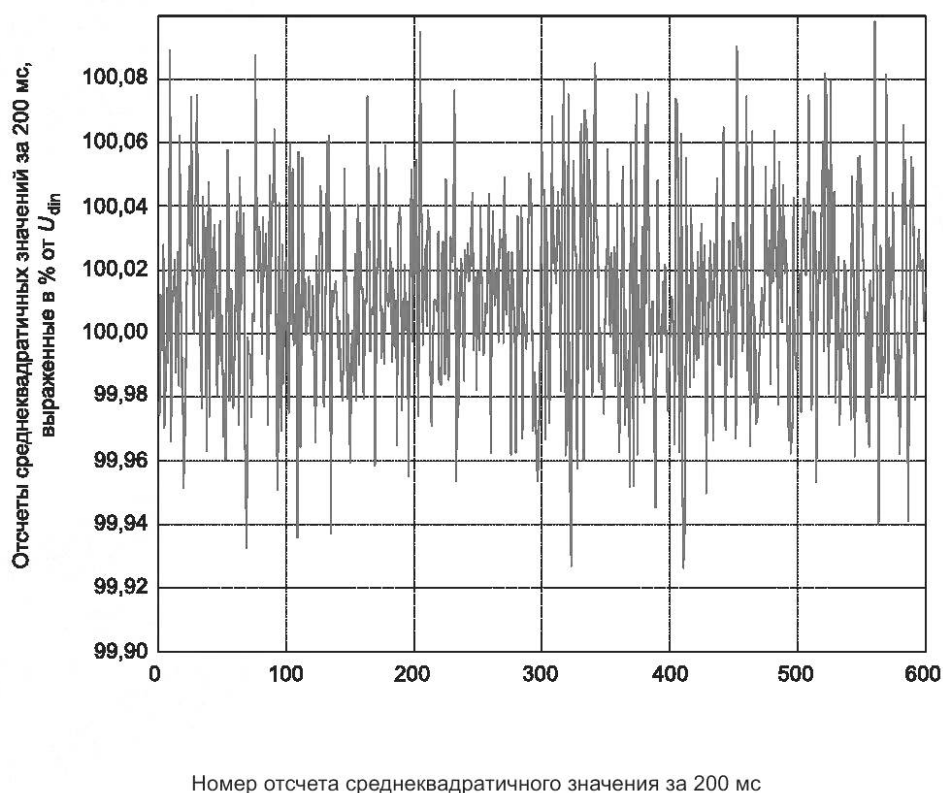
Рисунок G.1 — Моделирование сигнала в условиях шумов
