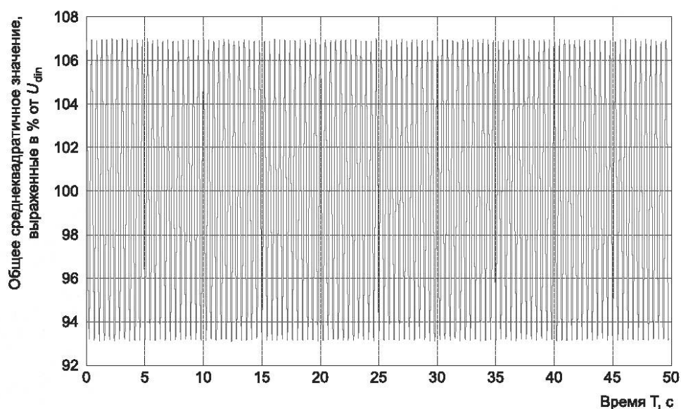
Рисунок G.2 — Осциллограмма для проверки измерения без пропусков среднеквадратичного значения напряжения
