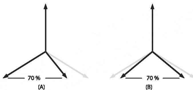
Рисунок D.1 — Испытание «фаза—нейтраль» в трехфазных системах
