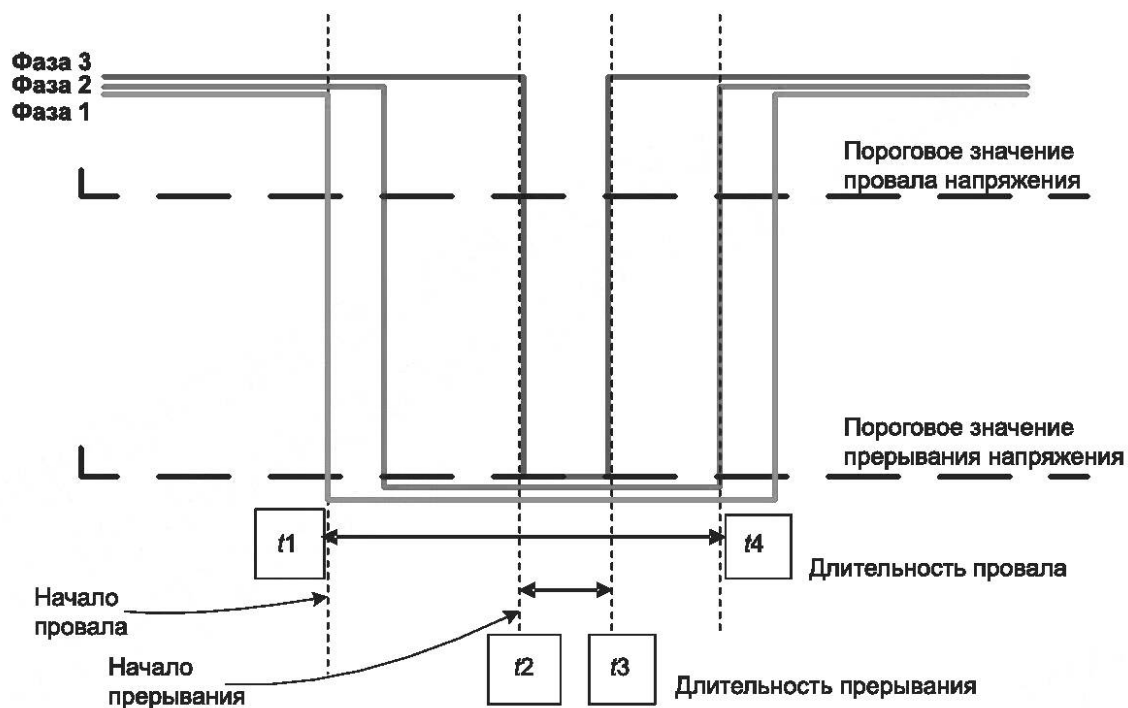
Рисунок 11 — Первая детализация формы сигнала при испытании на провалы/прерывания напряжения в многофазных системах
