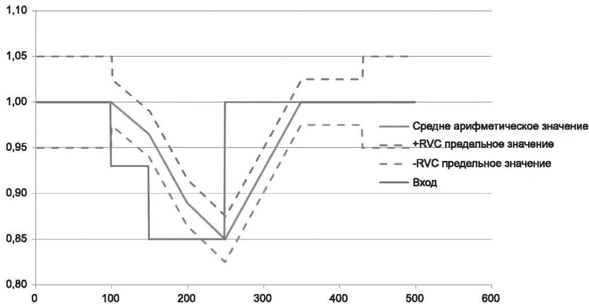
Рисунок 24 — Форма сигнала вместе с RVC предельными значениями и средним арифметическим значением по A13.1.3
