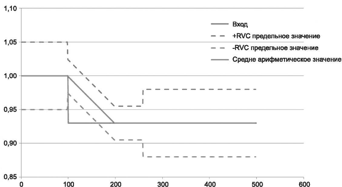
Рисунок 26 — Форма сигнала вместе с RVC предельными значениями и средним арифметическим значением по A13.2.1
