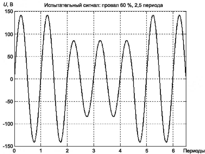
Рисунок 5 — Первая детализация формы сигнала при испытании на провалы напряжения в соответствии с испытанием A4.1.2
