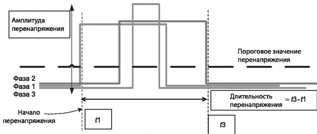
Рисунок 43 — Первая детализация формы волны при испытаниях на перенапряжение в многофазной системе
