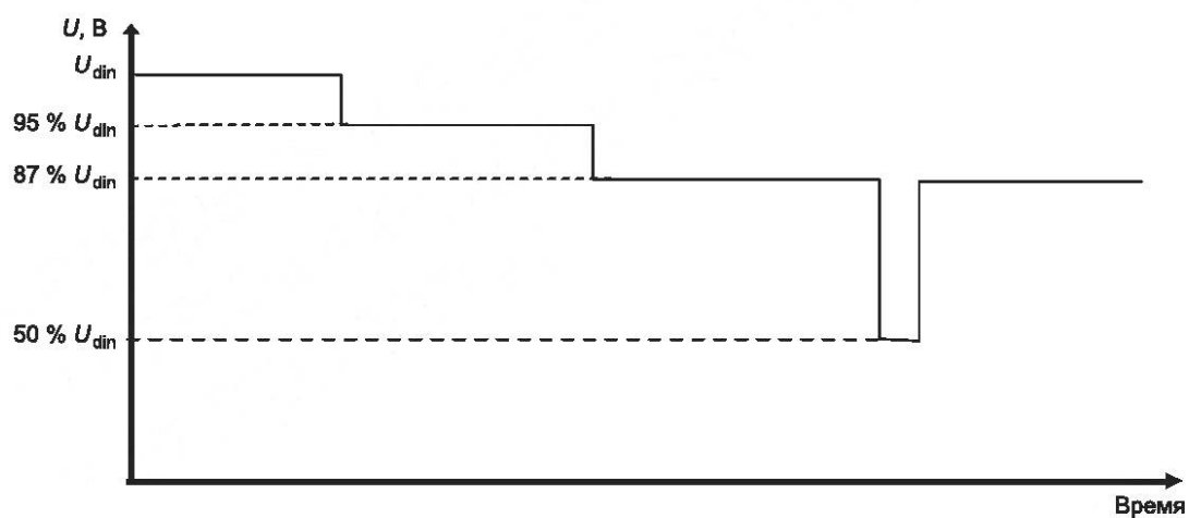
Рисунок 9 — Испытание скользящего опорного напряжения сравнения
