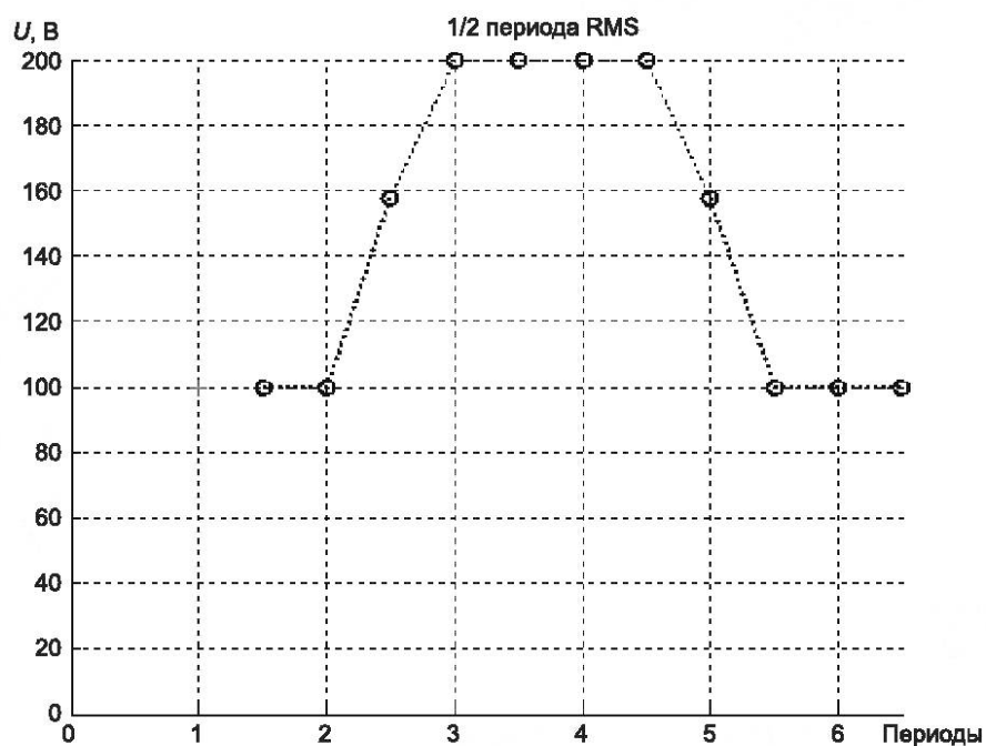
Рисунок 37 — Вторая детализация формы сигнала при испытании на перенапряжения в соответствии с испытанием S4.1.2
