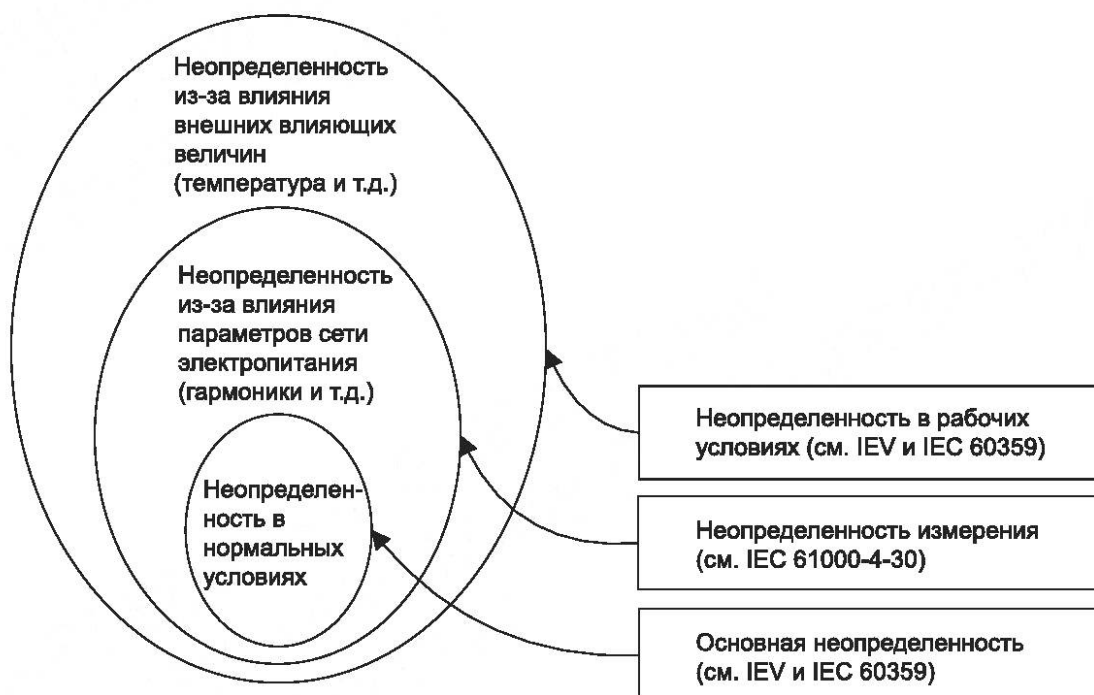
Рисунок А.1 — Различные виды неопределенности
