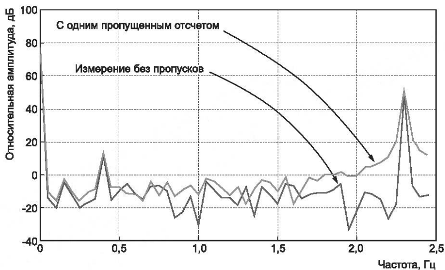
Рисунок G.4 — Спектральные эффекты утечки для пропавшего отсчета
