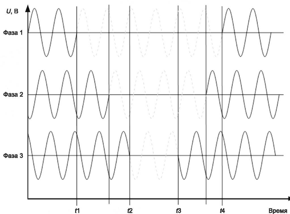
Рисунок 12 — Вторая детализация формы сигнала при испытании на провалы/прерывания напряжения в многофазных системах
