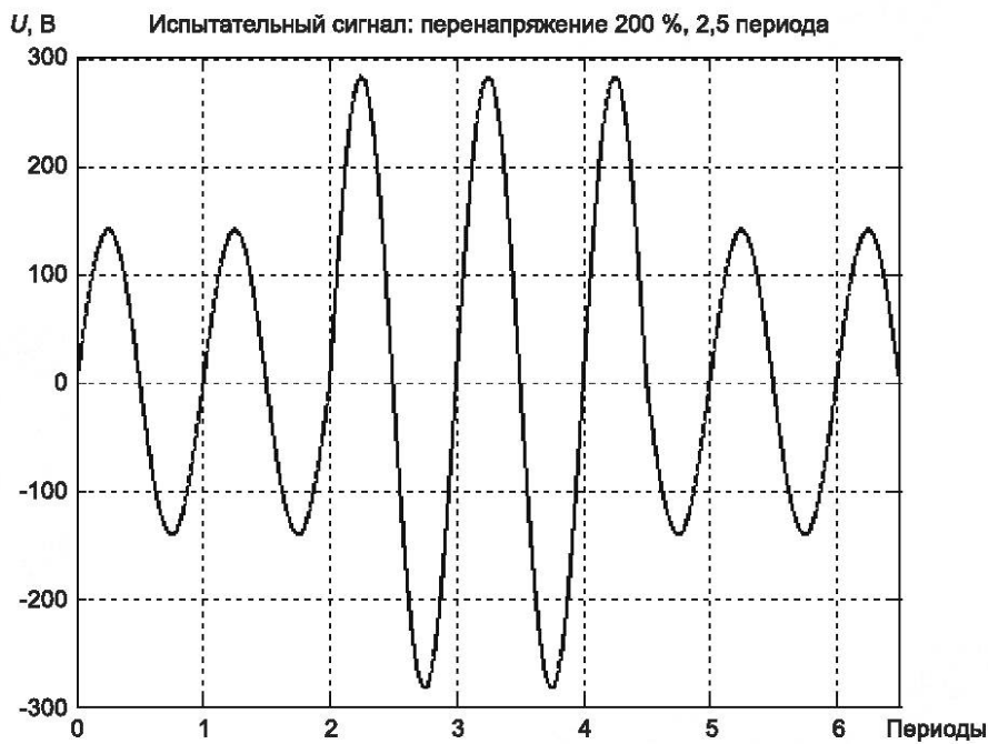
Рисунок 7 — Первая детализация формы сигнала при испытании на перенапряжения в соответствии с испытанием A4.1.2
