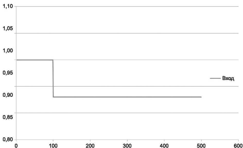
Рисунок 25 — Форма сигнала по A13.2.1
