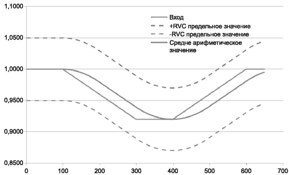
Рисунок 19 — Форма сигнала по A13.1.1
