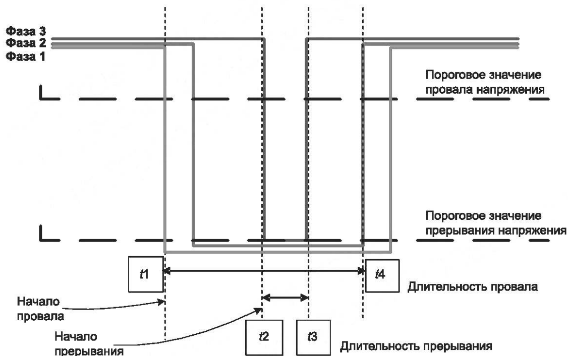
Рисунок 40 — Первая детализация формы сигнала при испытании на провалы или прерывания напряжения в многофазных системах
