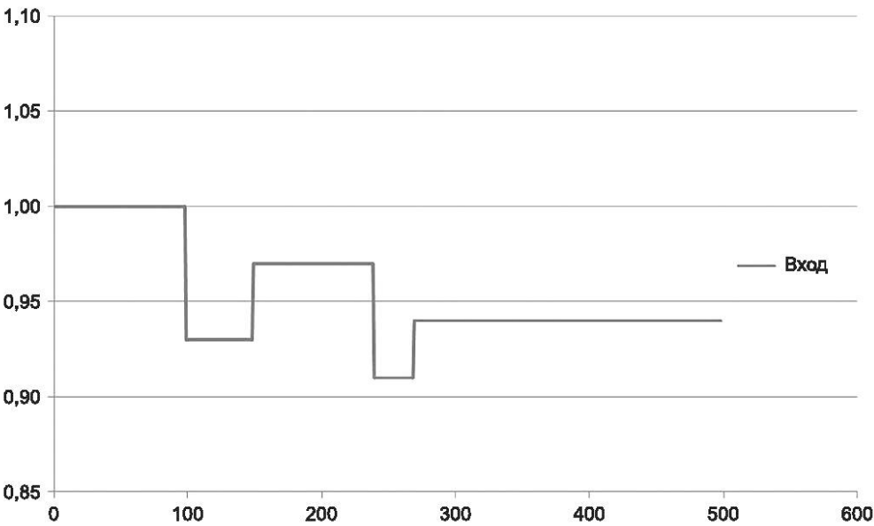
Рисунок 30 — Форма сигнала по A13.5.1
