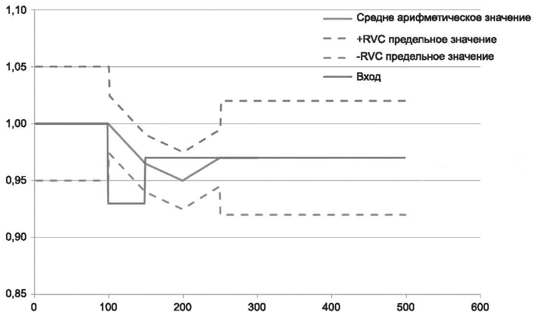
Рисунок 28 — Форма сигнала вместе с RVC предельными значениями и средним арифметическим значением по A13.3.1
