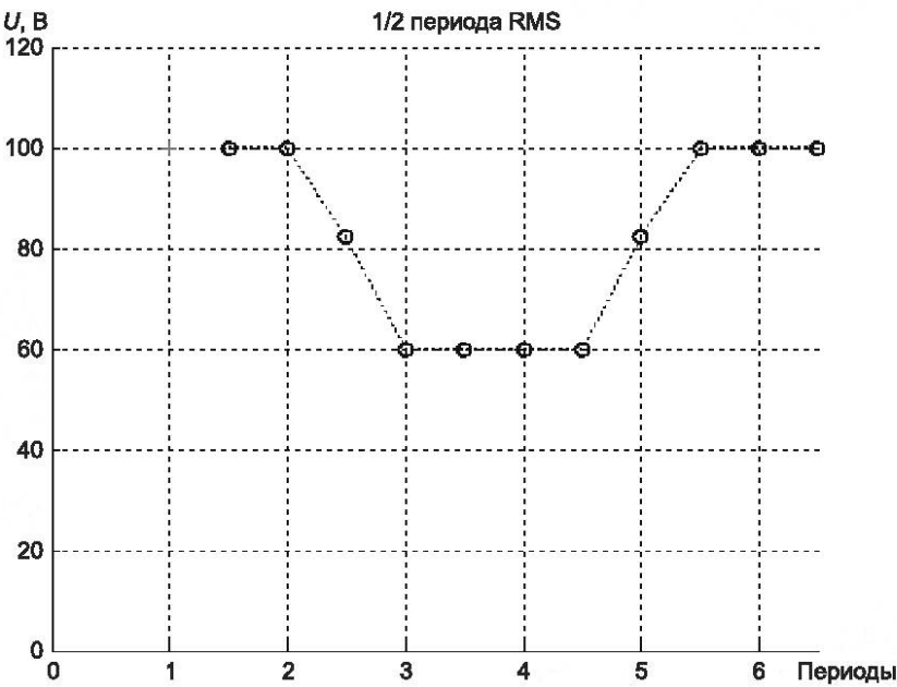
Рисунок 35 — Вторая детализация формы сигнала при испытании на провалы напряжения в соответствии с испытанием S4.1.2
