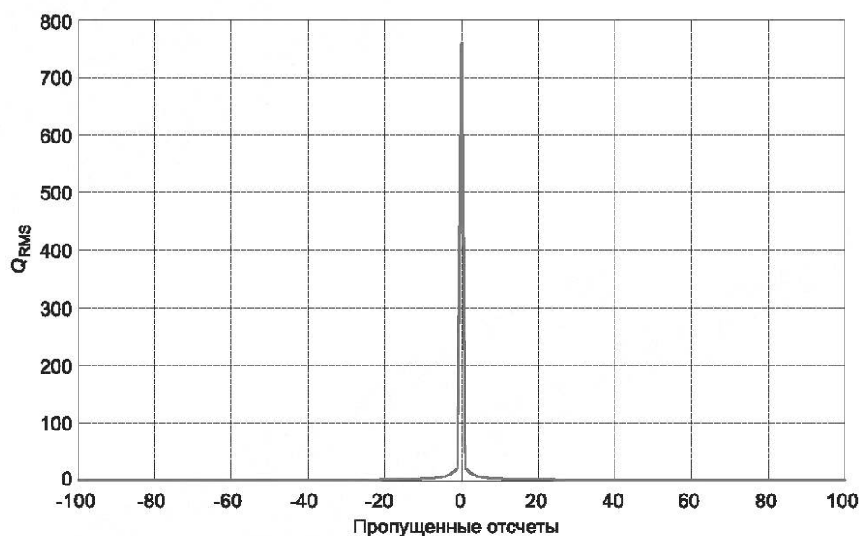
Рисунок G.5 — Иллюстрация Q_{\text{RMS}} для пропущенных отсчетов
