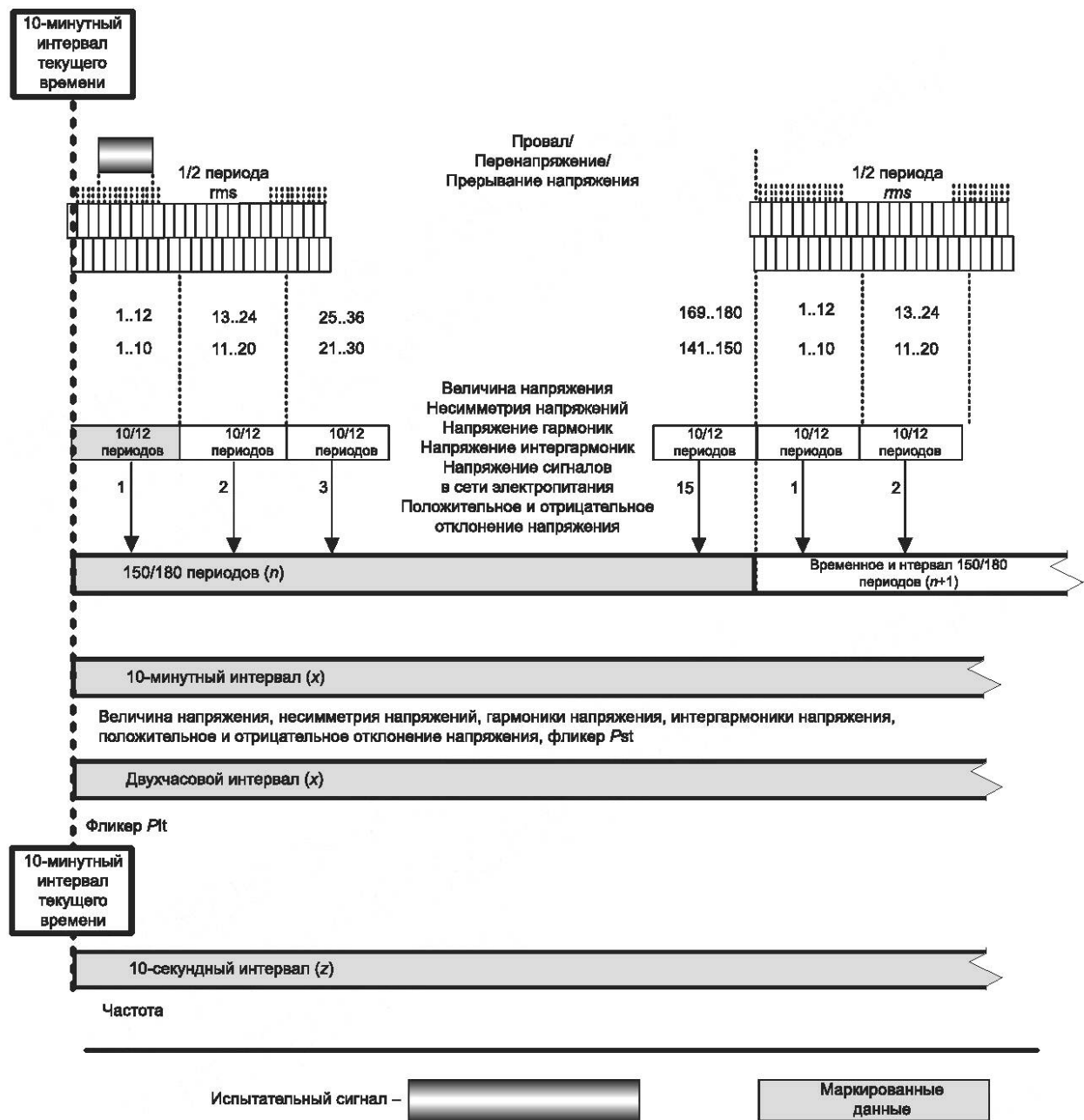
Рисунок 45 — Испытания маркирования для класса S
