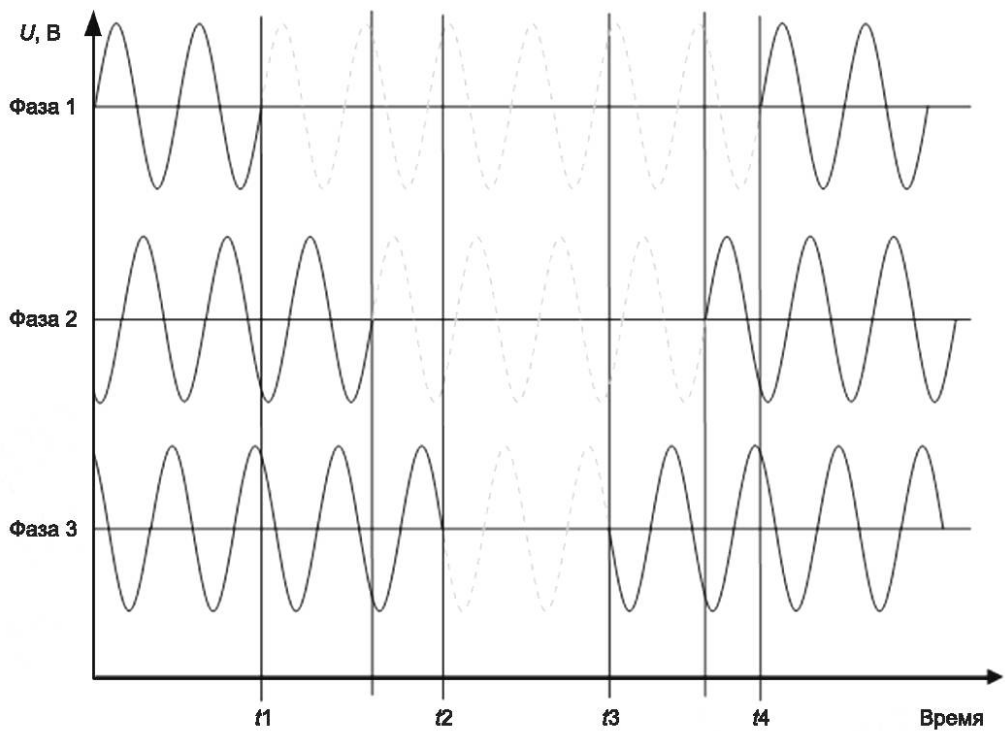
Рисунок 41 — Вторая детализация формы сигнала при испытании на провалы или прерывания напряжения в многофазных системах
