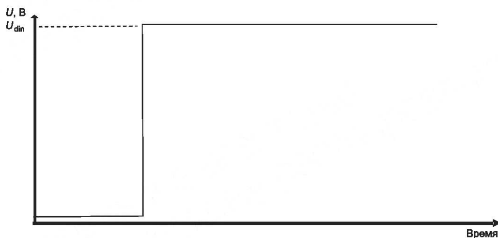
Рисунок 39 — Порог срабатывания при испытаниях скользящего опорного напряжения сравнения
