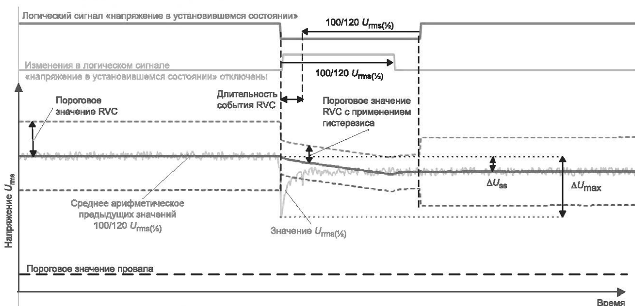
Рисунок 18 — Пример события RVC
