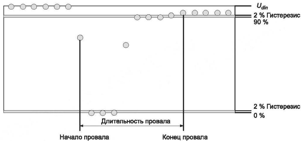
Рисунок 3 — Вторая детализация формы сигнала при испытании на провалы напряжения в соответствии с испытанием A4.1.1
