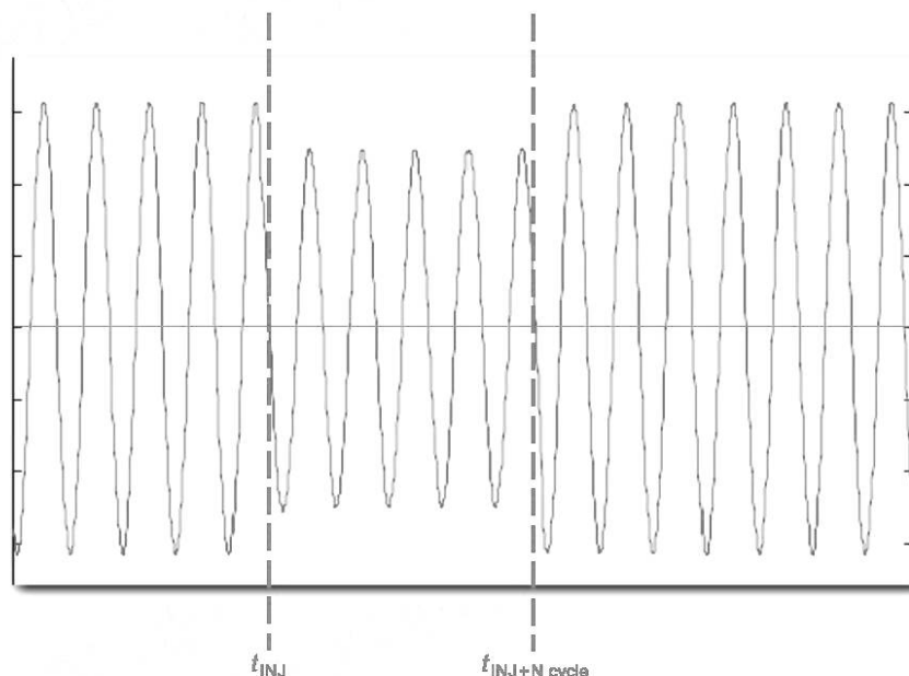
Рисунок Е.1 — Пример для одной фазы, показывающий типичное изменение для N периодов
