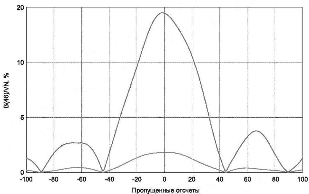
Рисунок G.13 — Амплитудное испытание для колеблющейся составляющей
