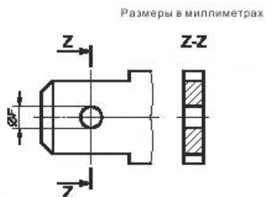
Рисунок К.5 — Размеры отверстий для фиксации
