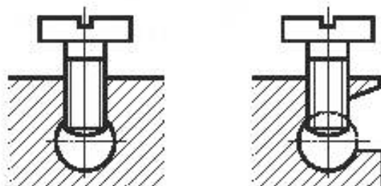
Рисунок IV.1b — Выводы без прижимных пластин
