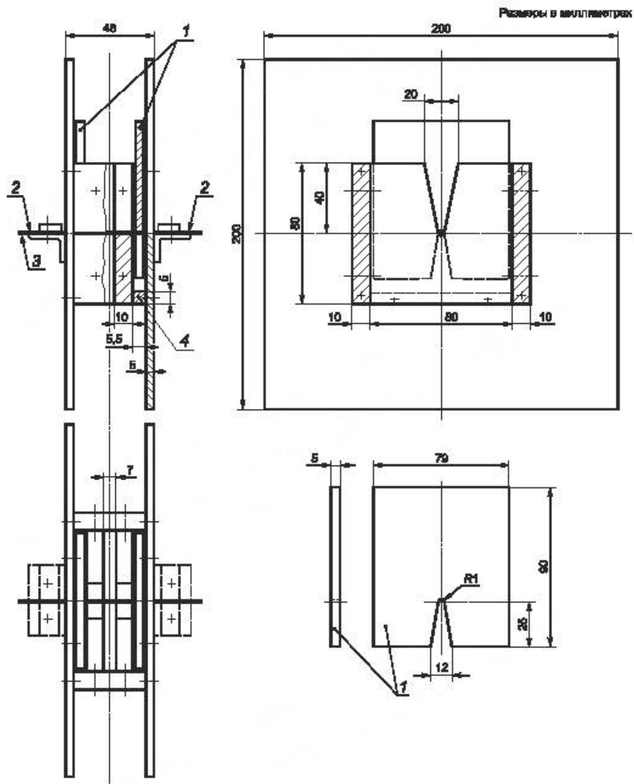
Рисунок IE.1 — Испытательное устройство для проверки устойчивости УЗДП к минимальным значениям I^2t и I_p
