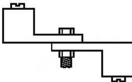
Рисунок L.2 — Пример присоединения выводов УЗДП
