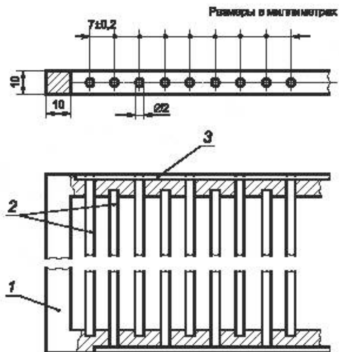
Рисунок С.2 — Решетка
