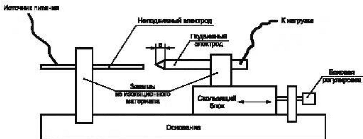
Рисунок 5 — Генератор дуги
