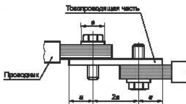
Рисунок L.4 — Пример присоединения выводов УЗДП
