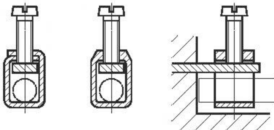
Рисунок IV.1a — Выводы с хомутиком
