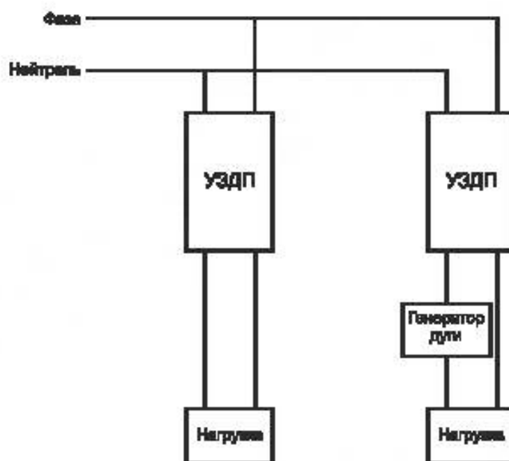
Рисунок 16 — Цель для испытания при перекрестных помехах
