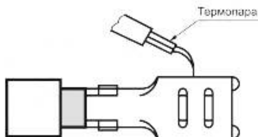
Рисунок К.1 — Пример расположения термодпары при измерении превышения температуры
