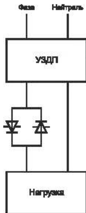
Рисунок 17 — Цепь для испытания управляющего тока
