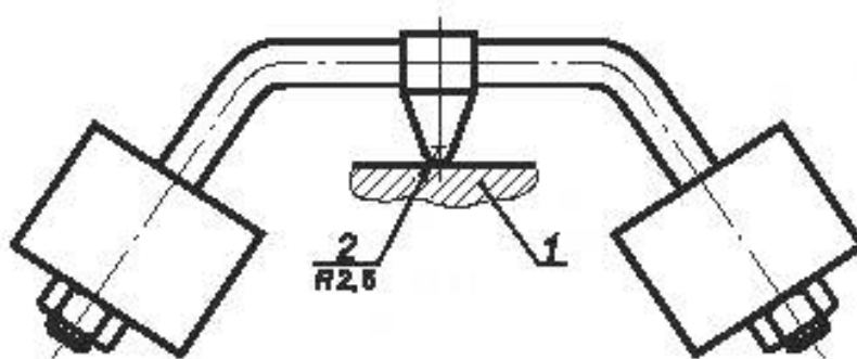
1 — образец; 2 — сфера
