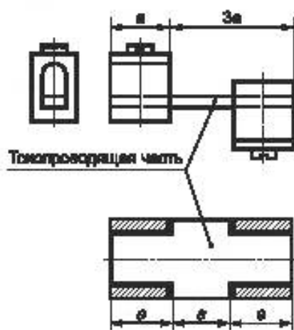
Рисунок L.5 — Пример присоединения выводов УЗДП
