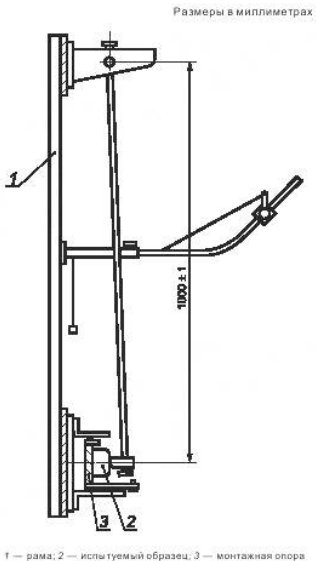
Рисунок 24 — Устройство для испытания на механический удар (9.12.2.2)
