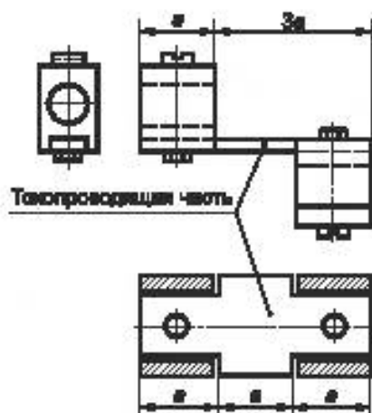
Рисунок L.6 — Пример присоединения выводов УЗДП
