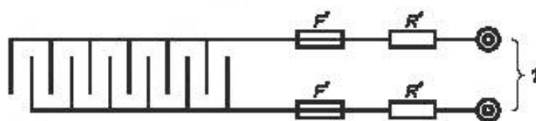
Рисунок С.3 — Электрическая цепь решетки
