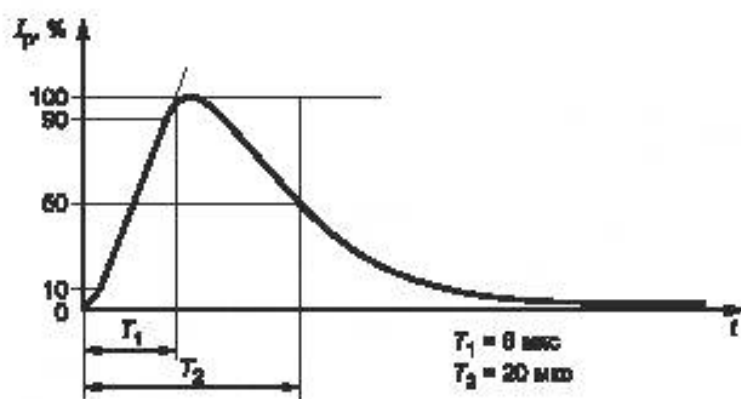
Рисунок 31 — Форма волны импульсного тока 8/20 мкс
