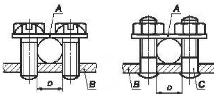
Рисунок IB.2 — Пример винтовых и штыревых выводов
