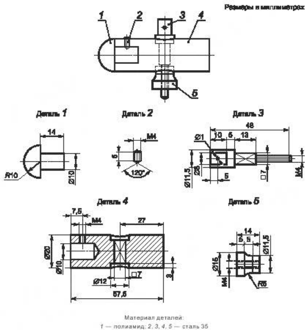
Рисунок 25 — Ударный элемент маятника устройств для испытания на механический удар (9.12.2.2)
