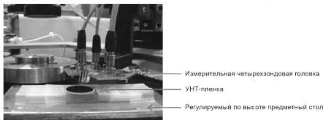
Рисунок 3 — Фотография установки с измерительной четырехзондовой головкой
