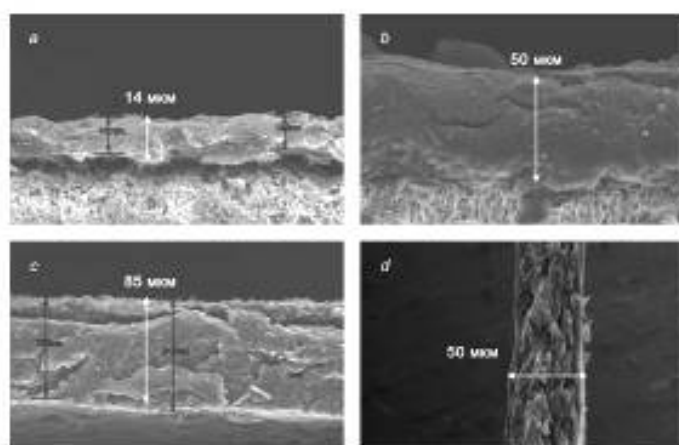
Рисунок А.1 — Изображения УНТ-лент, полученные с помощью автоэмиссионного растрового электронного микроскопа
