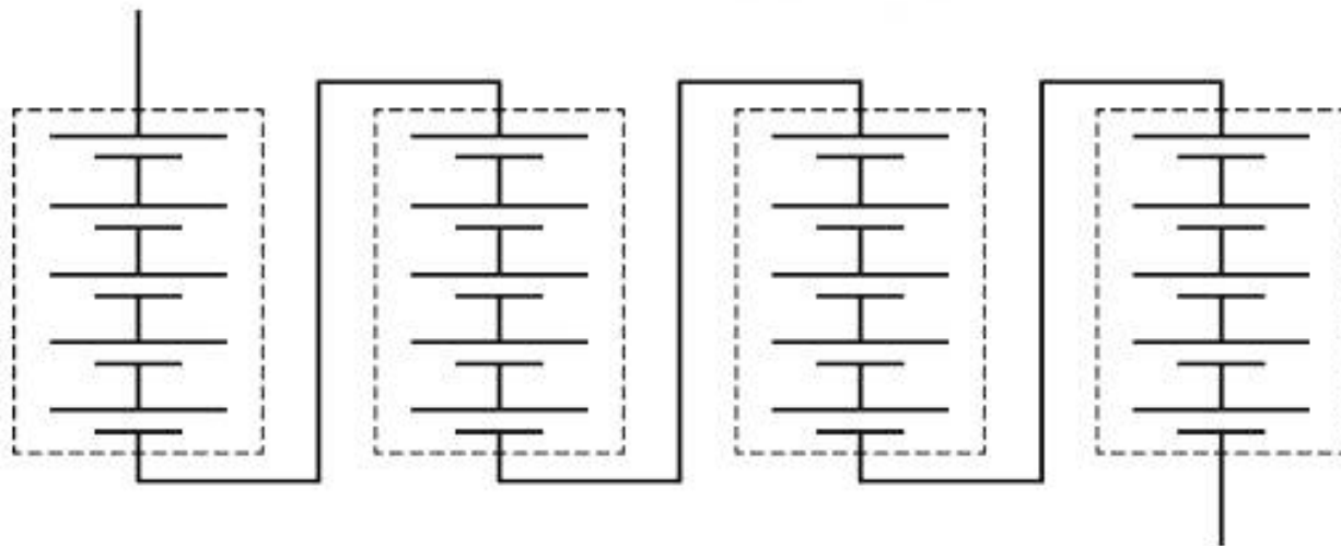
Рисунок А.8 — Структура (5S)4S
