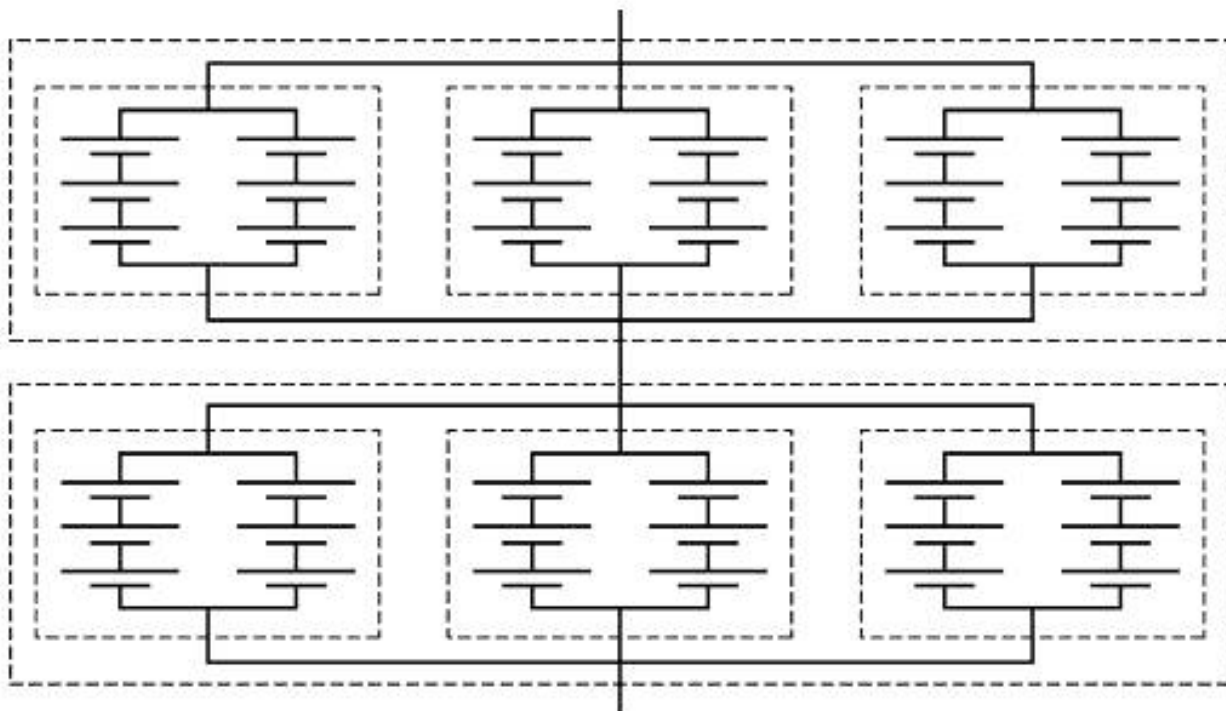
Рисунок А.9 — Структура ((3S2P)3P)2S
