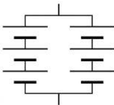
Рисунок А.3 — Структура 3S2P
