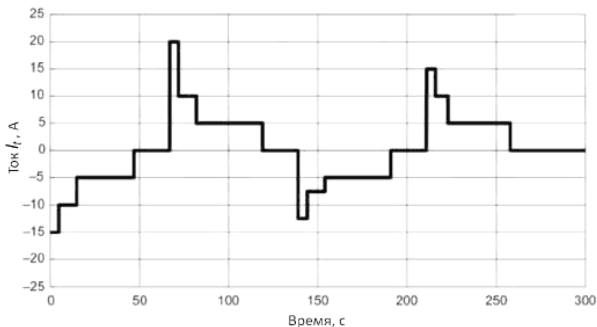
Рисунок 7 — ППЗ при циклировании аккумуляторов для ЭМГ
