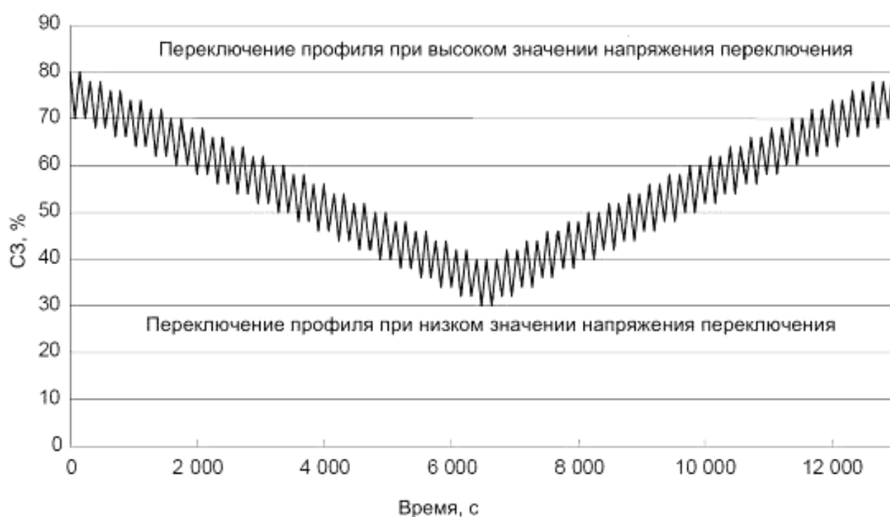
Рисунок 7 — ППЗ при циклировании аккумуляторов для ЭМГ
