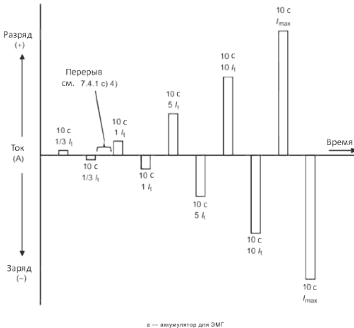
Рисунок 3, лист 1 — Порядок испытаний по определению вольт-амперных характеристик
