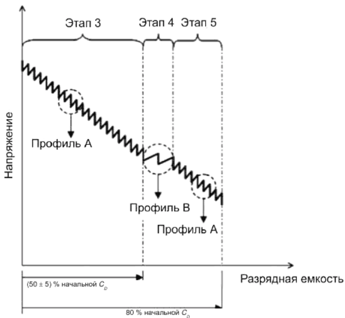
Рисунок В.2 — Концепция циклирования для аккумуляторов ЭМА
