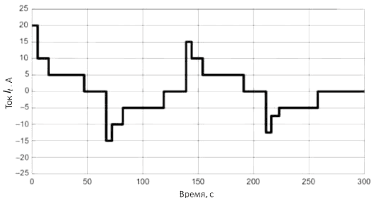
Рисунок 6 — ППР при циклировании аккумуляторов для ЭМГ
