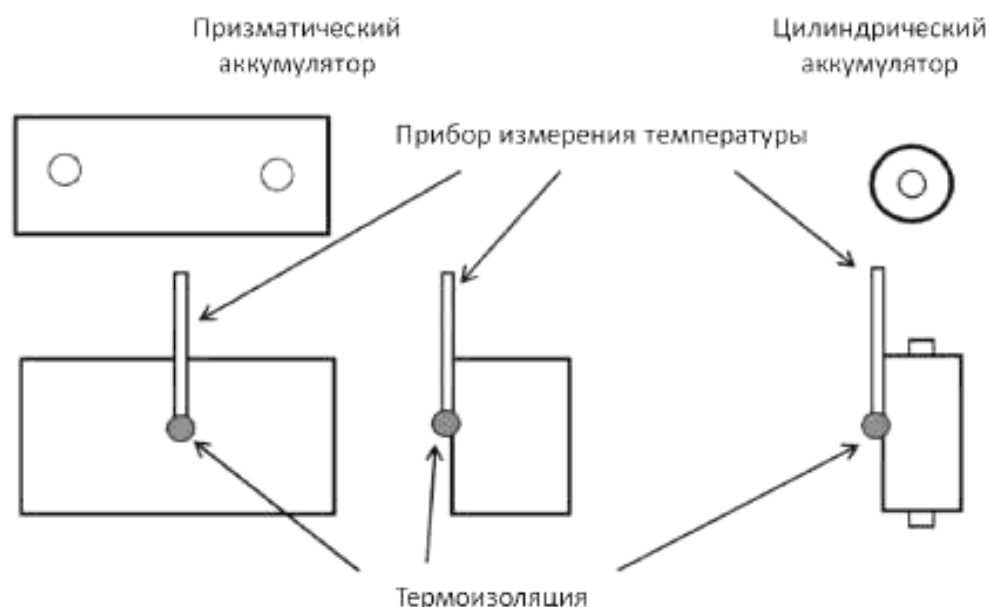
Рисунок 1 — Примеры измерения температуры аккумуляторов
