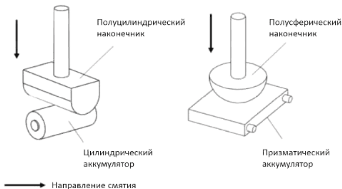
Рисунок 3 — Пример испытания на смятие
