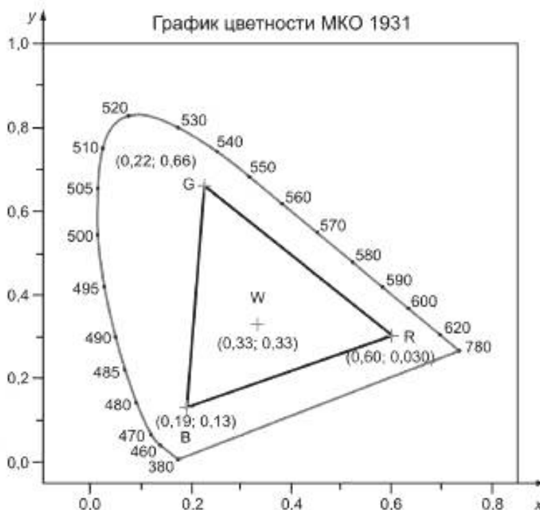
Рисунок 10 — Пример цветовой гаммы дисплея
