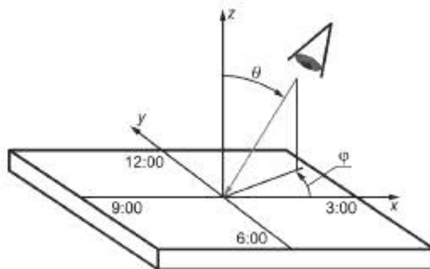
Рисунок 1 — Представление направления обзора или направления измерения, определяемого углом наклона и углом поворота (азимутальным углом) в полярной системе координат
