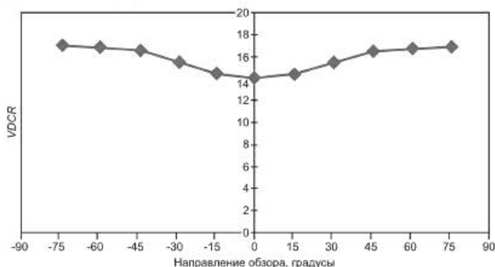
Рисунок 14 — Пример зависимости контрастности от направления обзора
