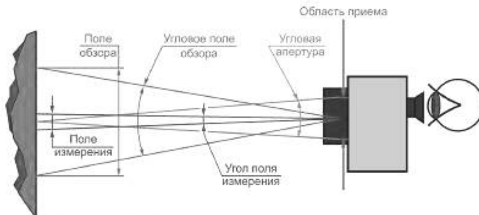
Рисунок 7 — Схема измерительной установки
