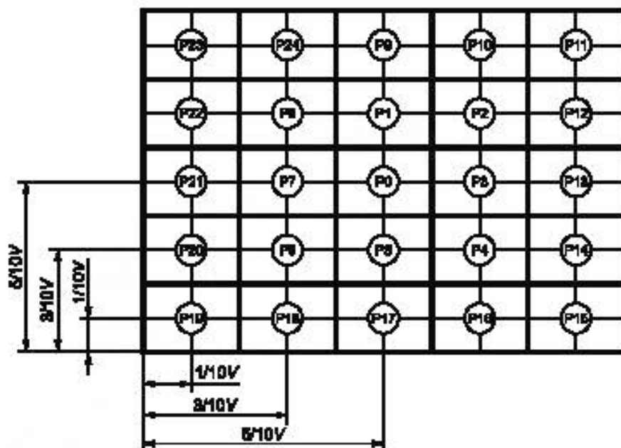
Рисунок 8 — Стандартные позиции измерений
