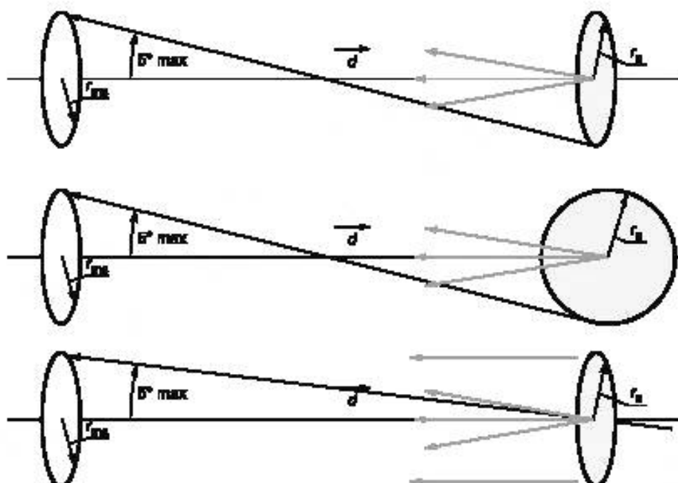
Рисунок 2 — Примеры направленного освещения
