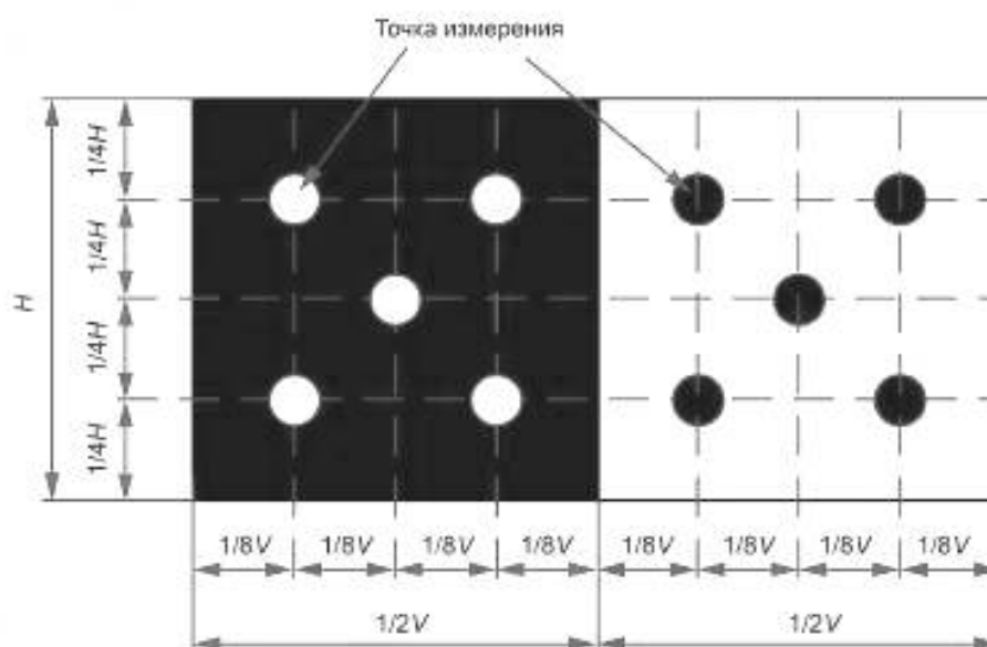
Рисунок 3 — Точки измерения
