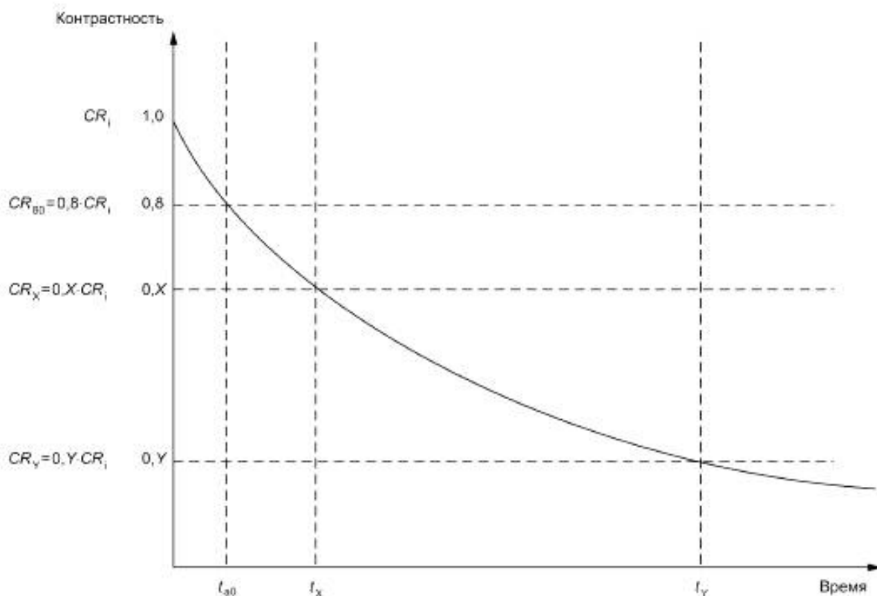
Рисунок 10 — Временные характеристики контрастности
