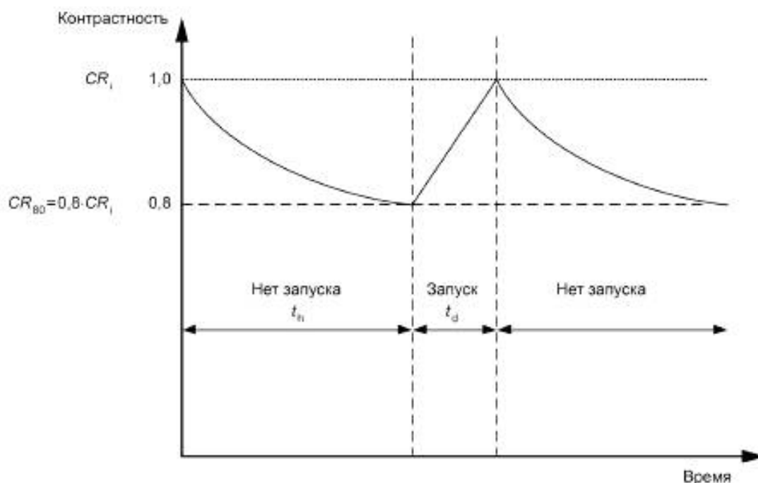
Рисунок 11 — Контрастность изображения и режим запуска
