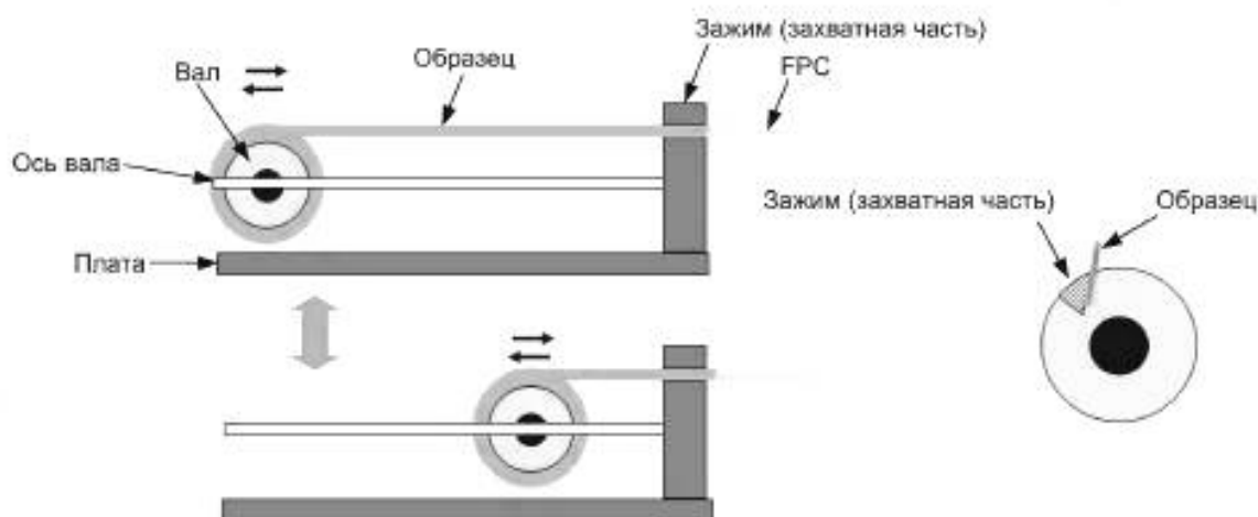
Рисунок 4 — Устройство для испытания на сворачивание (роллинг)
