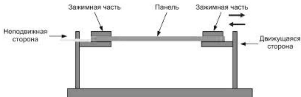
Рисунок 6 — Устройство для испытания на растяжение
