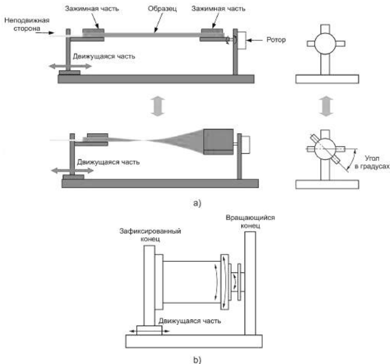
Рисунок 5 — Устройство для испытания на кручение
