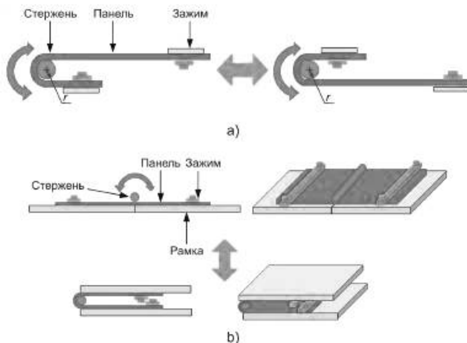
Рисунок 1 — Устройства для различных испытаний на циклический изгиб
