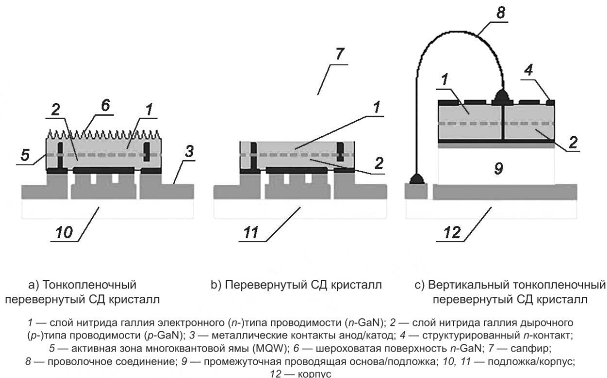
Рисунок G.1 — Схематические изображения СД кристаллов
