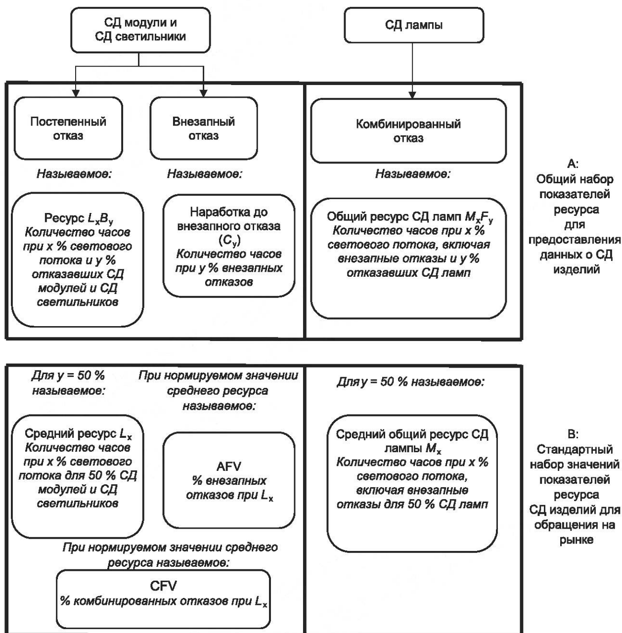
Рисунок С.6 — Общие сведения о различных показателях ресурса СД изделий
