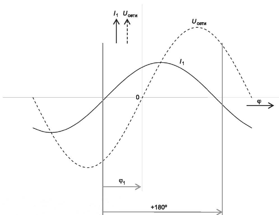
Рисунок Е.1 — Определение угла фазового сдвига \varphi_1 основного тока ( I_1 опережает U_{\text{сети}} , \varphi_1 > 0 )
