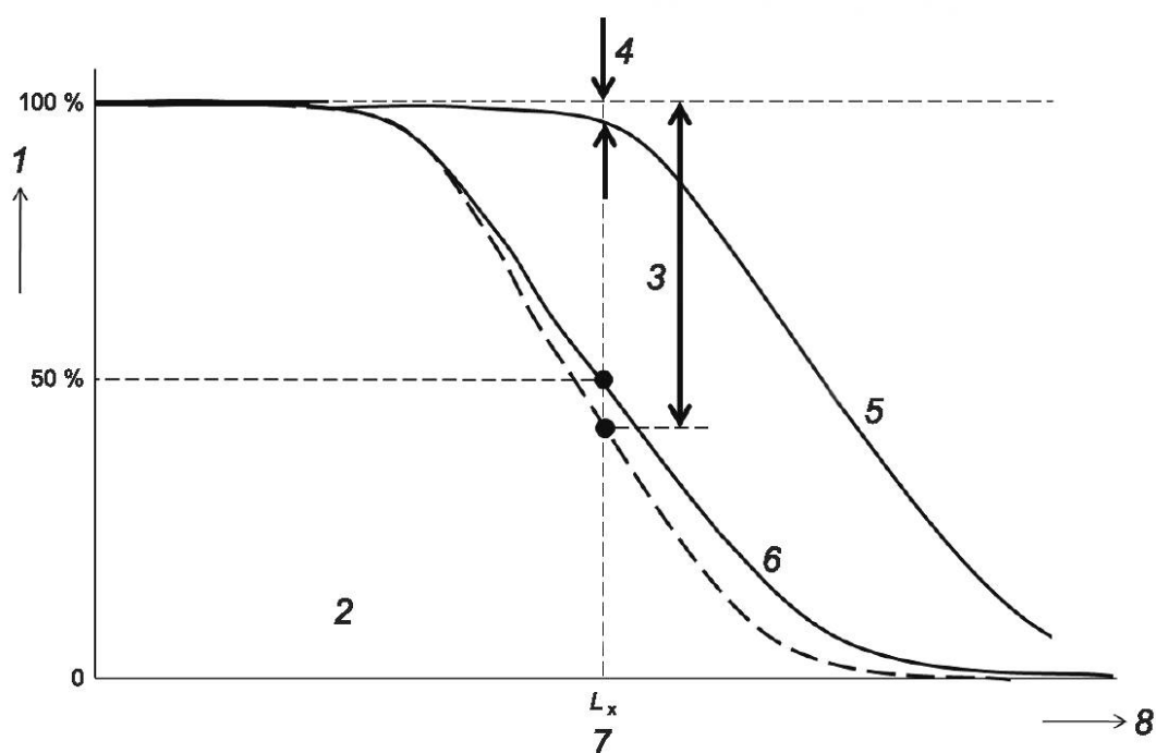
Рисунок С.4 — Кривая доверительной вероятности постепенного отказа R_{\text{постепенное}}
