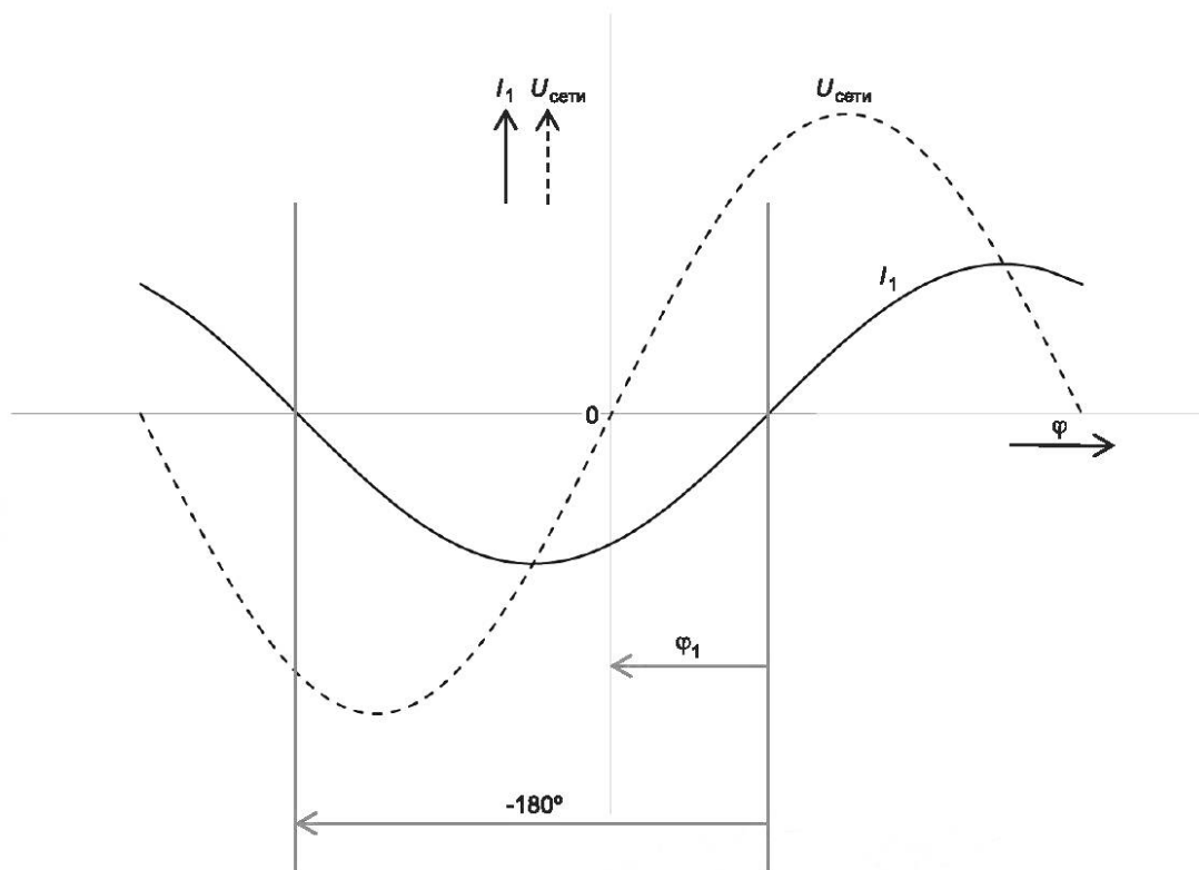
Рисунок Е.2 — Определение угла фазового сдвига \varphi_1 основного тока ( I_1 отстает от U_{\text{сети}} , \varphi_1 < 0 )
