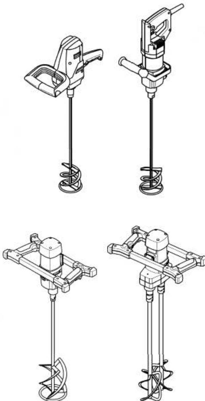
Рисунок 101 — Смесители с различными конфигурациями рукояток и шпинделей
