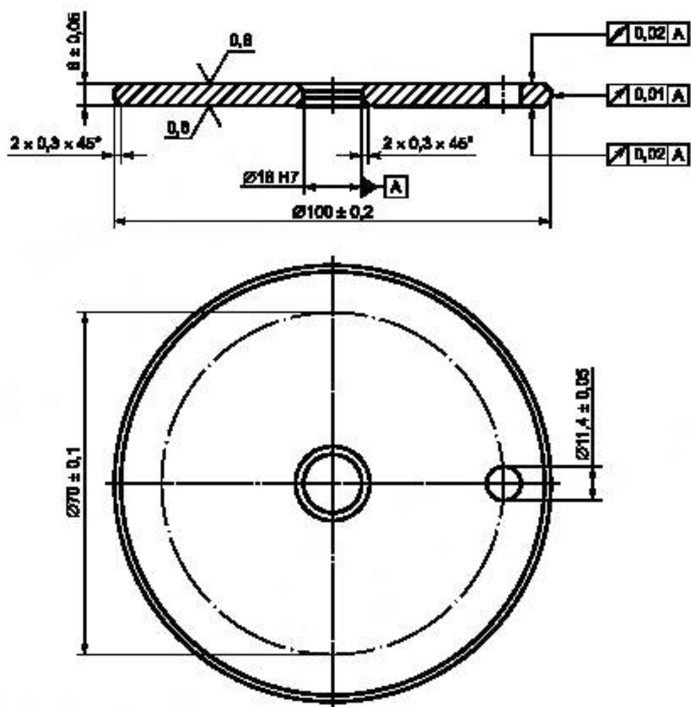
Рисунок I.103 — Диск с дисбалансом
