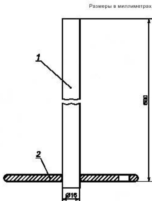
Рисунок I.102 — Испытательная насадка для смесителя
