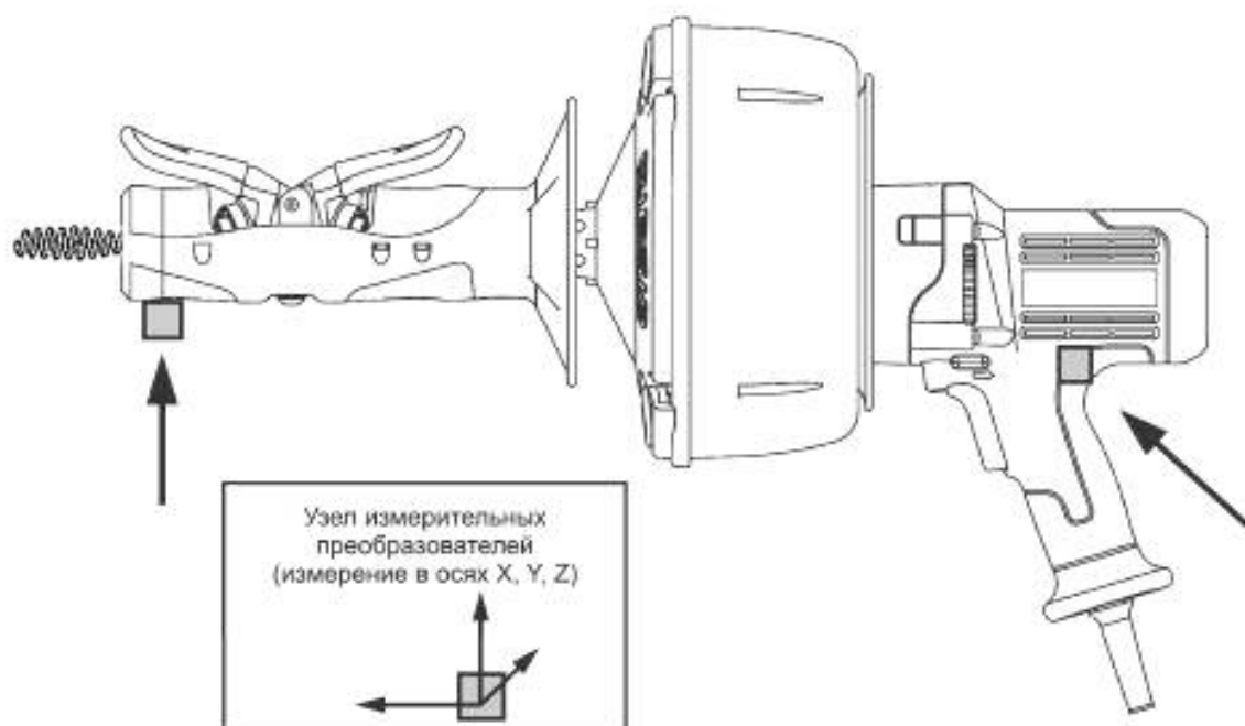
Рисунок I.101 — Расположение измерительных преобразователей для машины
