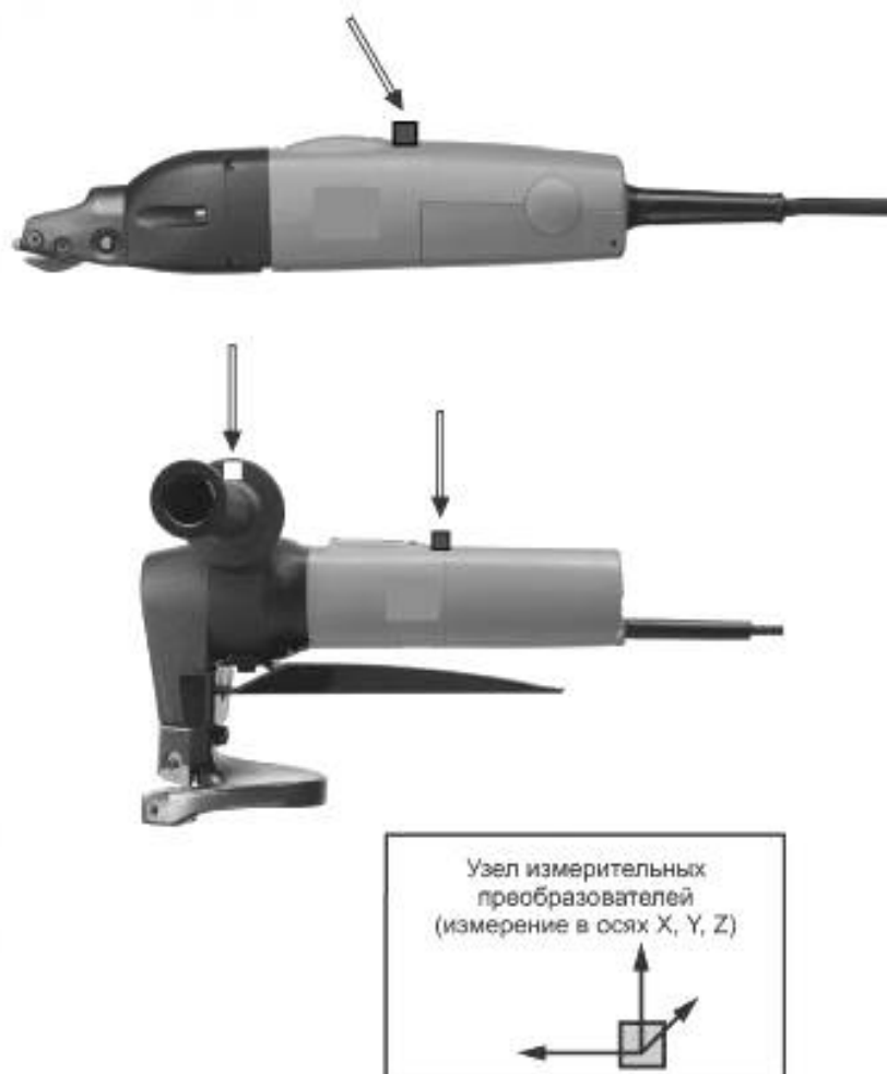
Рисунок I.101 — Расположение измерительных преобразователей для ножниц
