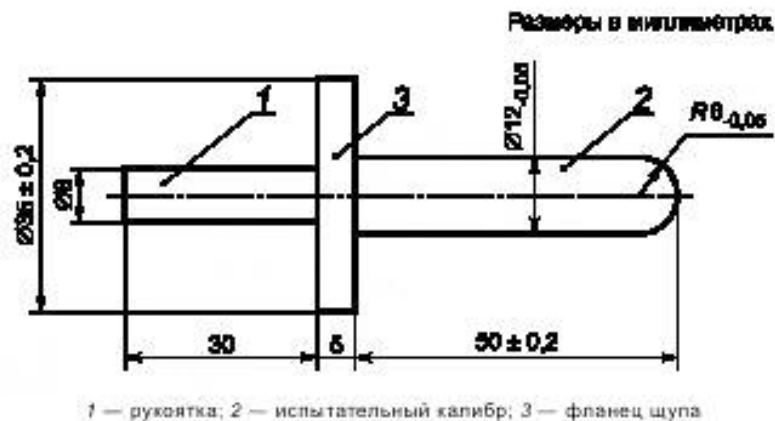
Рисунок 102 — Испытательный щуп
