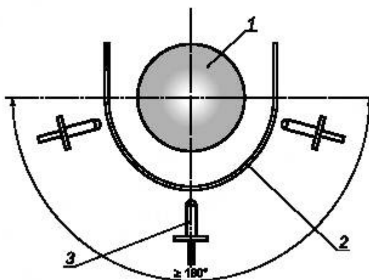
Рисунок 103 — Испытание защитного кожуха сверлильного патрона (вид сверху)
