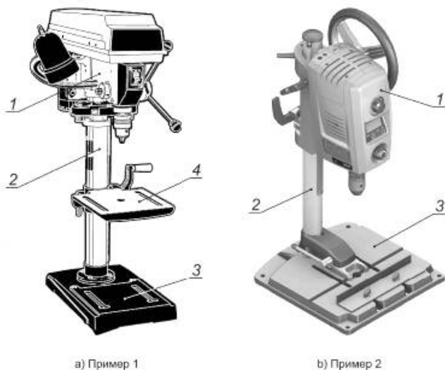
Рисунок 101 — Примеры конструкций сверлильных машин
