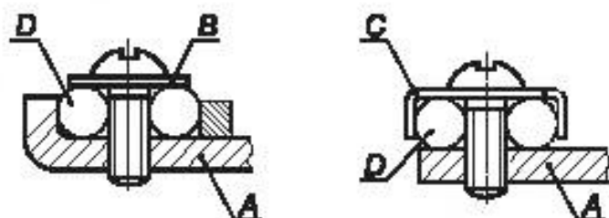
А — зафиксированная часть; В — шайба или прижимная пластина; С — устройство, ограничивающее расплющивание проводника; D — пространство для укладки проводника
