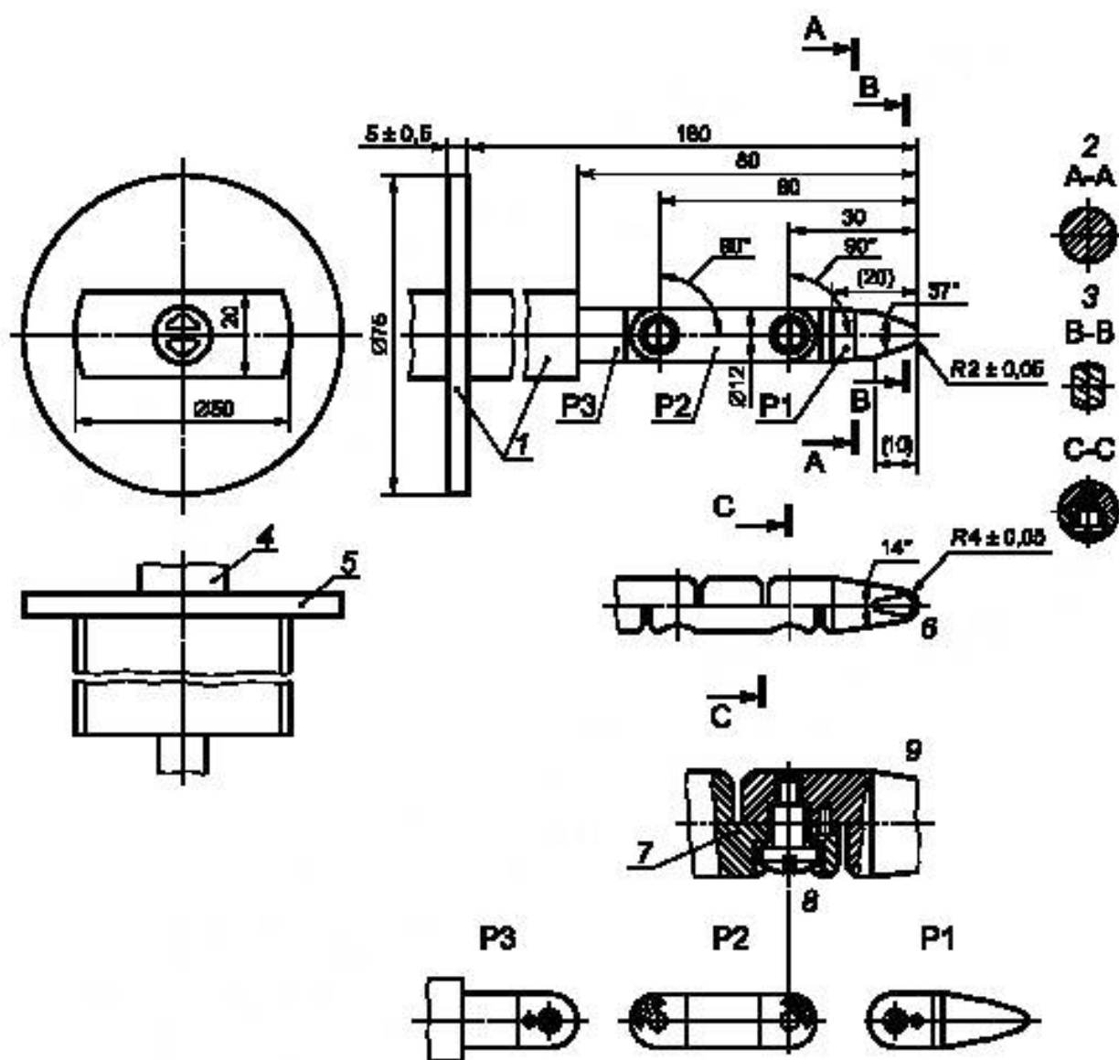
1 — изоляционный материал; 2 — разрез A-A; 3 — разрез B-B; 4 — рукоятка; 5 — стопорная пластина; 6 — сферический край; 7 — деталь х (пример); 8 — вид сбоку; 9 — фаска всех ребер
