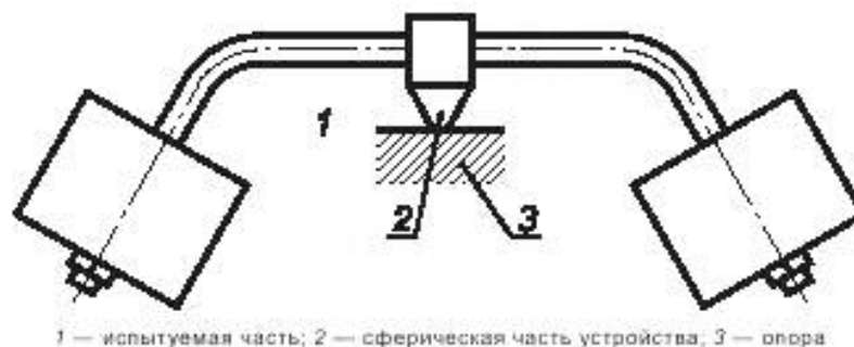
Рисунок 14 — Устройство для испытания давлением шарика
