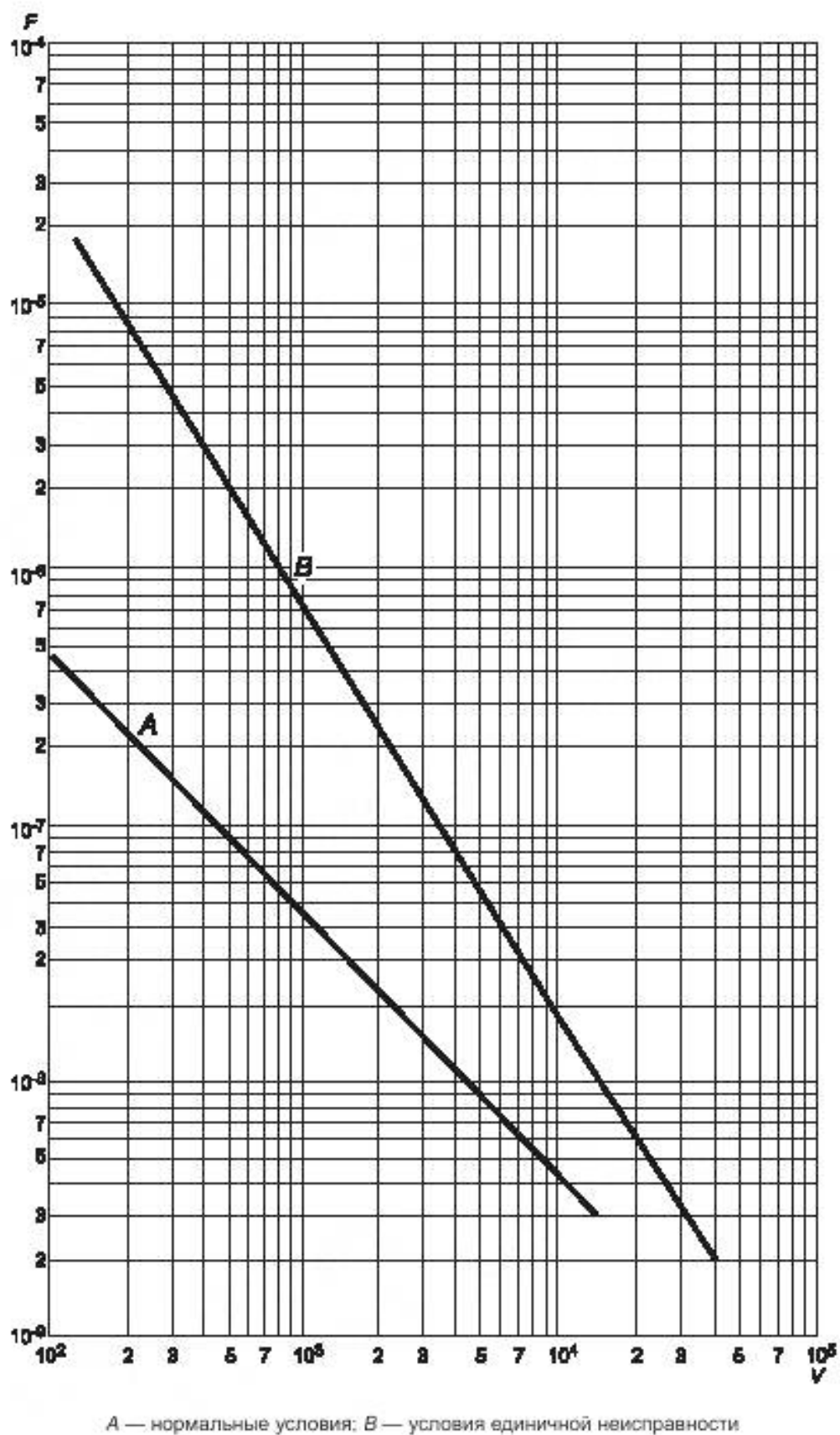
Рисунок 3 — Значение емкости в зависимости от напряжения в нормальных условиях и условиях единичной неисправности (см. перечисление с) 6.3.1 и перечисление с) 6.3.2)
