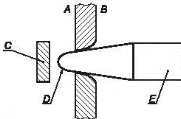
А — область внутри оборудования; В — область за пределами оборудования; С — опасная для жизни часть; D — конец испытательного пальца, который рассматривается как доступный; E — испытательный палец
