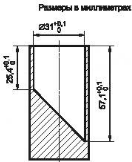
Рисунок 16 — Цилиндр для проверки размеров небольших компонентов
