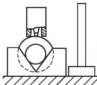
б) Образец помещен в V-образный блок
