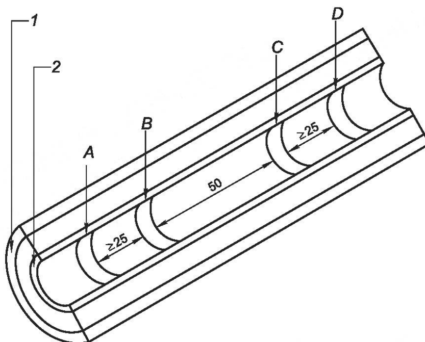
а) Испытуемый образец для определения объемного удельного электрического сопротивления экрана по жиле
