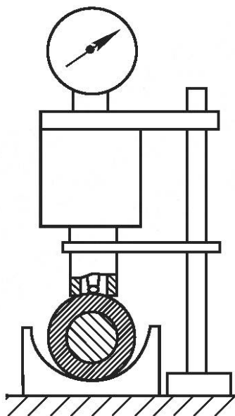
а) Образец помещен в канавку
