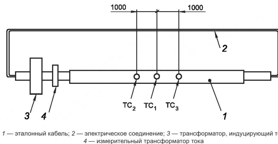
Рисунок А.5 — Эталонный кабель для нагрева одножильных кабелей
