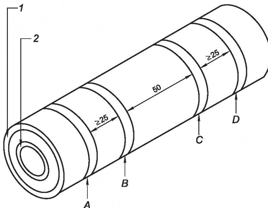
б) Испытуемый образец для определения объемного удельного электрического сопротивления экрана по изоляции
