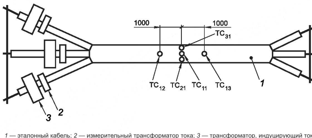
Рисунок А.6 — Эталонный кабель для нагрева трехжильных кабелей
