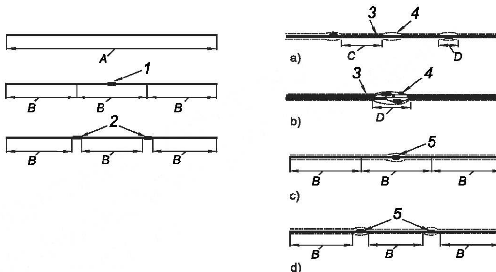
1 — соединительная муфта в средней секции; 2 — соединительные муфты; 3 — броня; 4 — фазовая(ые) муфта(ы); 5 — фазовая муфта или часть кабеля, имеющая механическую особенность; А — не менее шести полных витков; В — не менее двух полных витков; С — не менее одного шага скрутки брони; D — часть кабеля, имеющая механическую особенность
