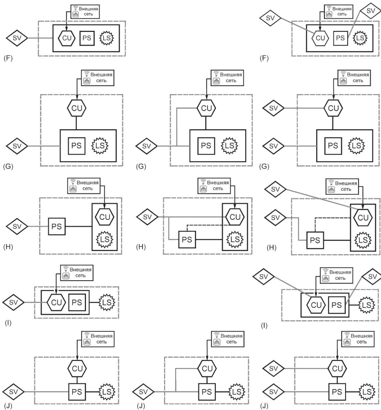
а) Одно напряжение питания
