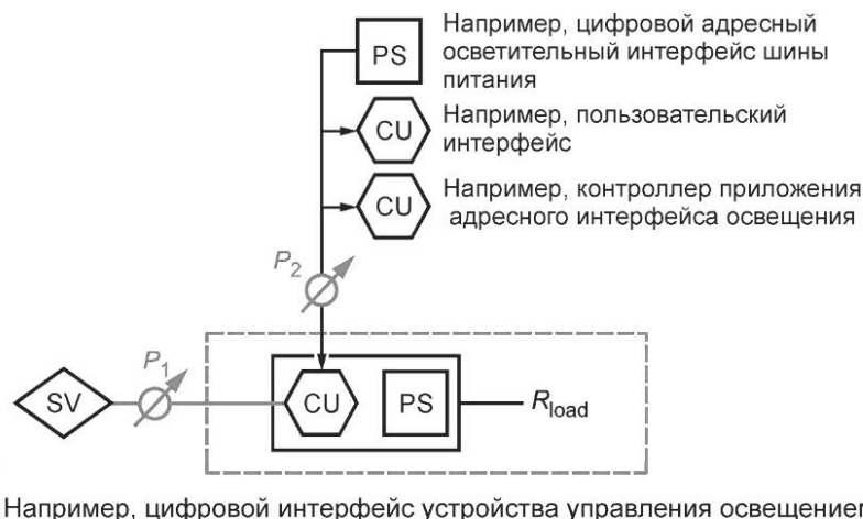
Рисунок D.2 — Пример измерительной установки для «базового» устройства управления в режиме ожидания
