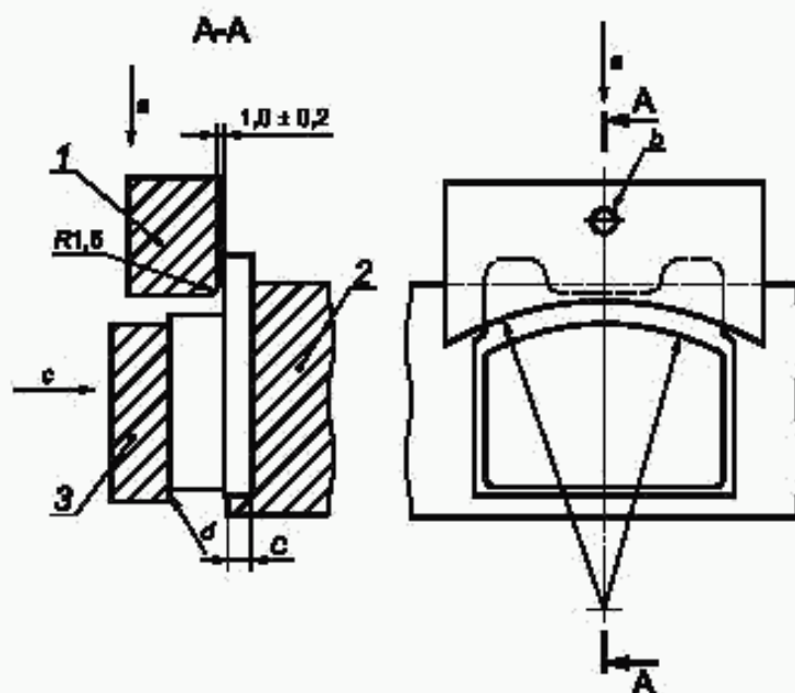
1 — нагружающее устройство (параллельно опоре колодки); 2 — опора колодки; 3 — прижимное устройство; расстояние c \leq толщине колодки; a — направление силы сдвига; b — точка опоры; c — прижимная нагрузка; d — трение, сведенное к минимуму на границе поверхности
