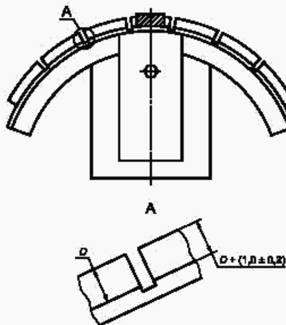
Рисунок 1 — Колодка для испытания части накладки
