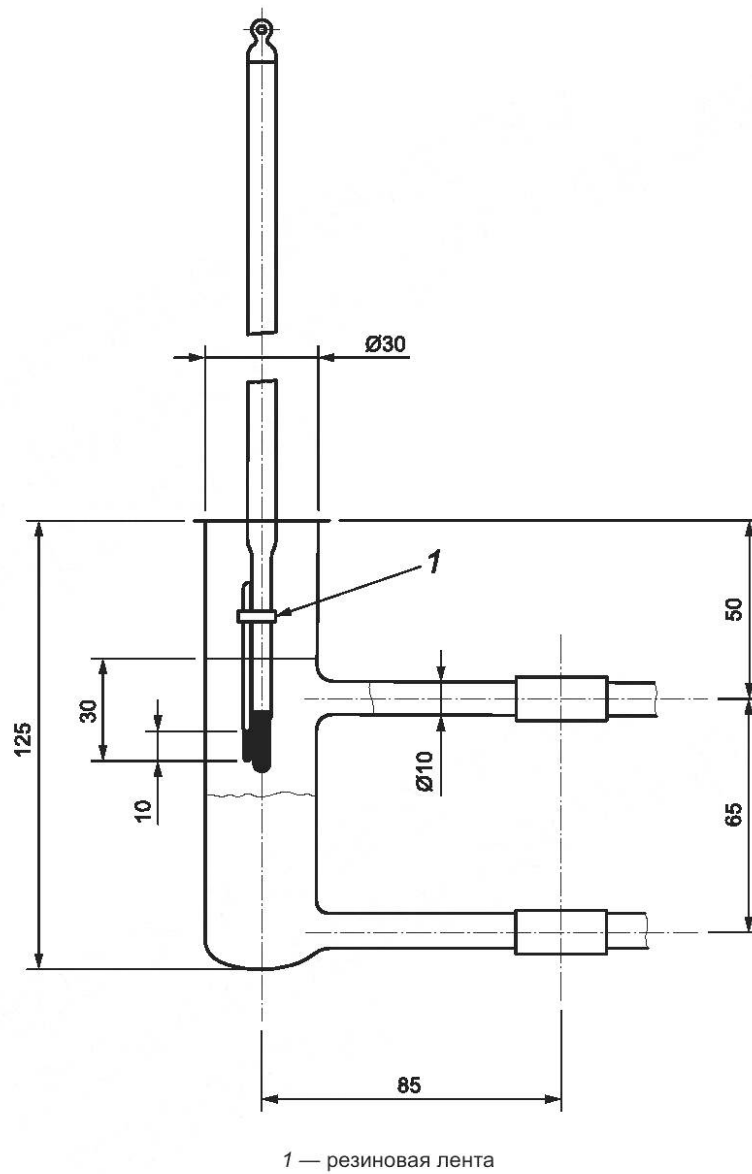
Рисунок 1 — Водяная рубашка
