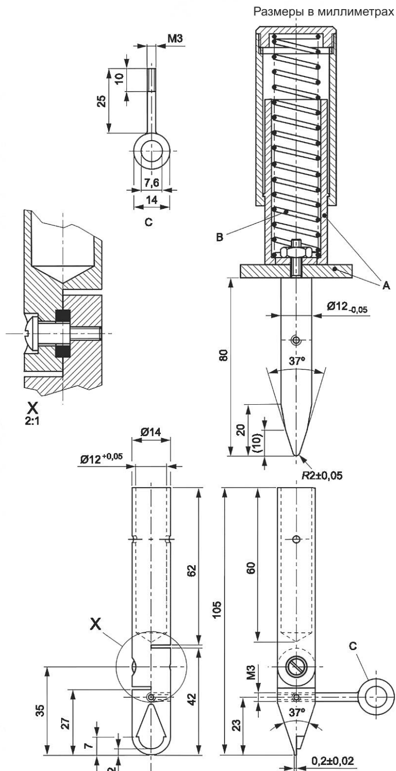
Рисунок 1 — Испытательный палец
