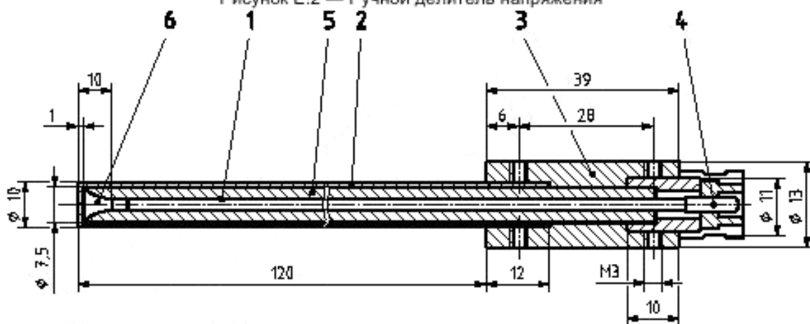
Рисунок Е.2 — Ручной делитель напряжения
