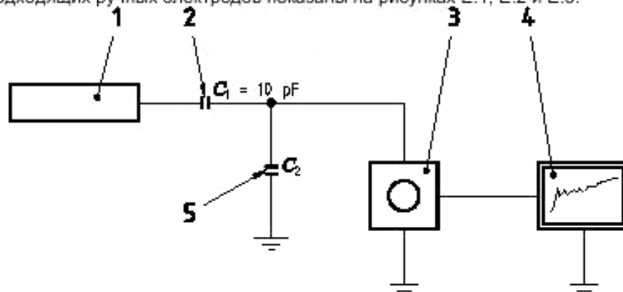
Рисунок Е.1 — Представление системы в целом
