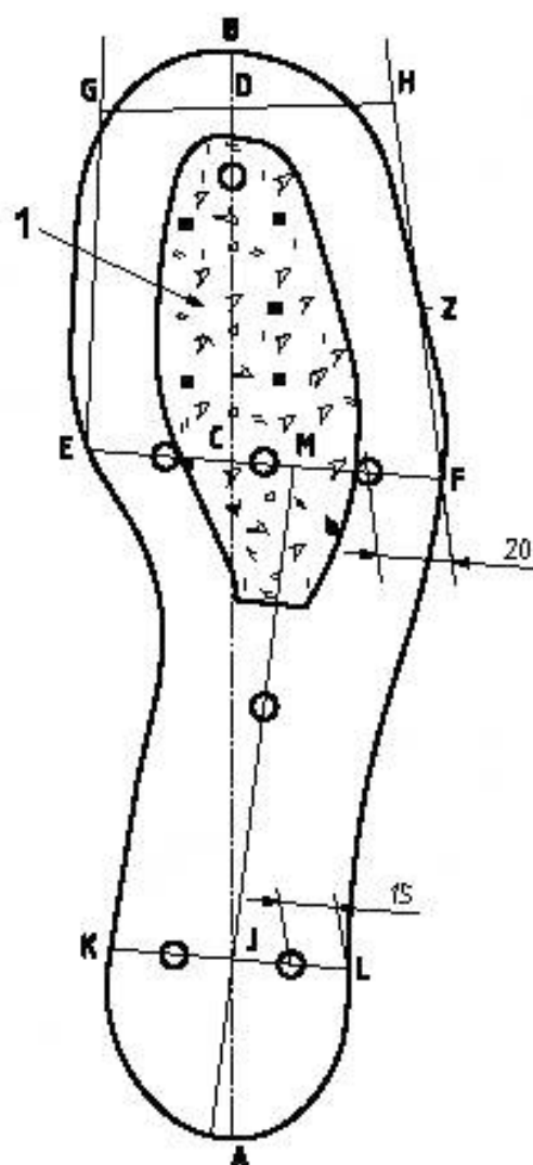
О – позиция потайных заклепок; 1 – нержавеющая сталь Рисунок А.1 — Рисунок несъемной стельки
