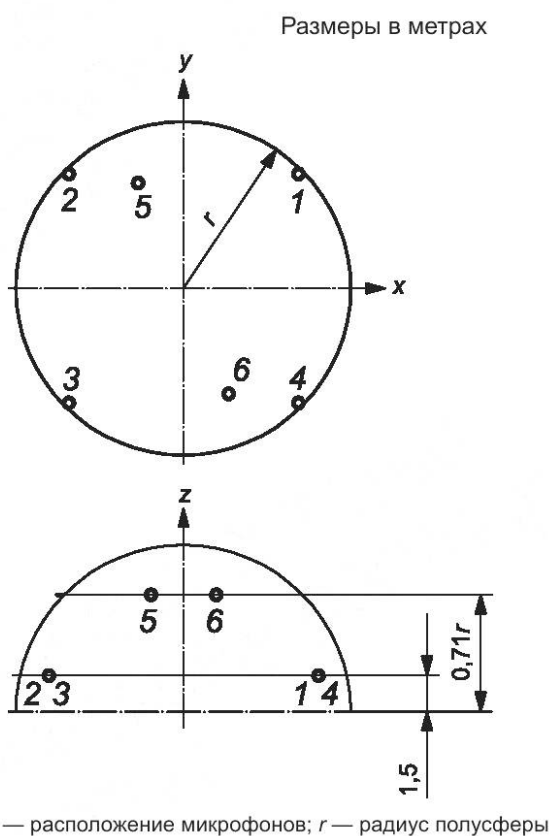
Рисунок 1 — Установка микрофонов на полусфере
