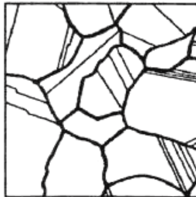
— Границы зерен
