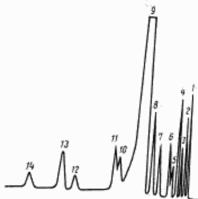
Типовая хроматограмма образца хлорбензола
