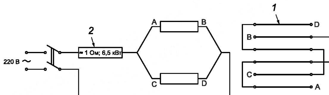
1 — стержень из карбида кремния; 2 — добавочное сопротивление
