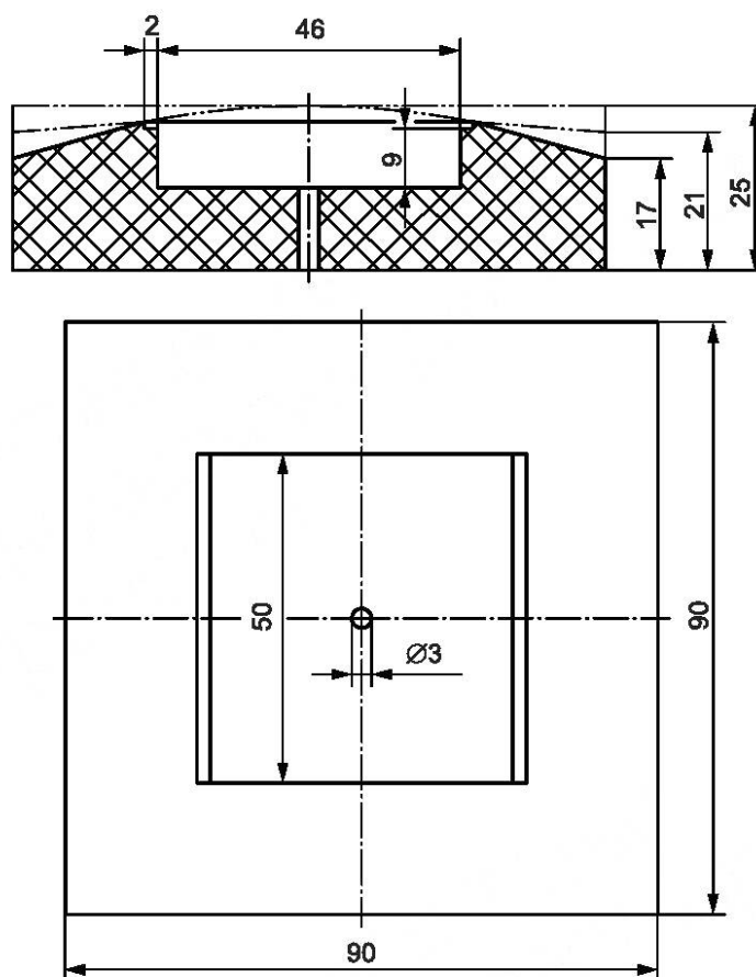
Рисунок 3 — Монтажный блок калориметра
