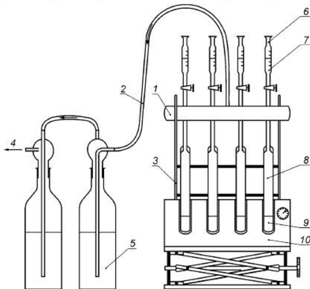
1 — вытяжной коллак; 2 — линия вытяжки для кислотных паров; 3 — опорная стойка; 4 — к отсасывающему насосу; 5 — раствор гидроксида натрия; 6 — капельная воронка; 7 — перекись водорода; 8 — трубка для разложения; 9 — образец в концентрированной серной кислоте; 10 — нагреватель сушильного блока
