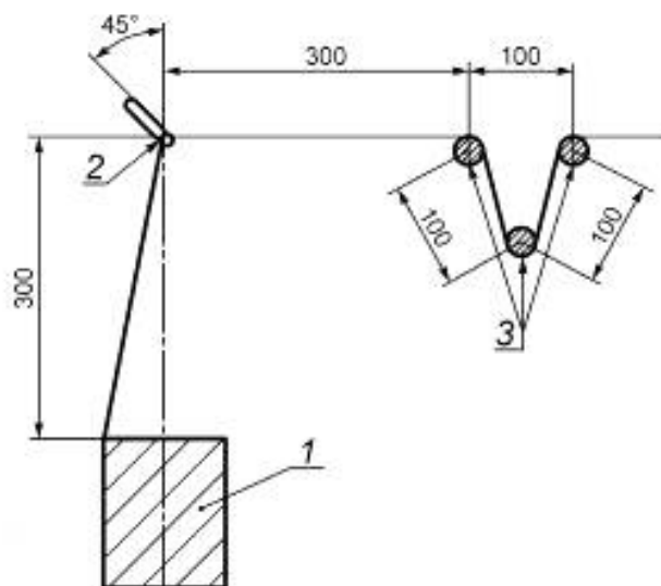
Рисунок 1 — Устройство для контролируемой разматки ролинга
