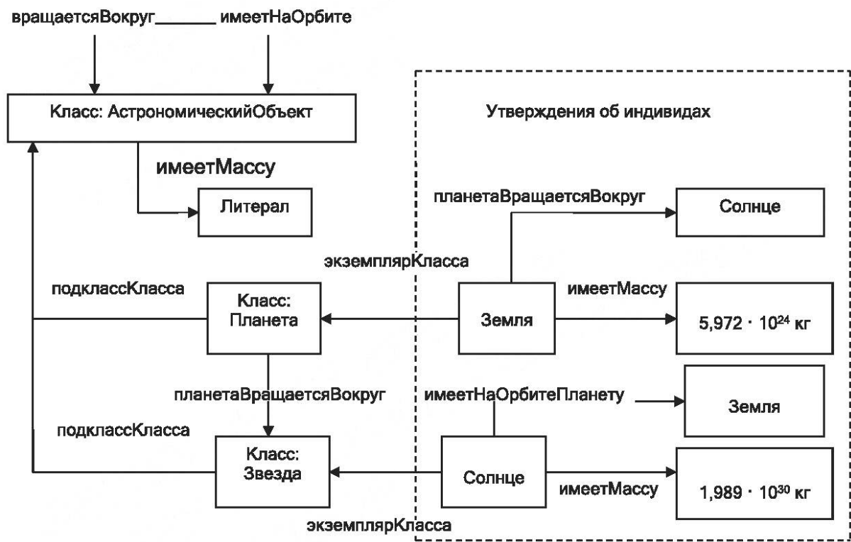
Рисунок 17 — Иллюстрация фрагмента онтологии и утверждений
