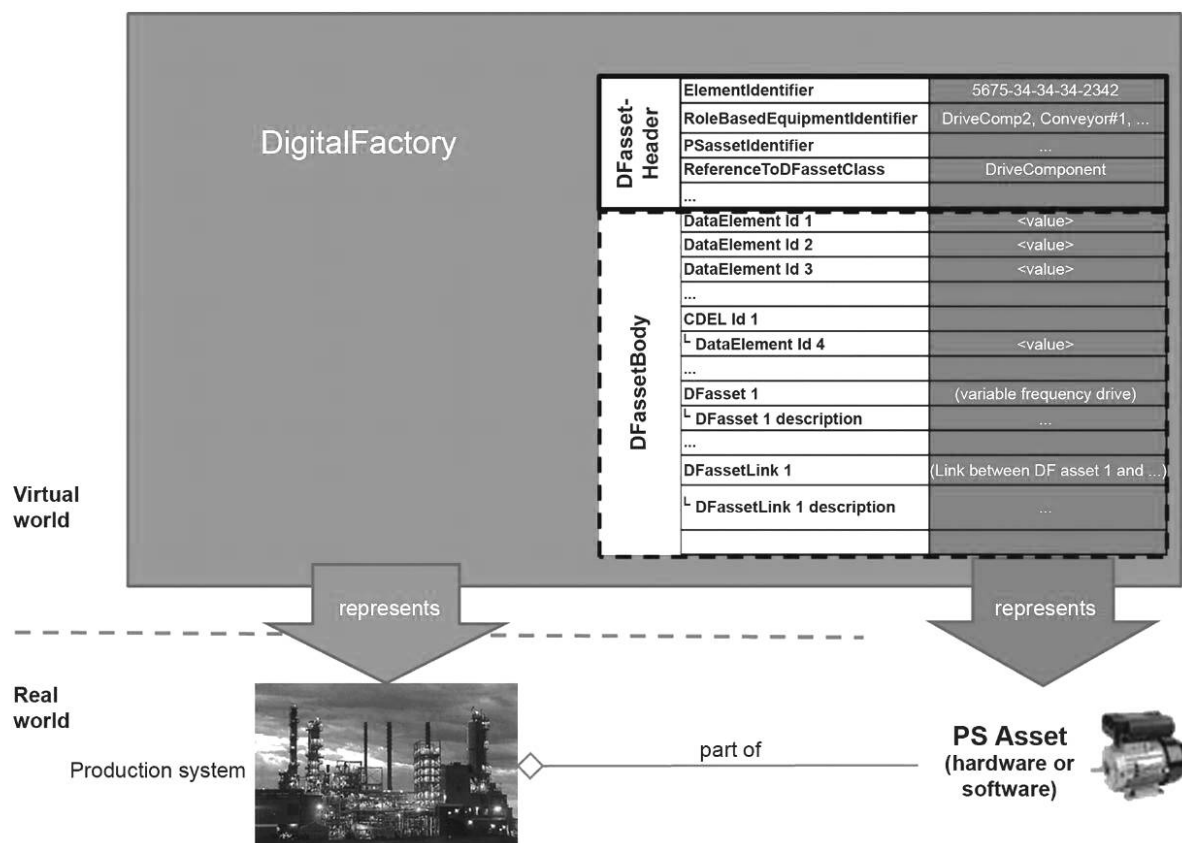
Рисунок 2 — Представление производственной системы
